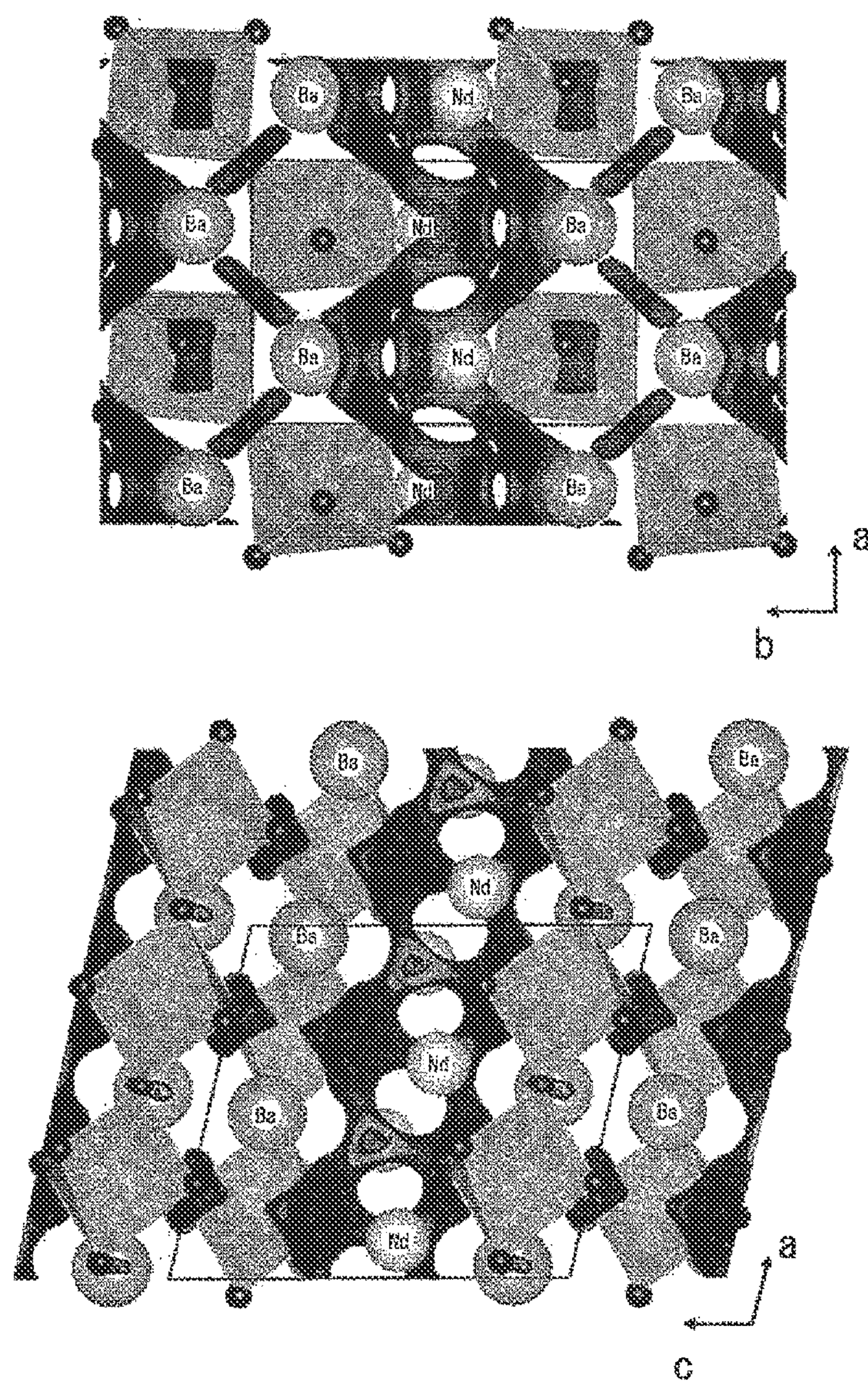
EXAMPLE 1-1 \text{NdBaInO}_4
