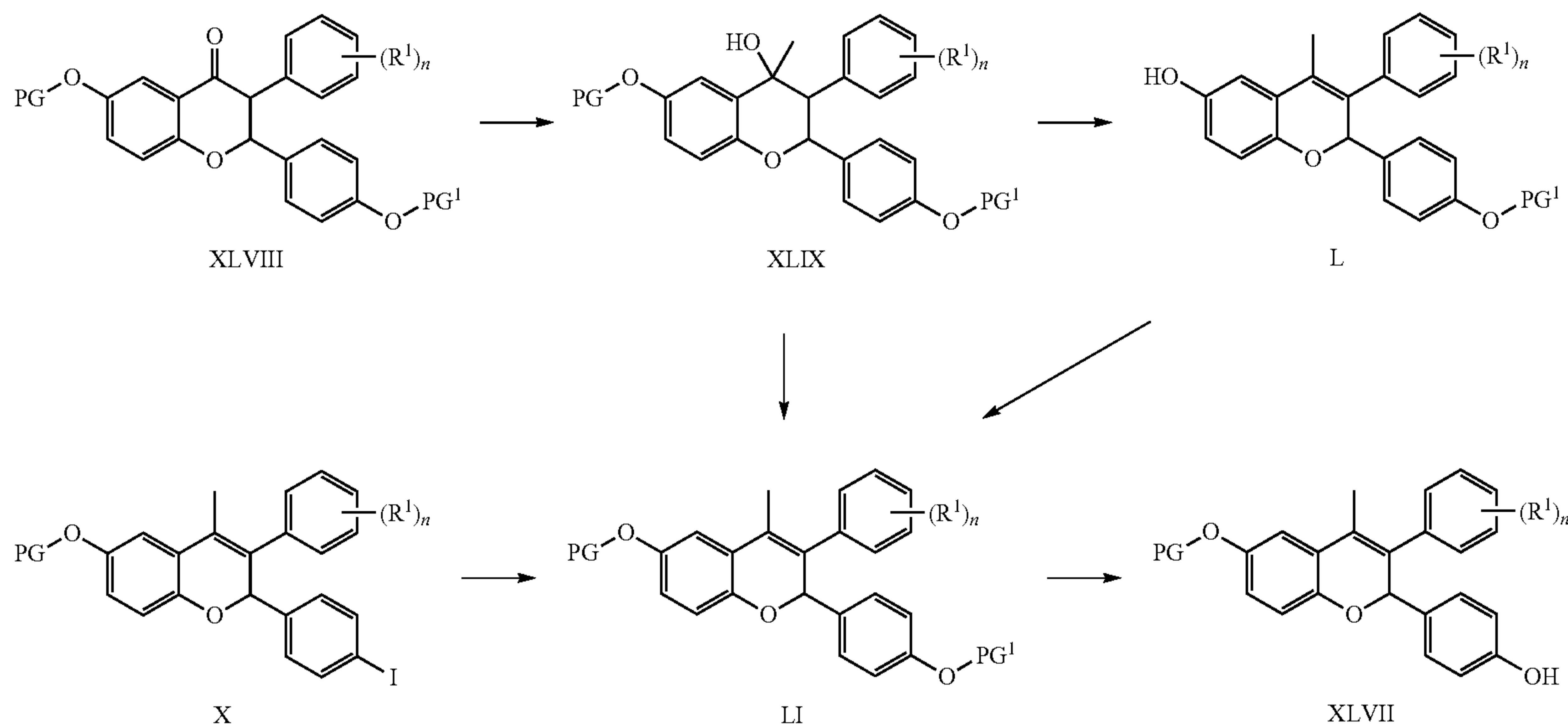
Scheme 14.
