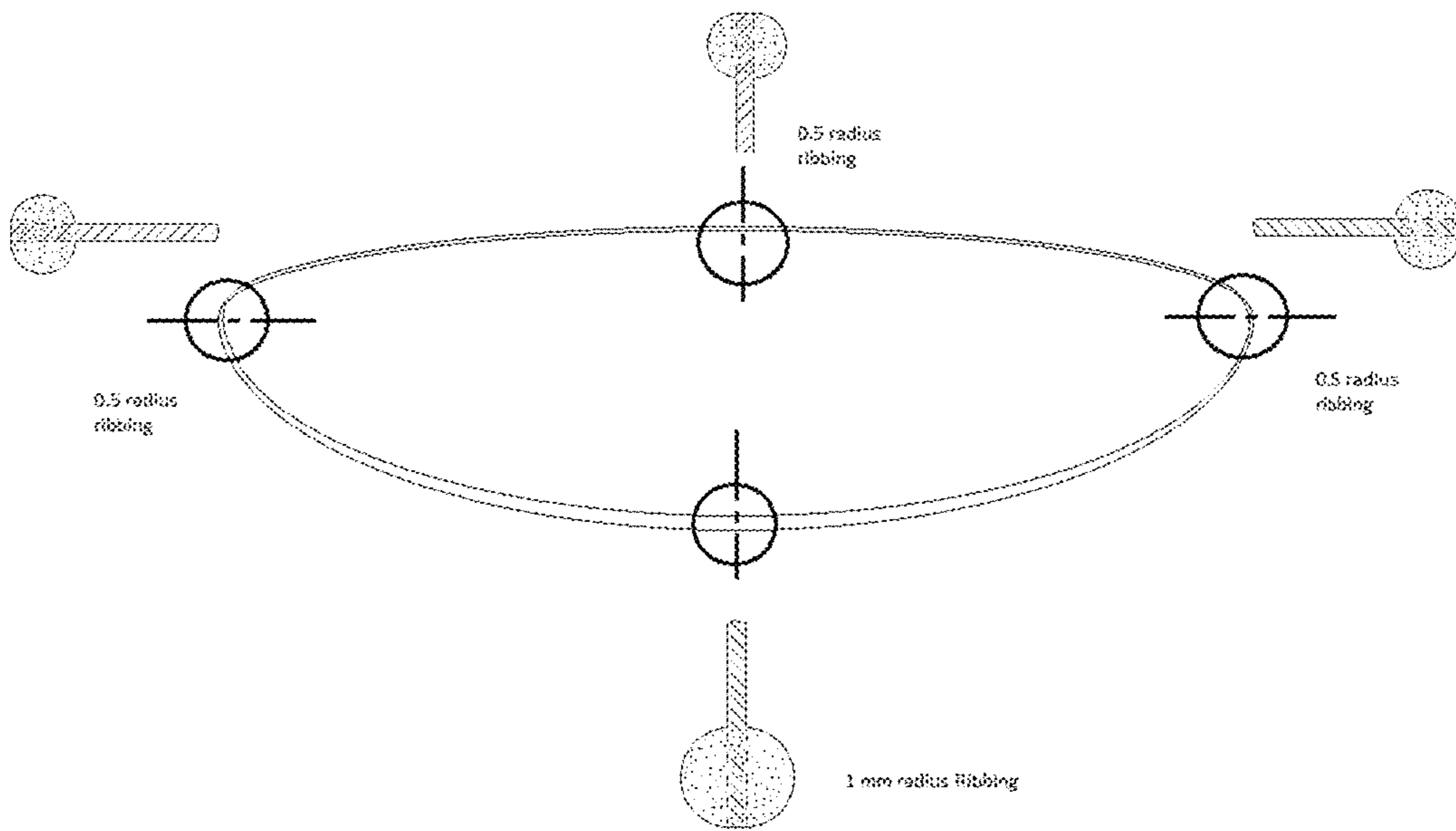
FIG. 13B
