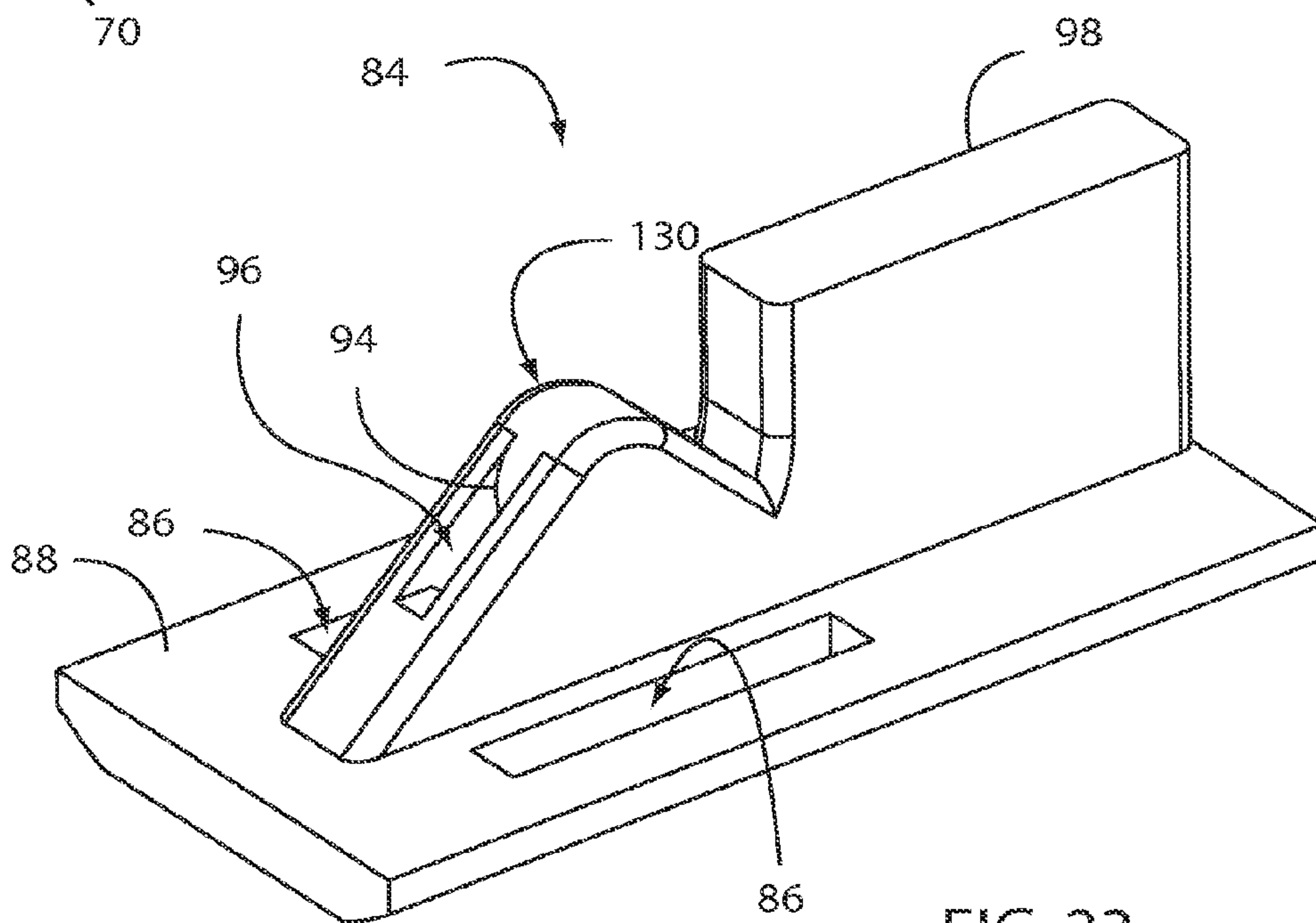
FIG. 22
