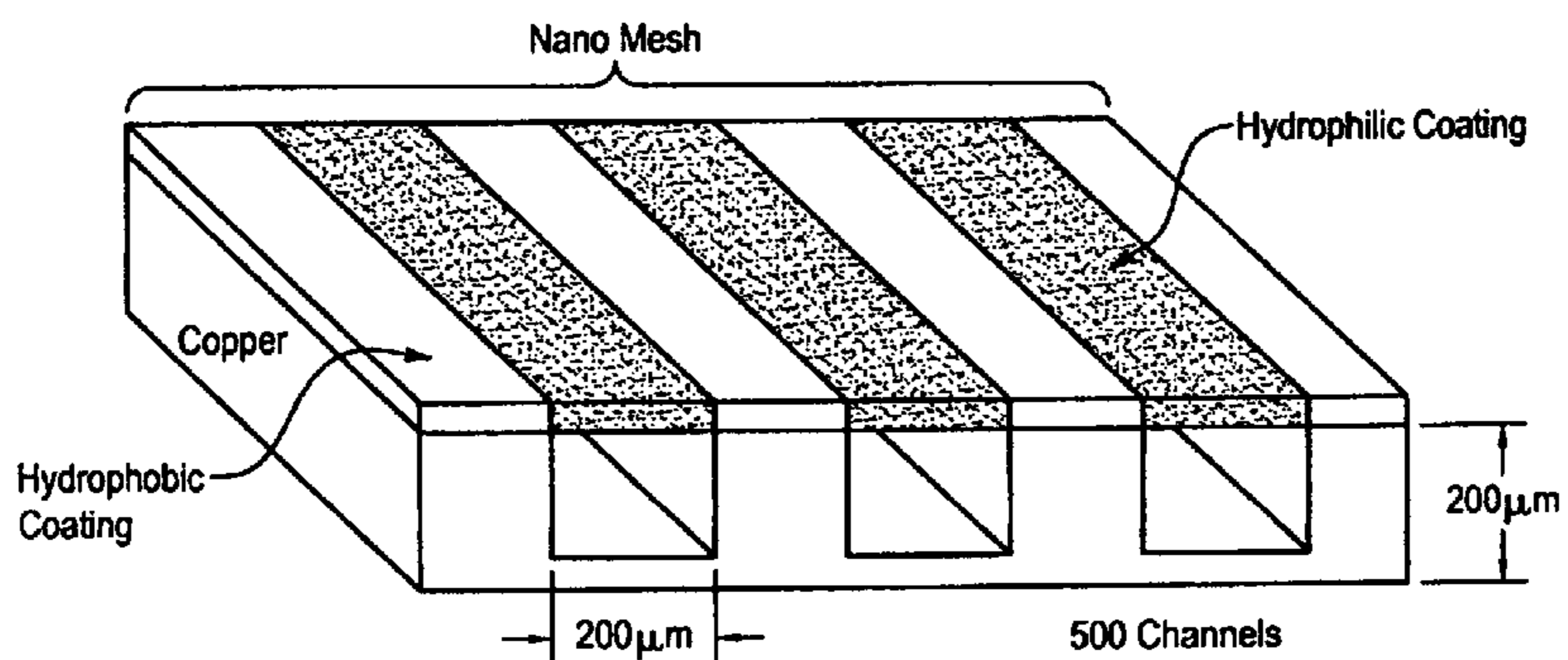
Condenser FIG. 20-b
