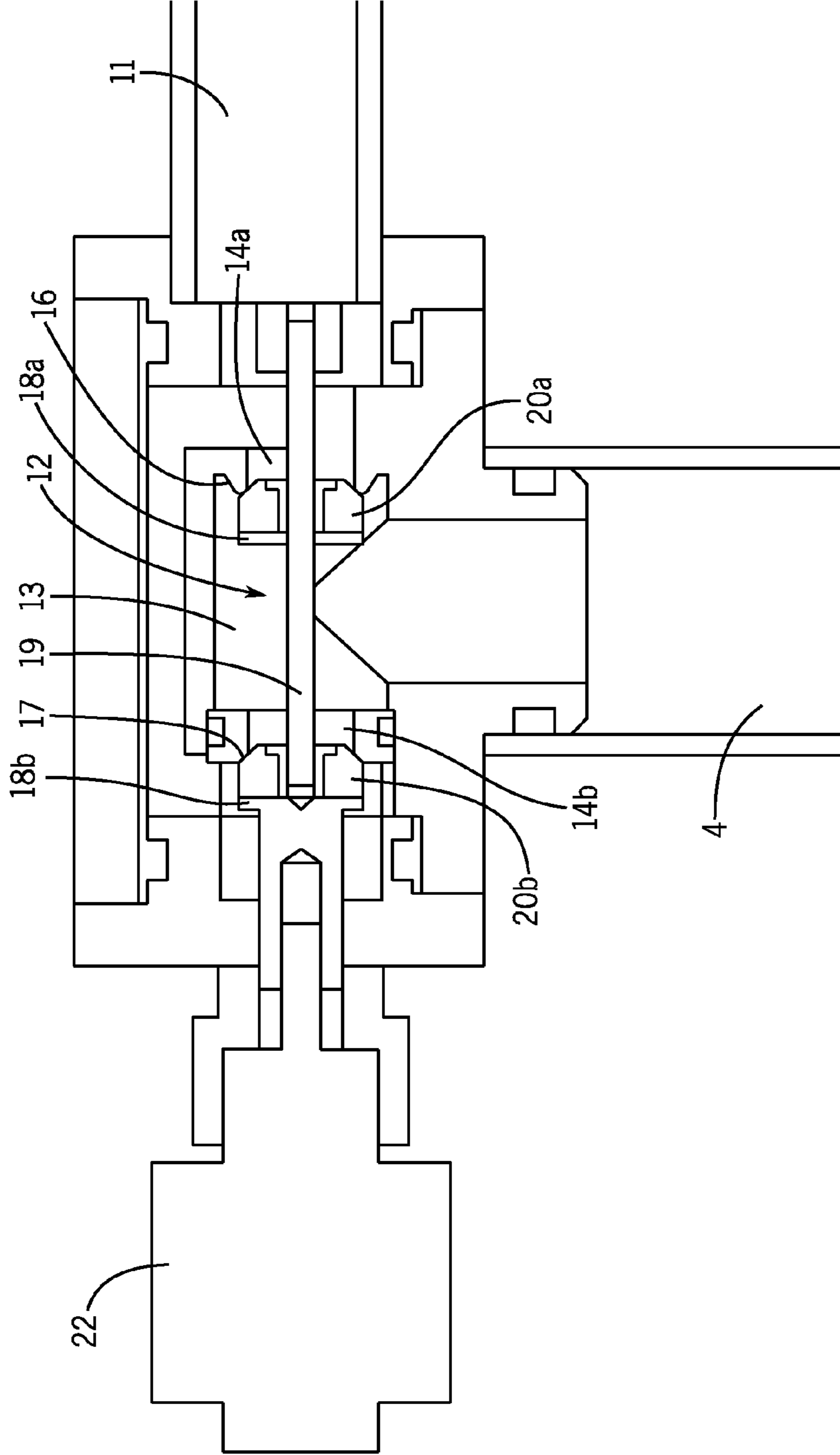
FIG. 11C
