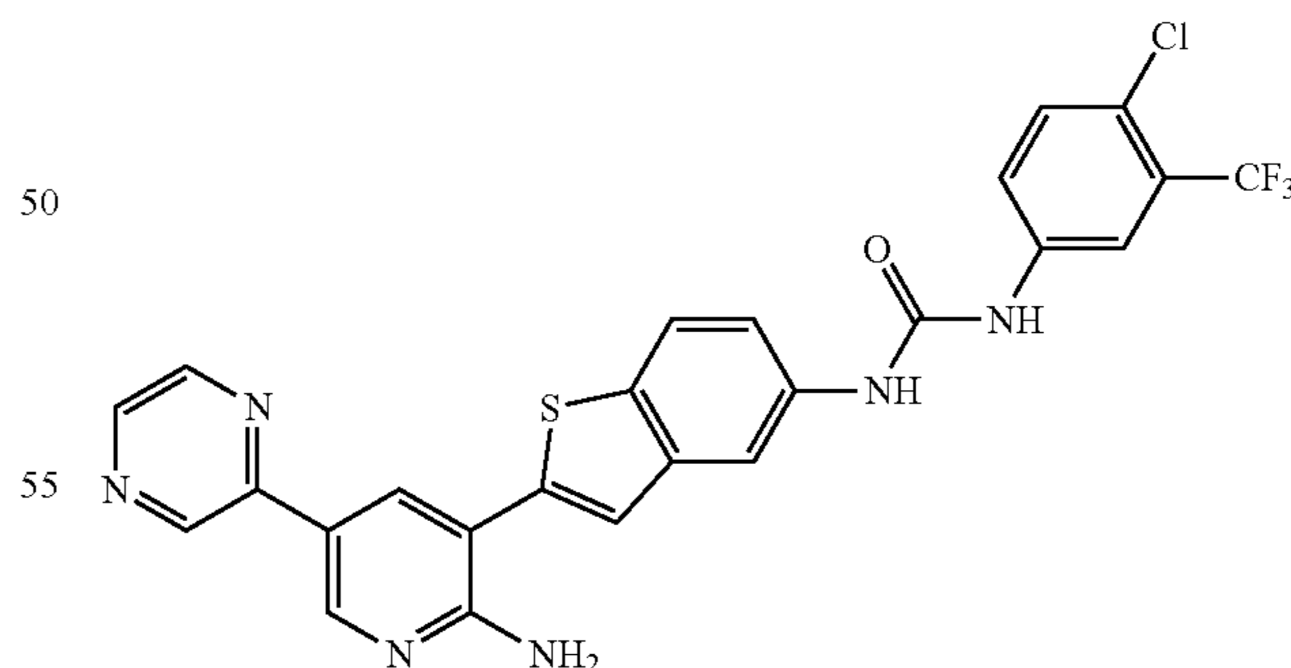
1-[2-(2-amino-5-pyrazin-2-ylpyridin-3-yl)-1-benzothien-5-yl]-3-[4-chloro-3-(trifluoromethyl)phenyl]urea
