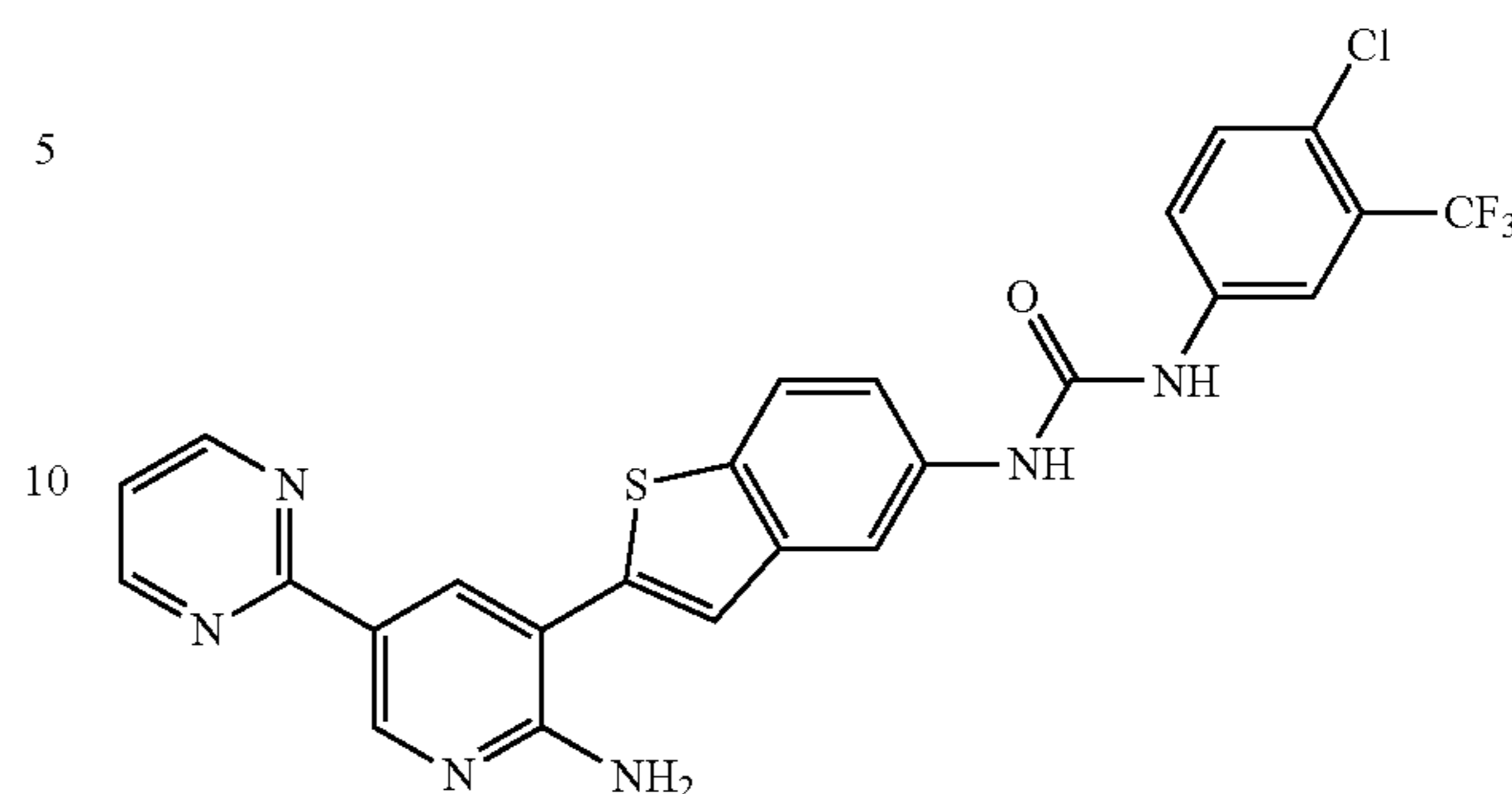
1-[2-(2-amino-5-pyrimidin-2-ylpyridin-3-yl)-1-benzothien-5-yl]-3-[4-chloro-3-(trifluoromethyl)phenyl]urea
