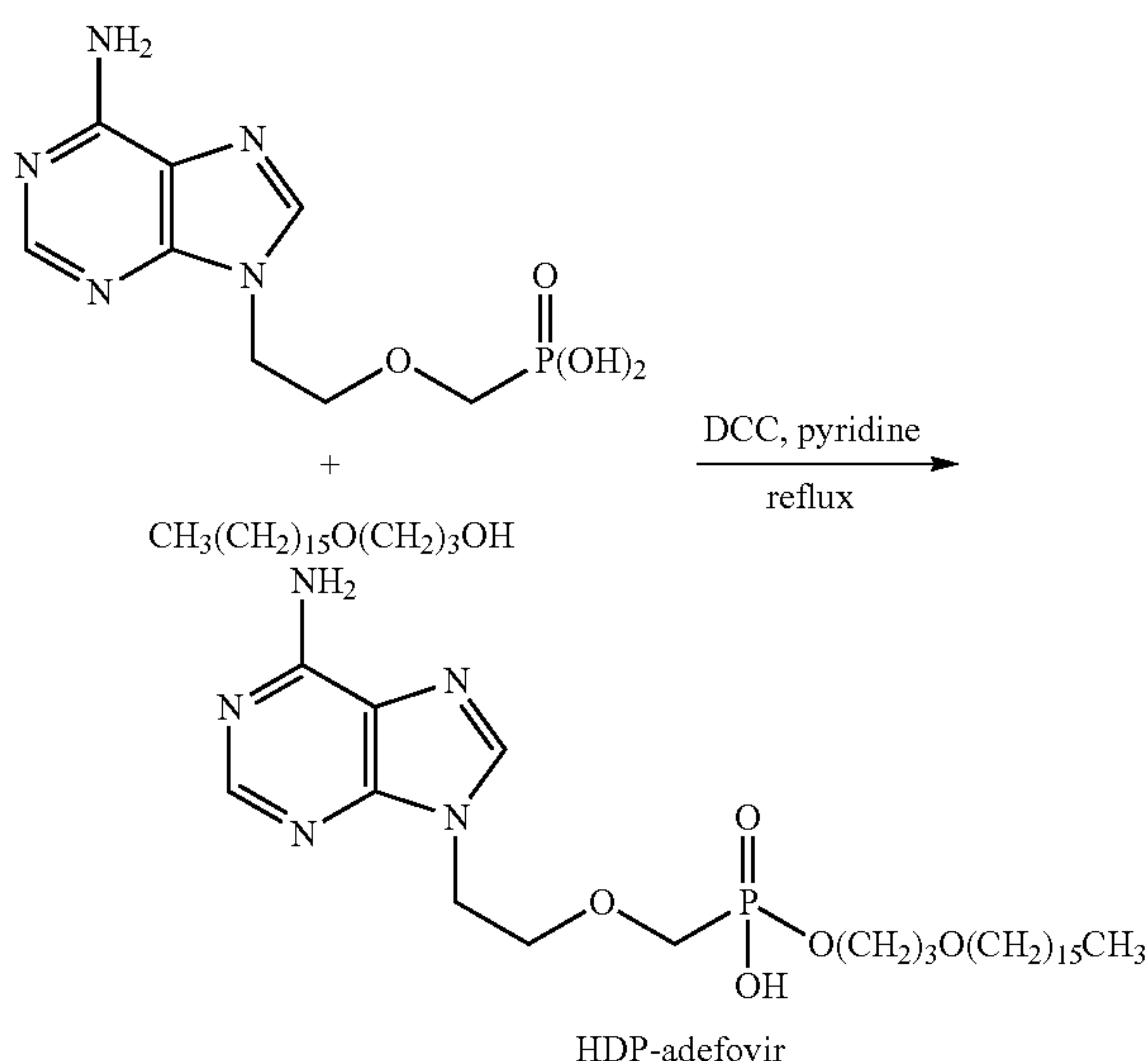
Scheme VI
