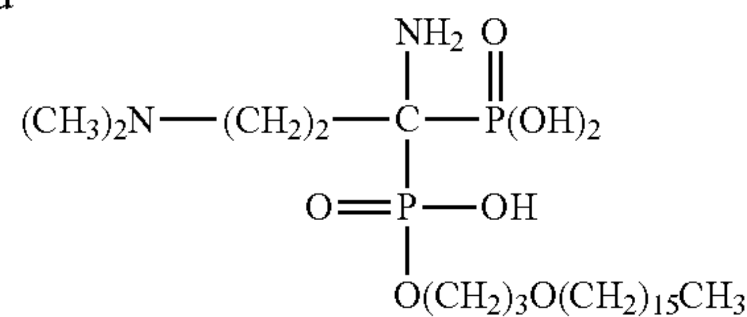
HDP-amino-olpadronate
