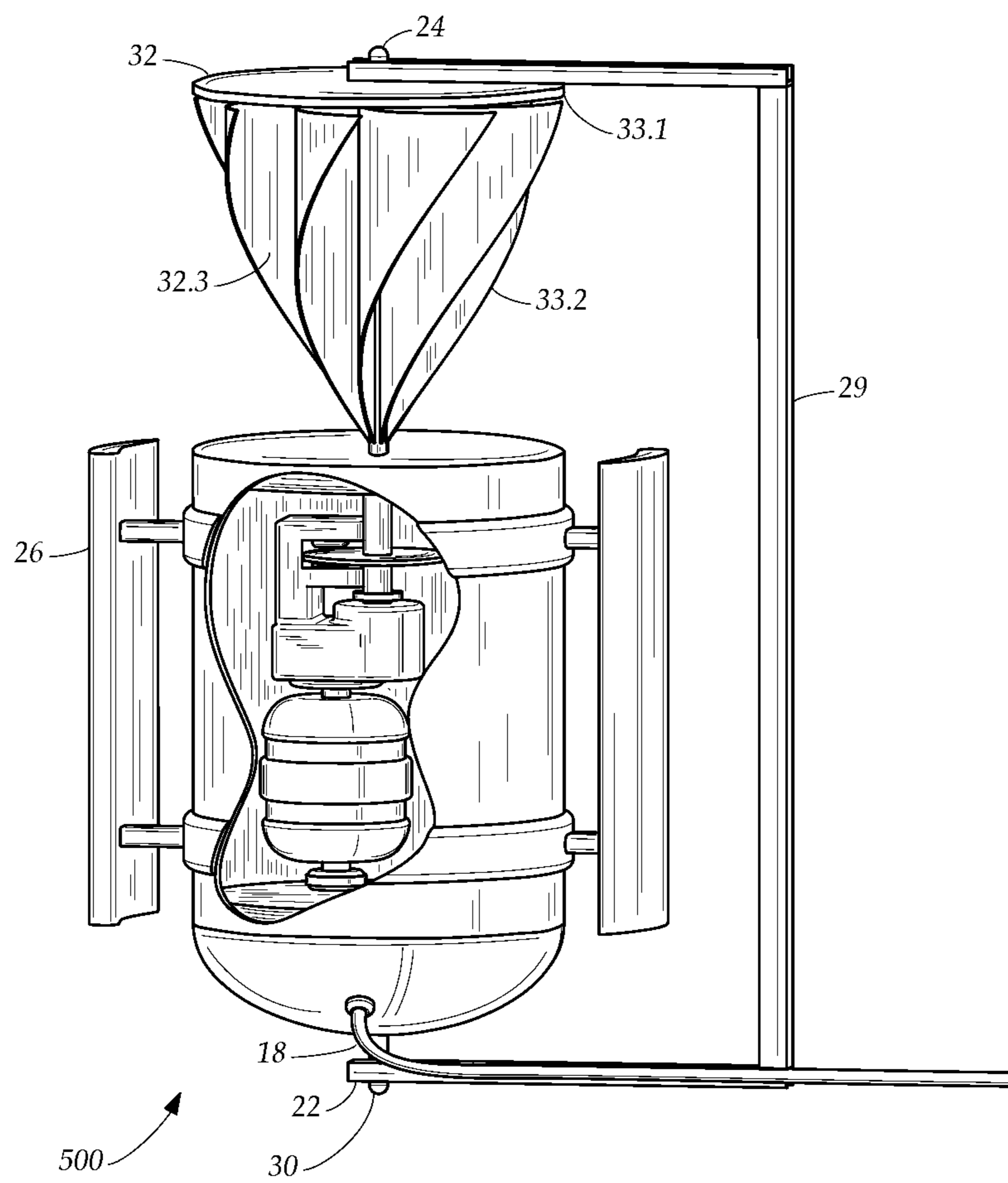
FIG. 8
