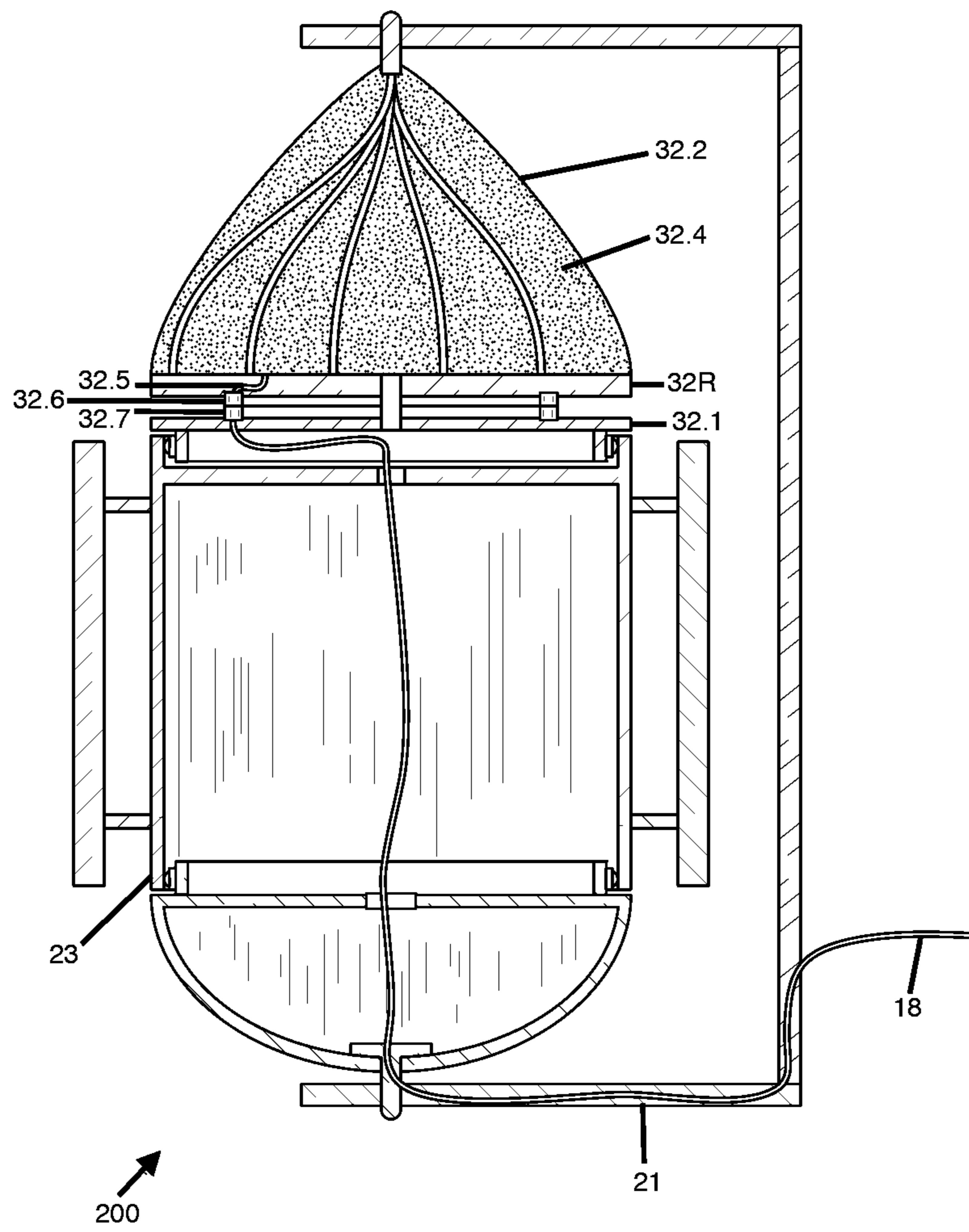
FIG. 17B
