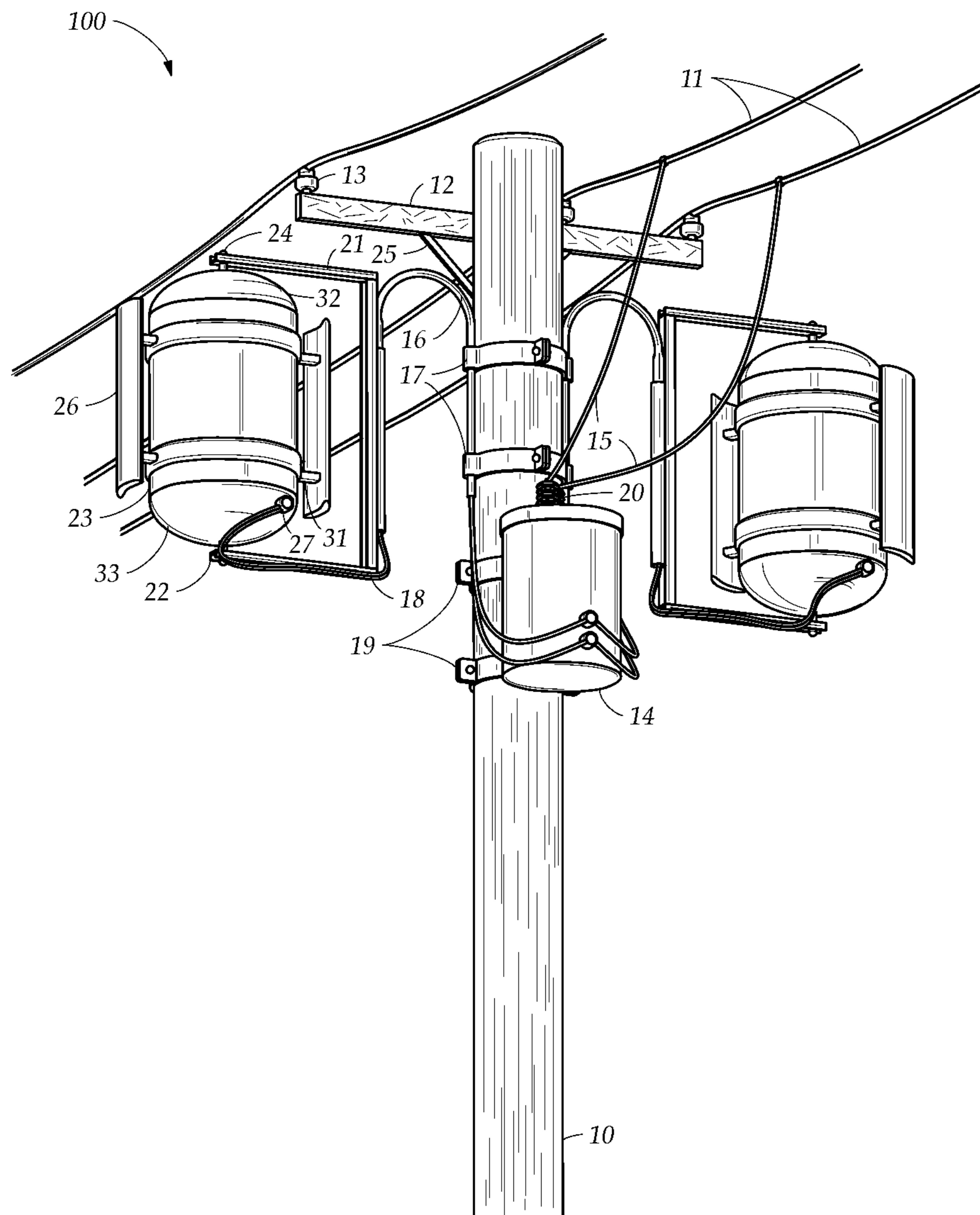
FIG. 1B
