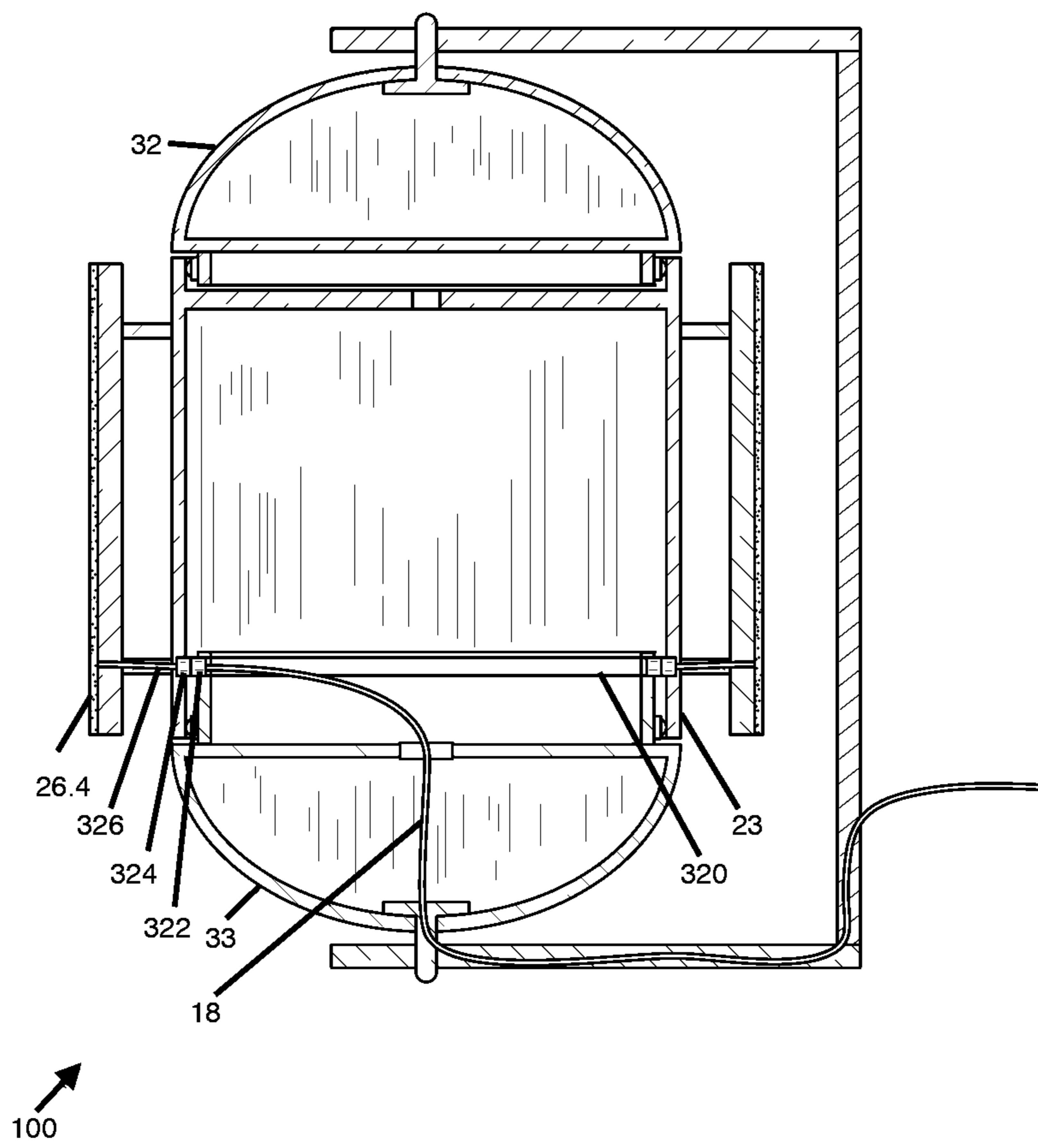
FIG. 17A
