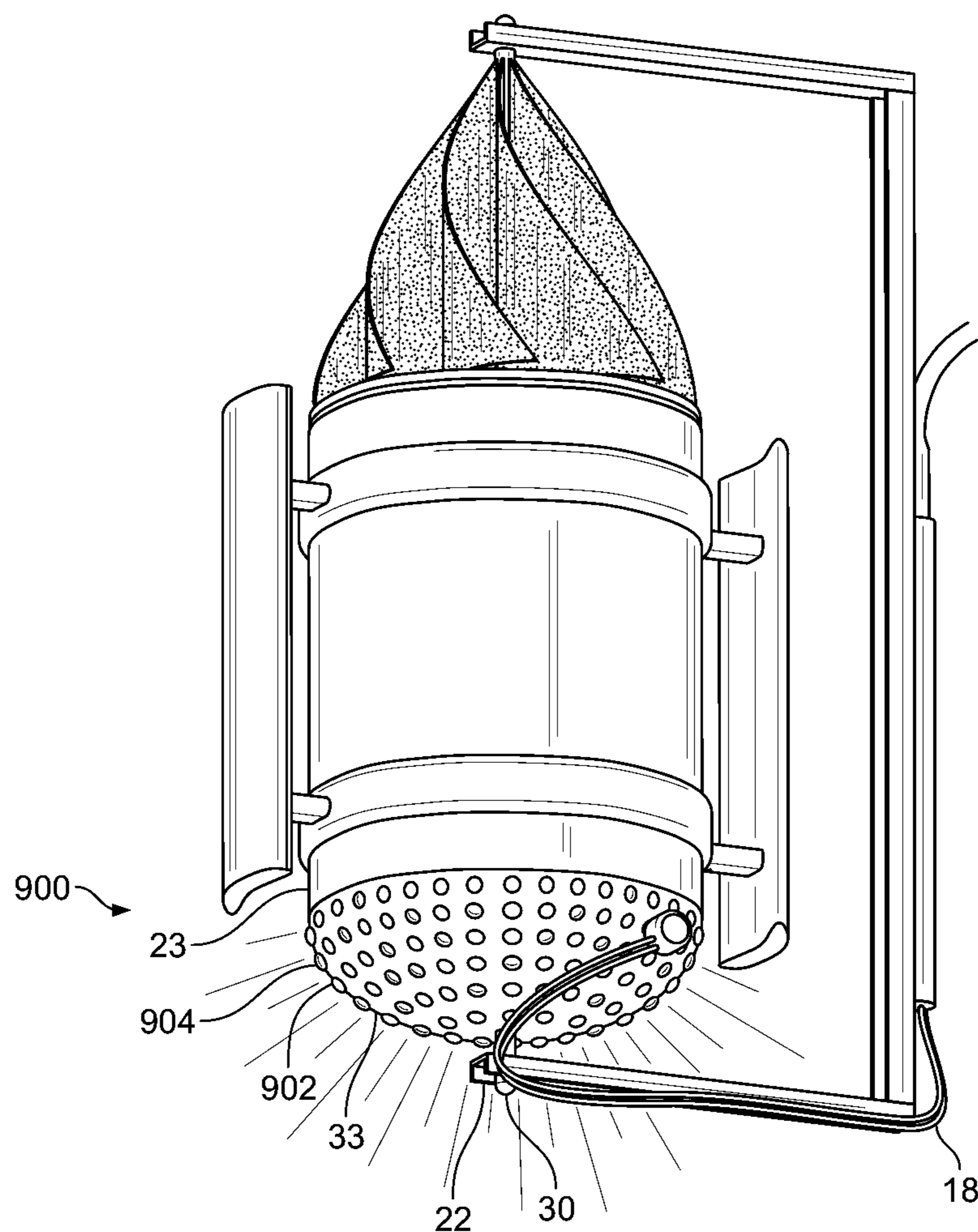
FIG. 19
