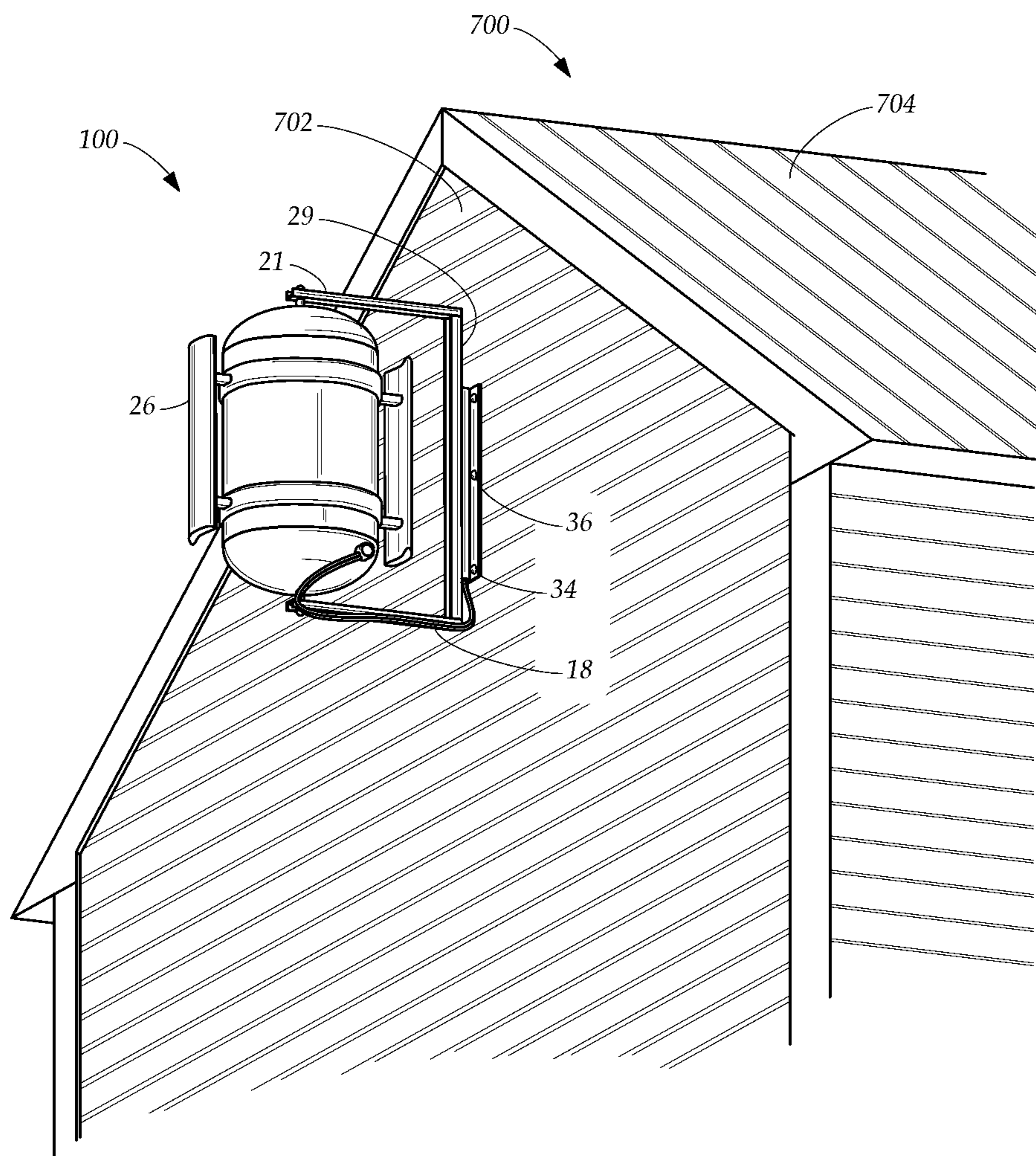
FIG. 11
