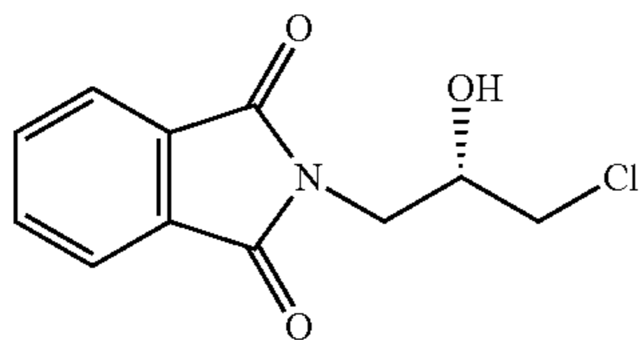
(S)-1-Chloro-3-phthalimido-2-propanol
