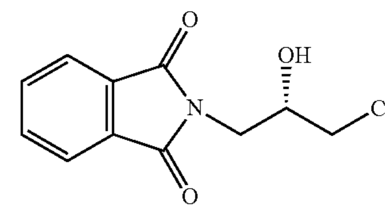
(S)-1-Chloro-3-phthalimido-2-propanol
