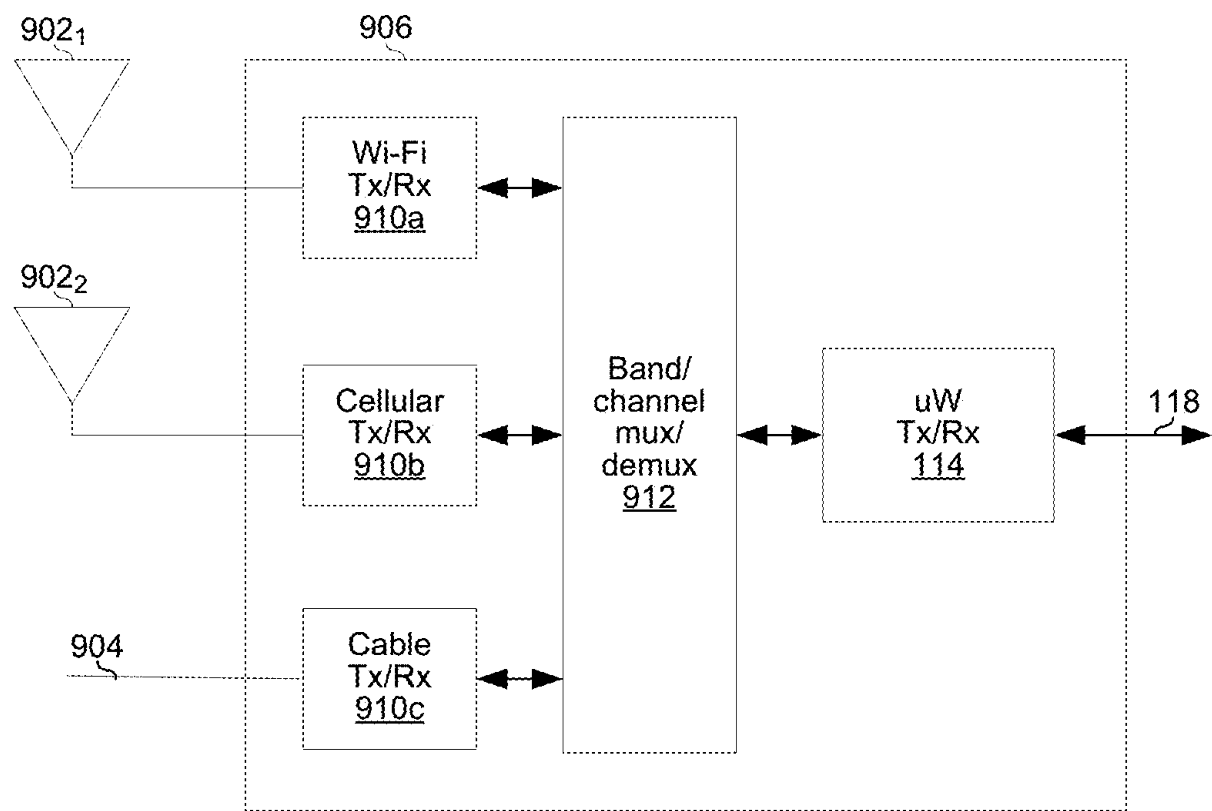
FIG. 9B
