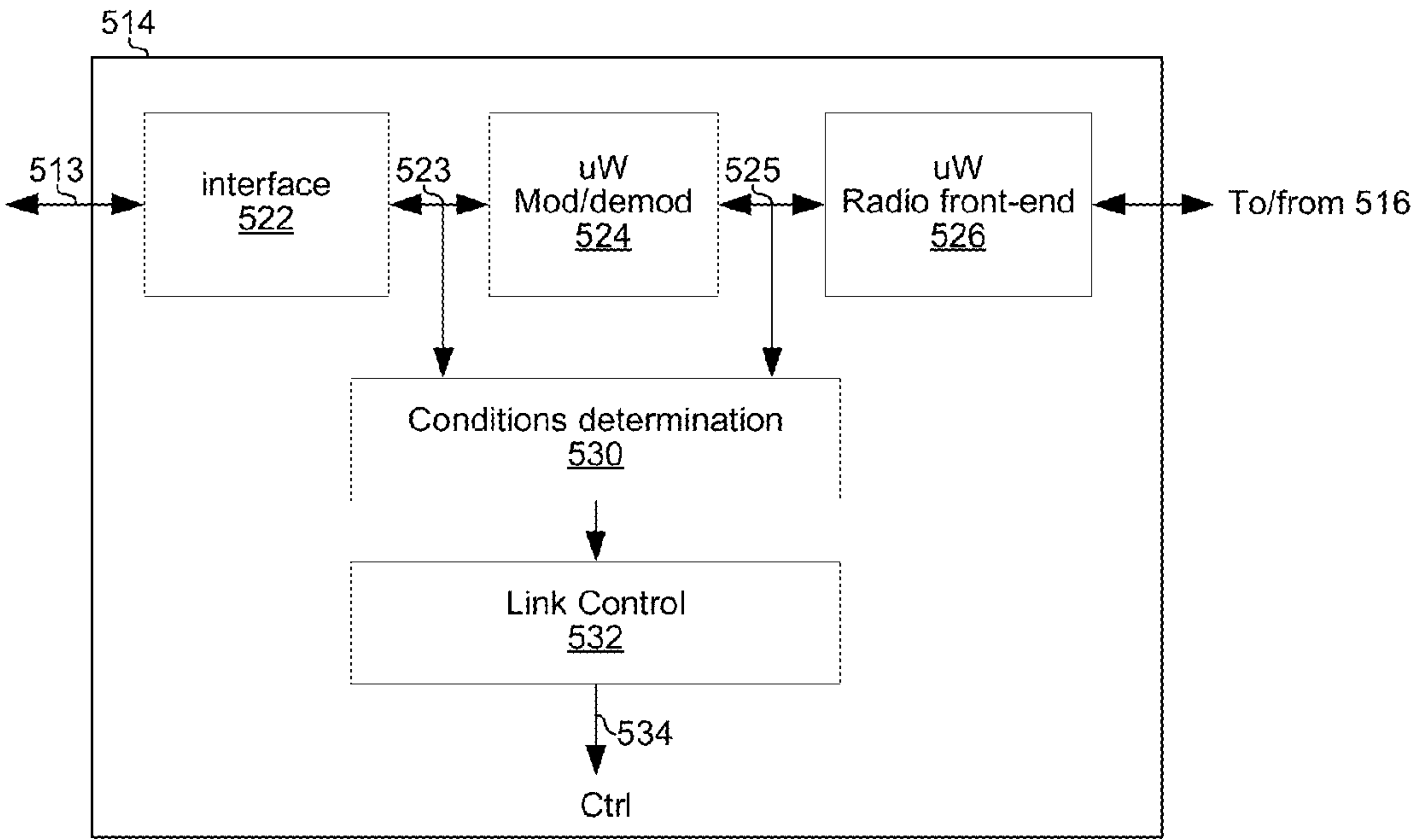
FIG. 5C
