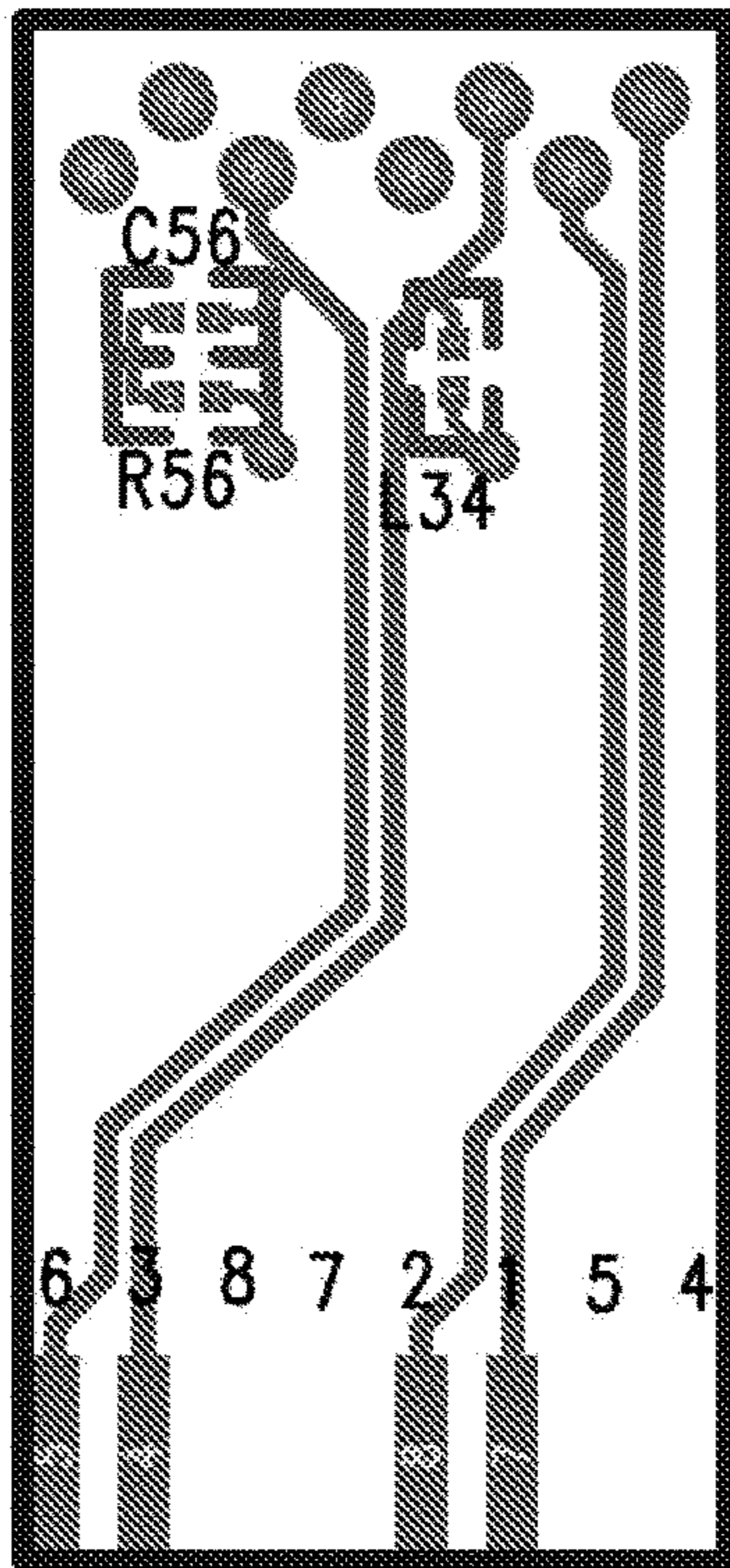
PCB Top Layer
