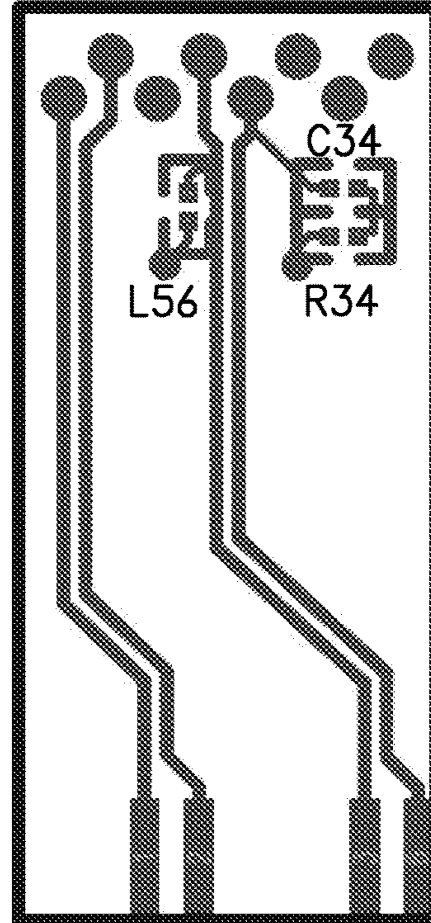
PCB Bottom Layer
