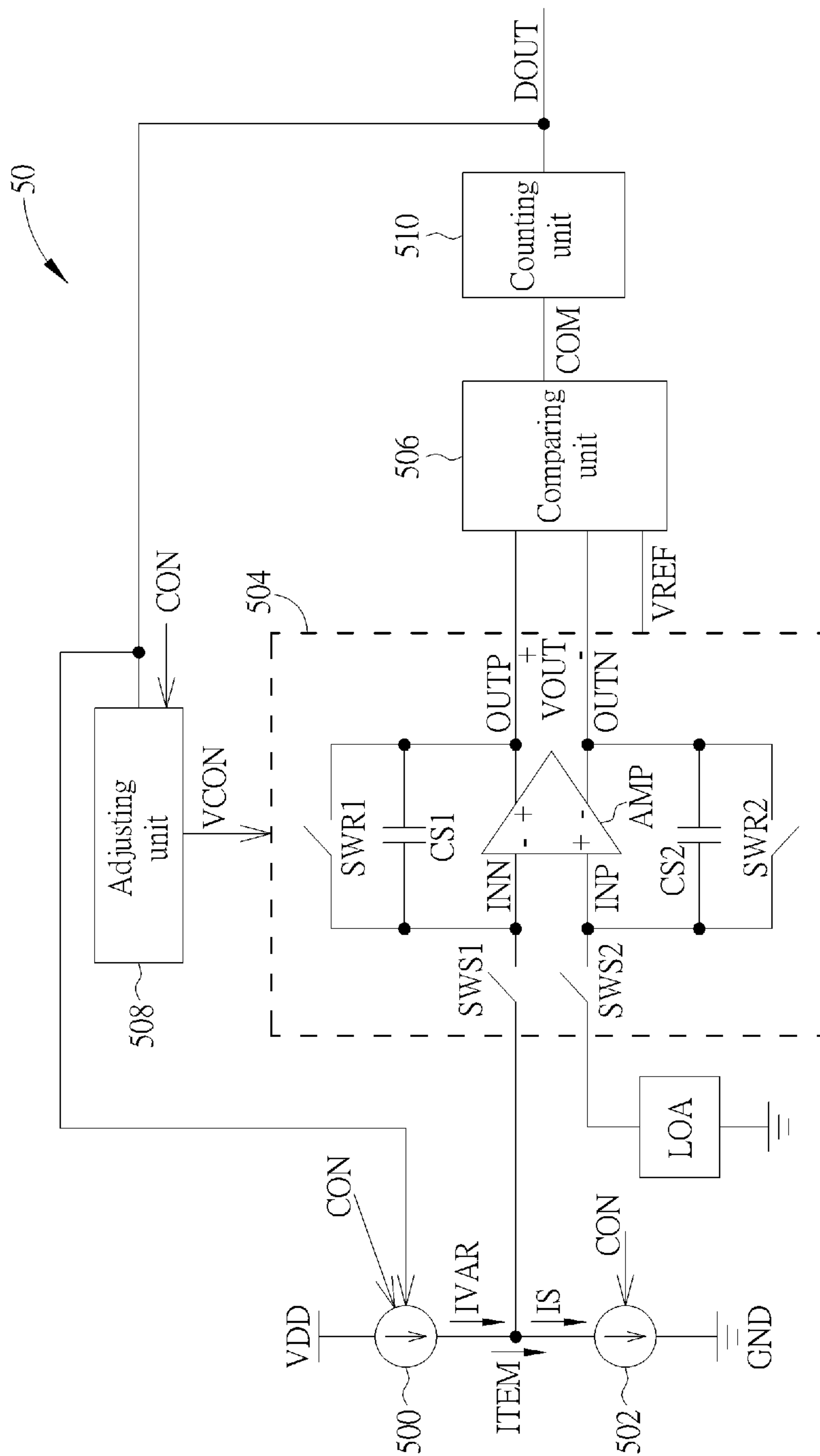
FIG. 5
