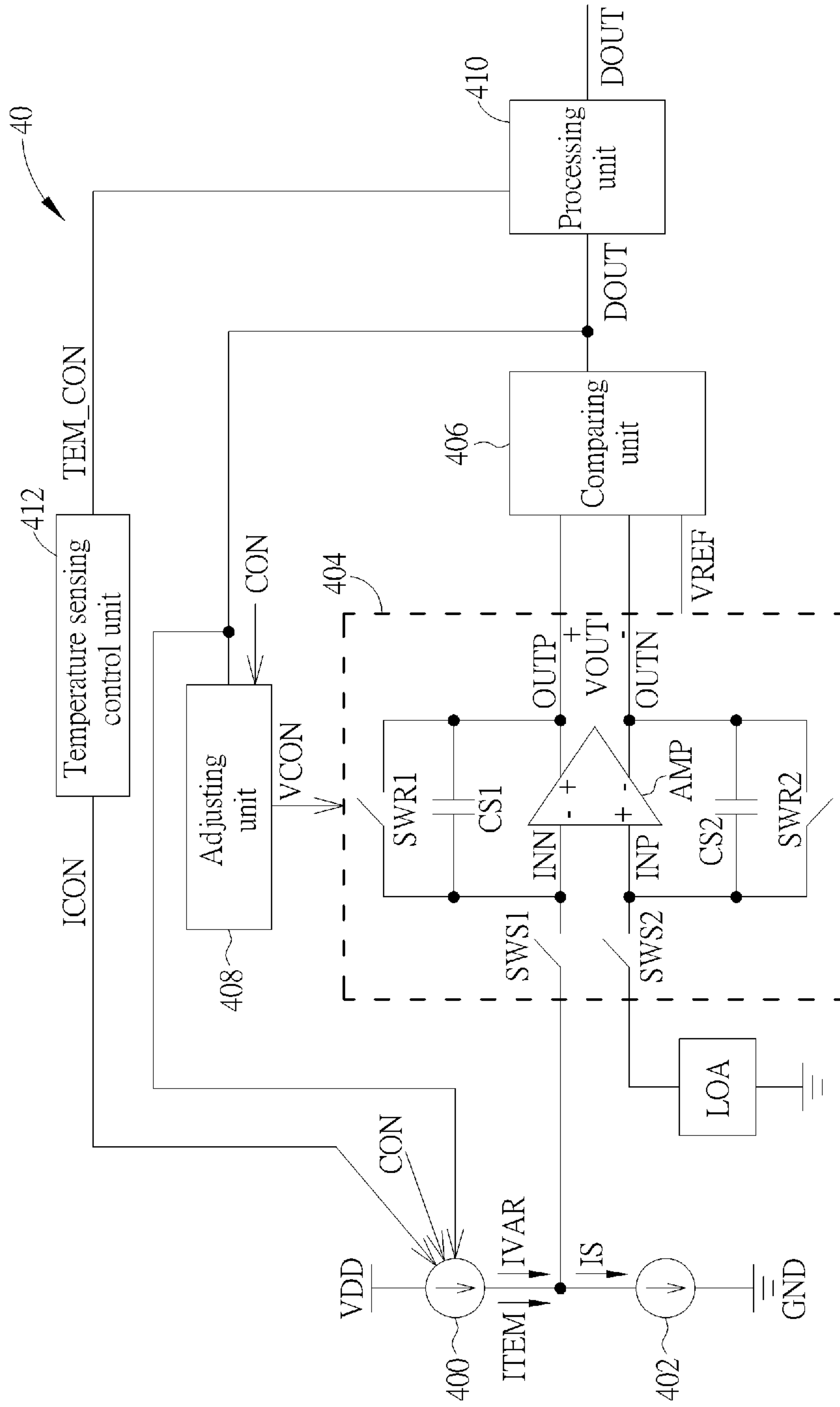
FIG. 4
