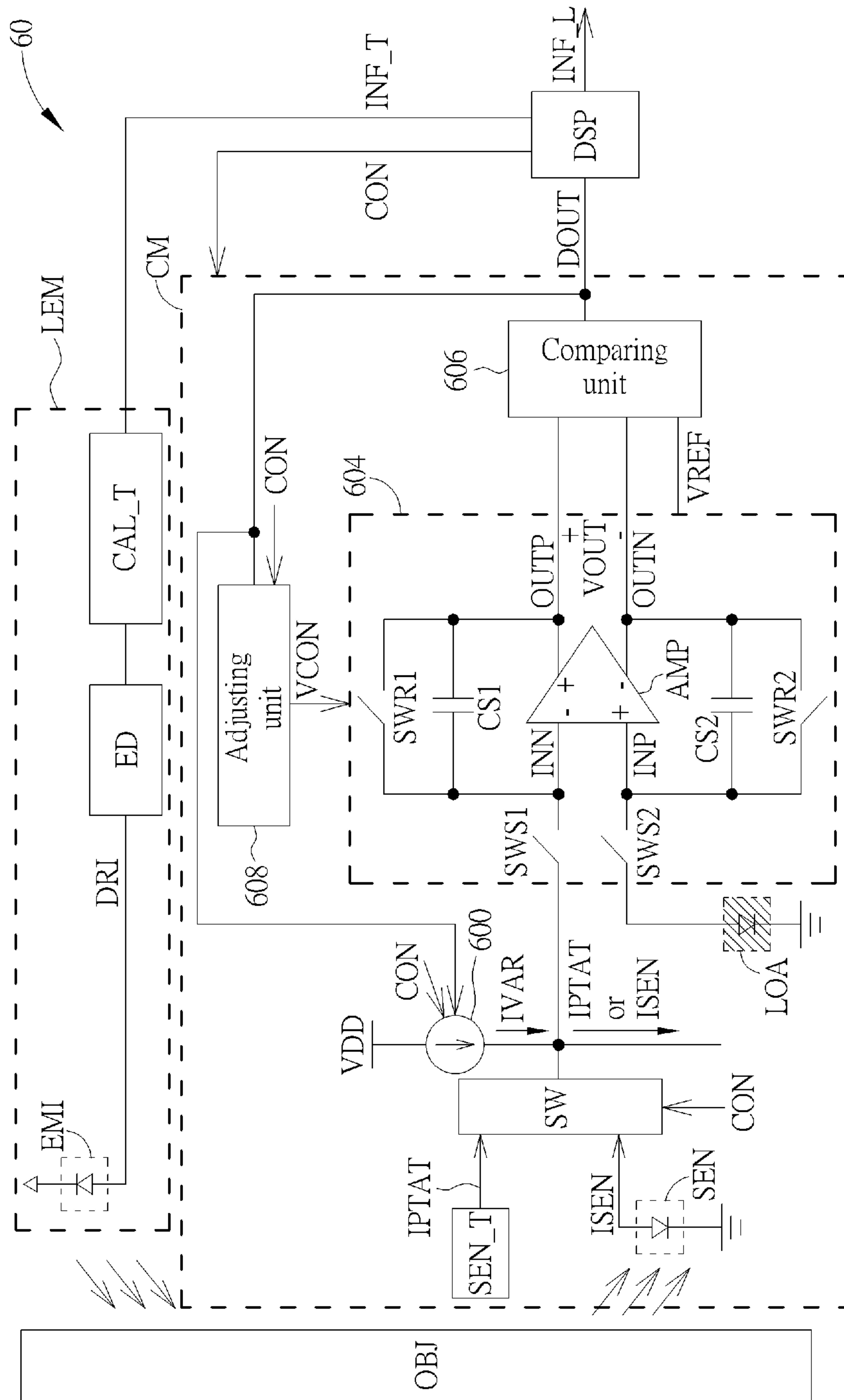
FIG. 6
