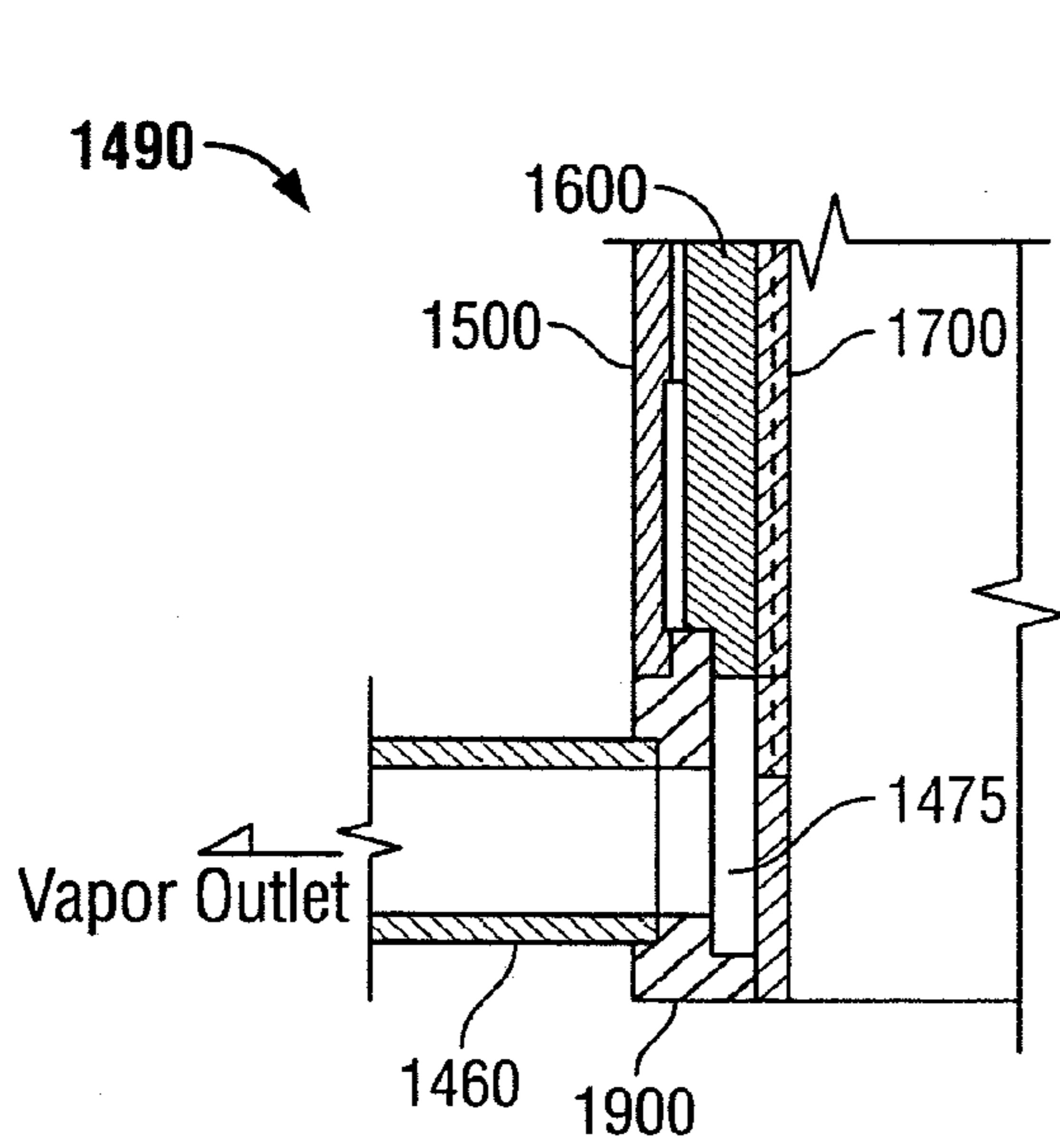
FIG. 14E
