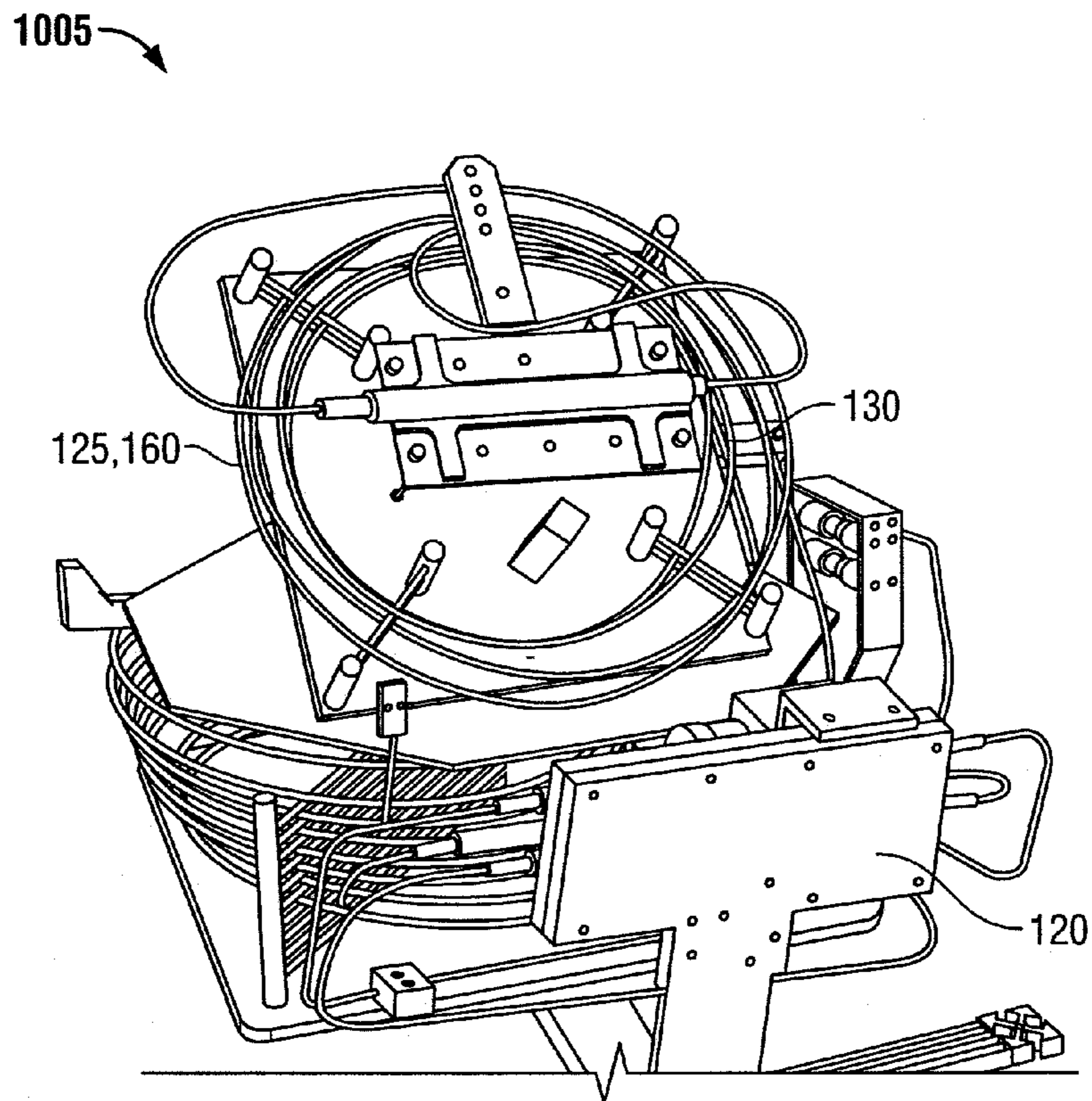
FIG. 9B
