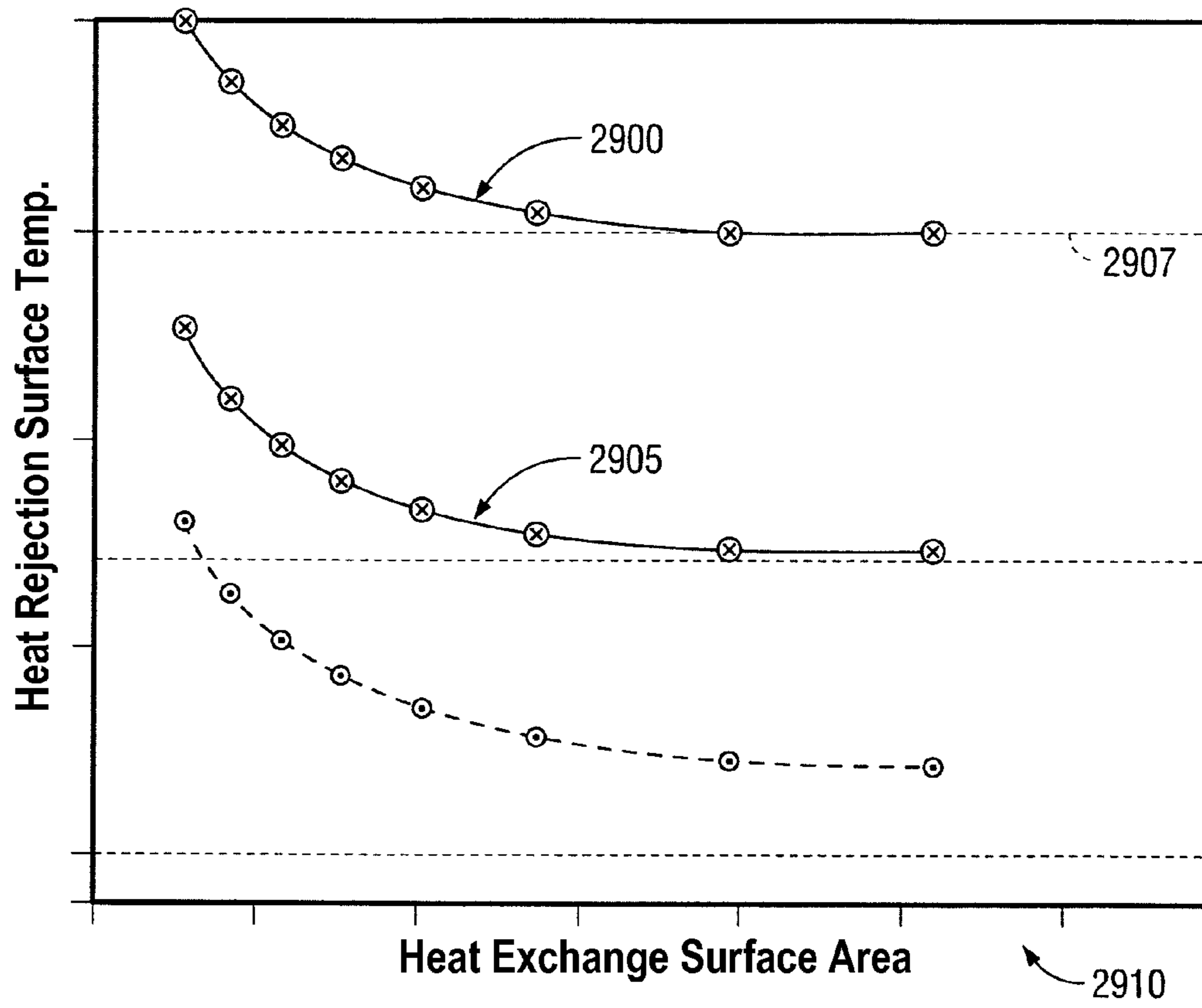
FIG. 29
