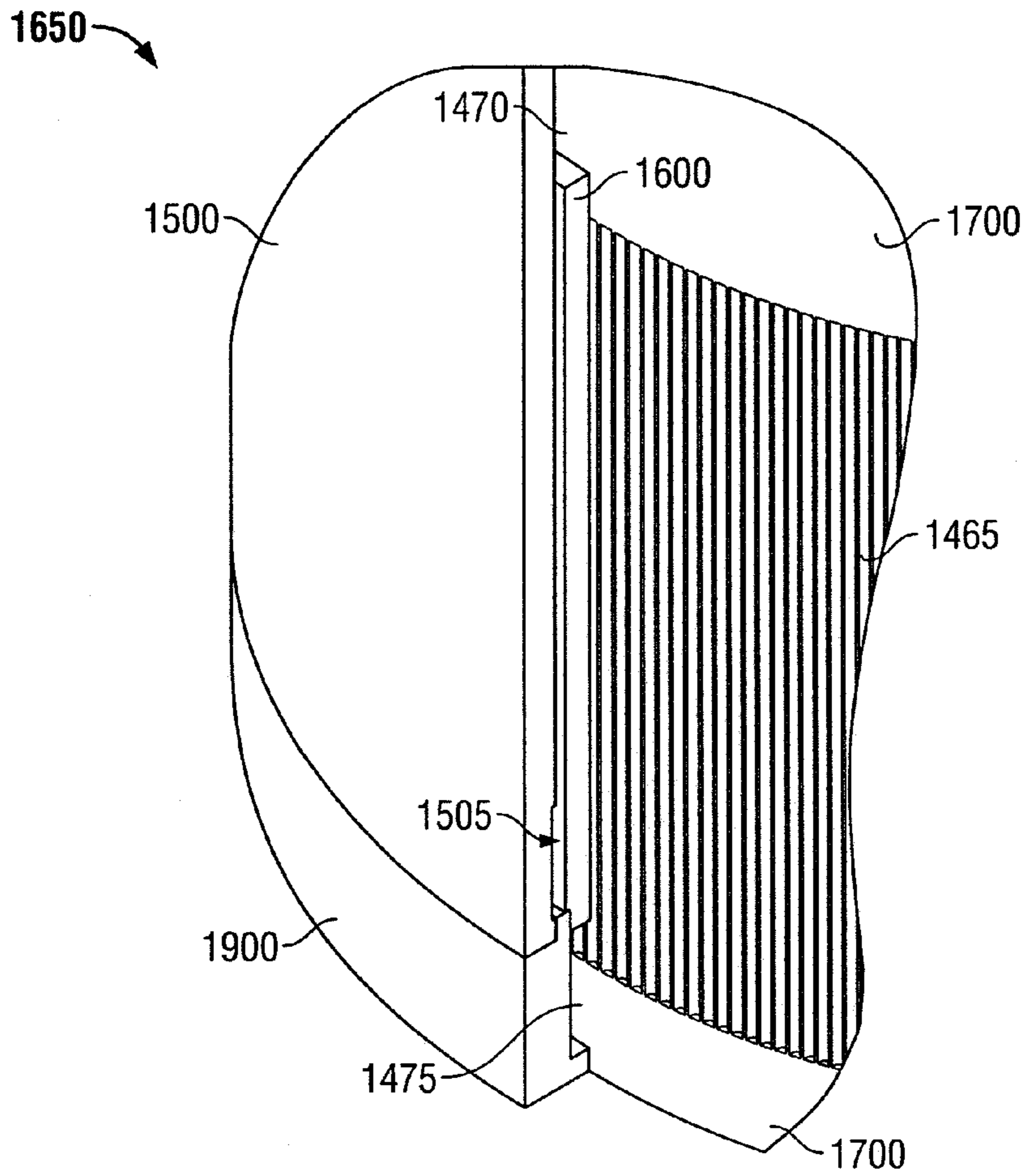
FIG. 14H
