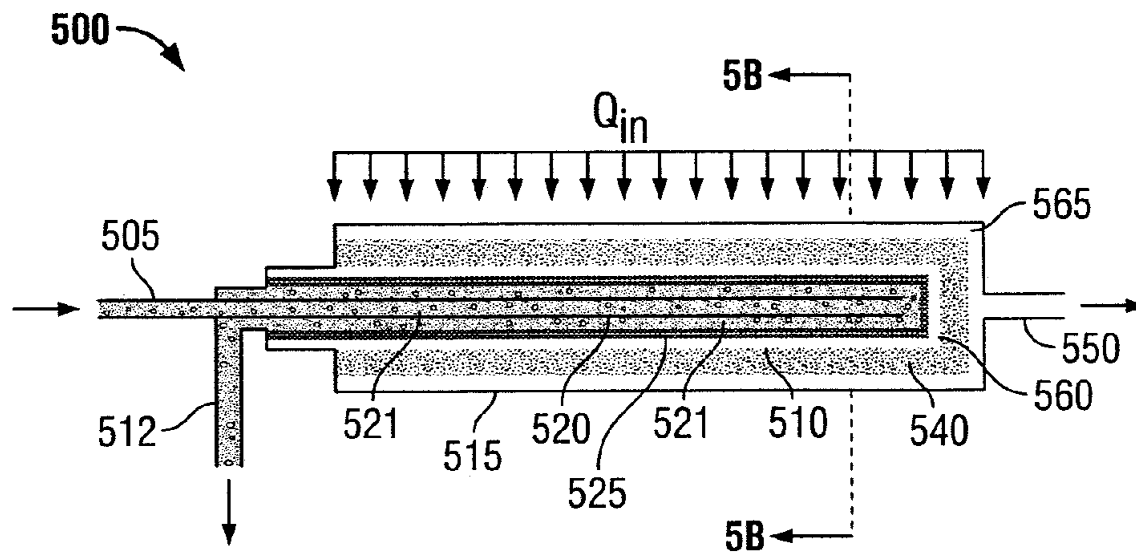
FIG. 5A
