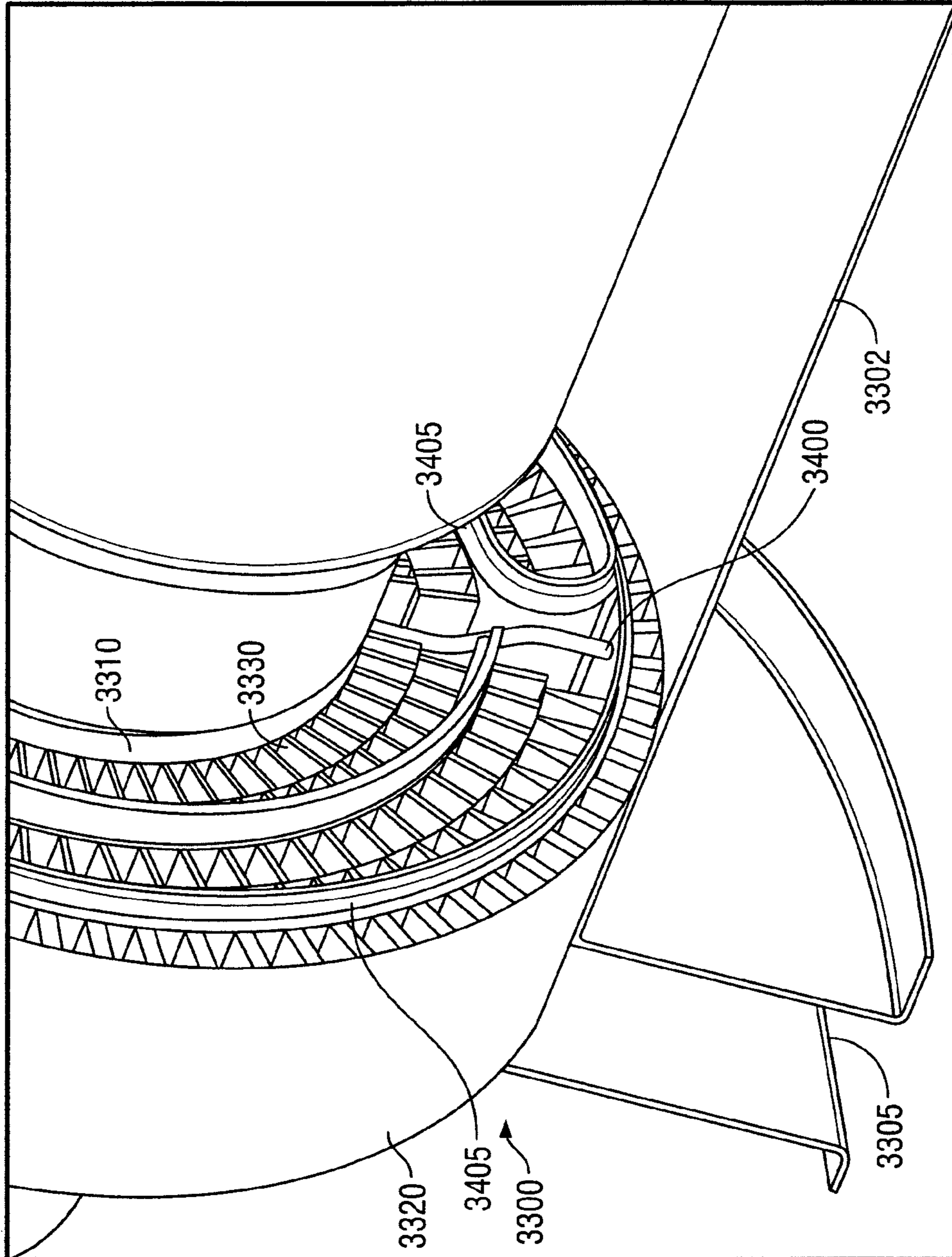
FIG. 34
