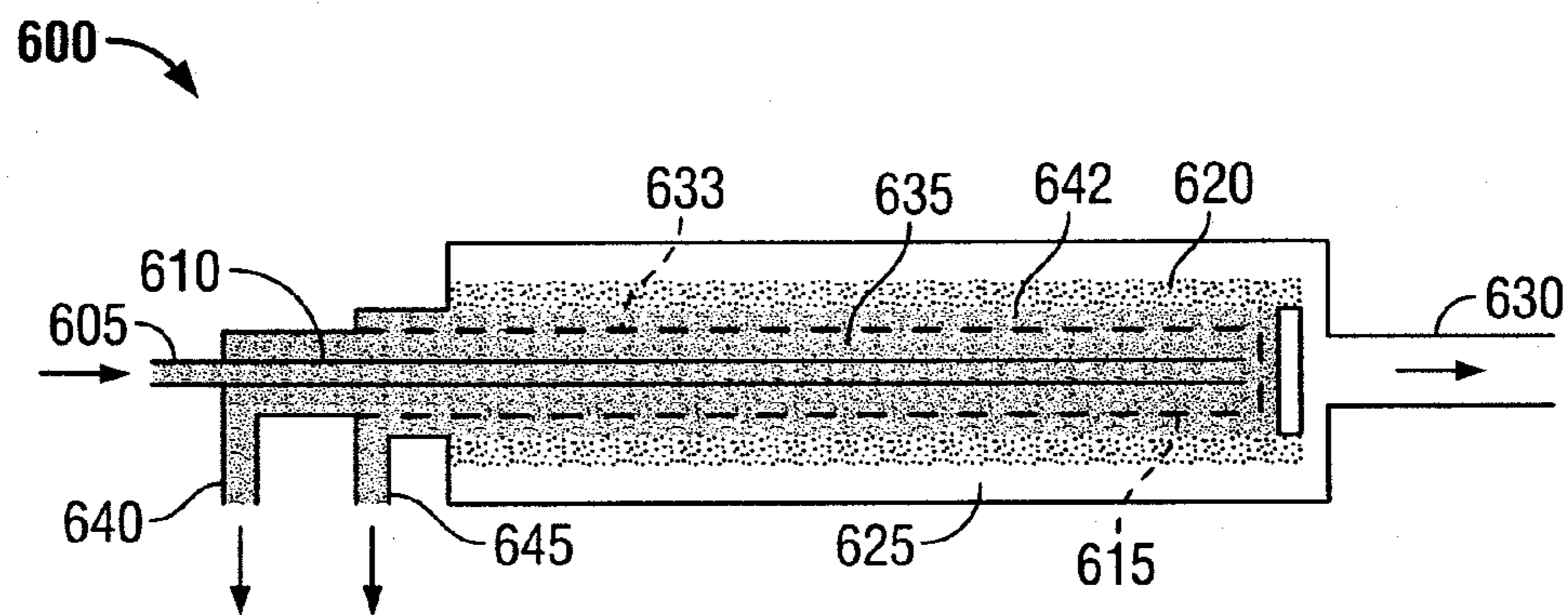
FIG. 6
