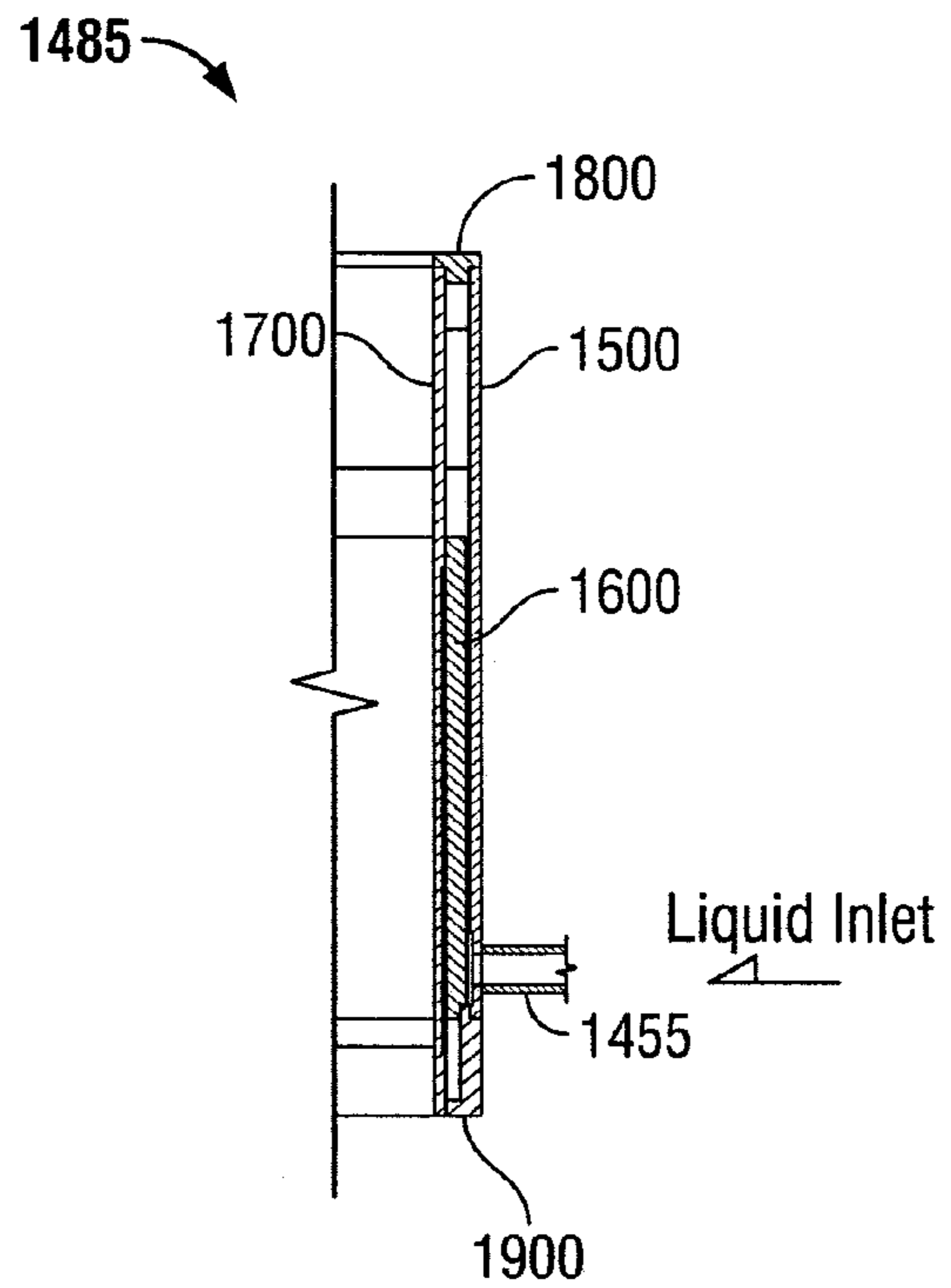
FIG. 14F
