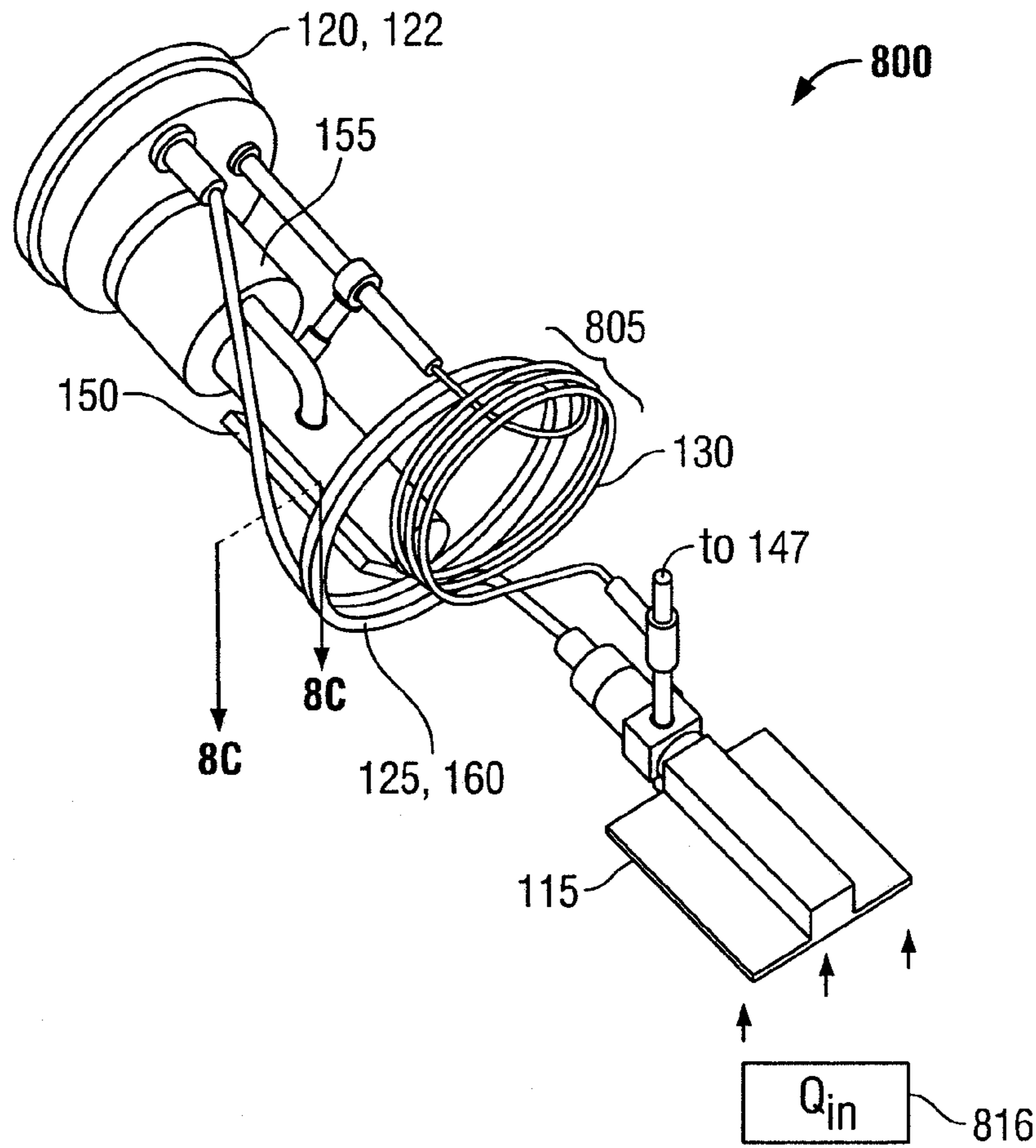
FIG. 8A
