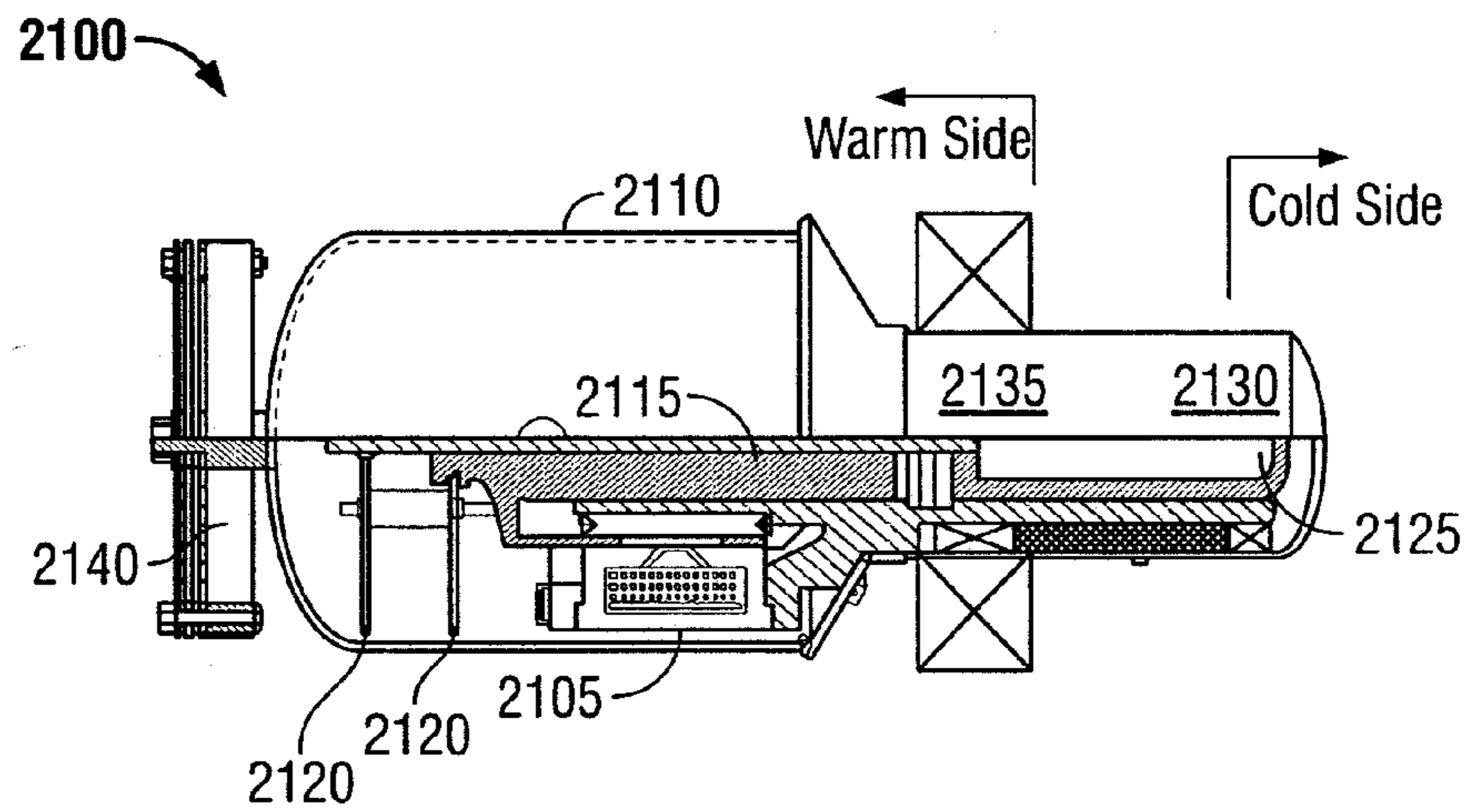
FIG. 21
