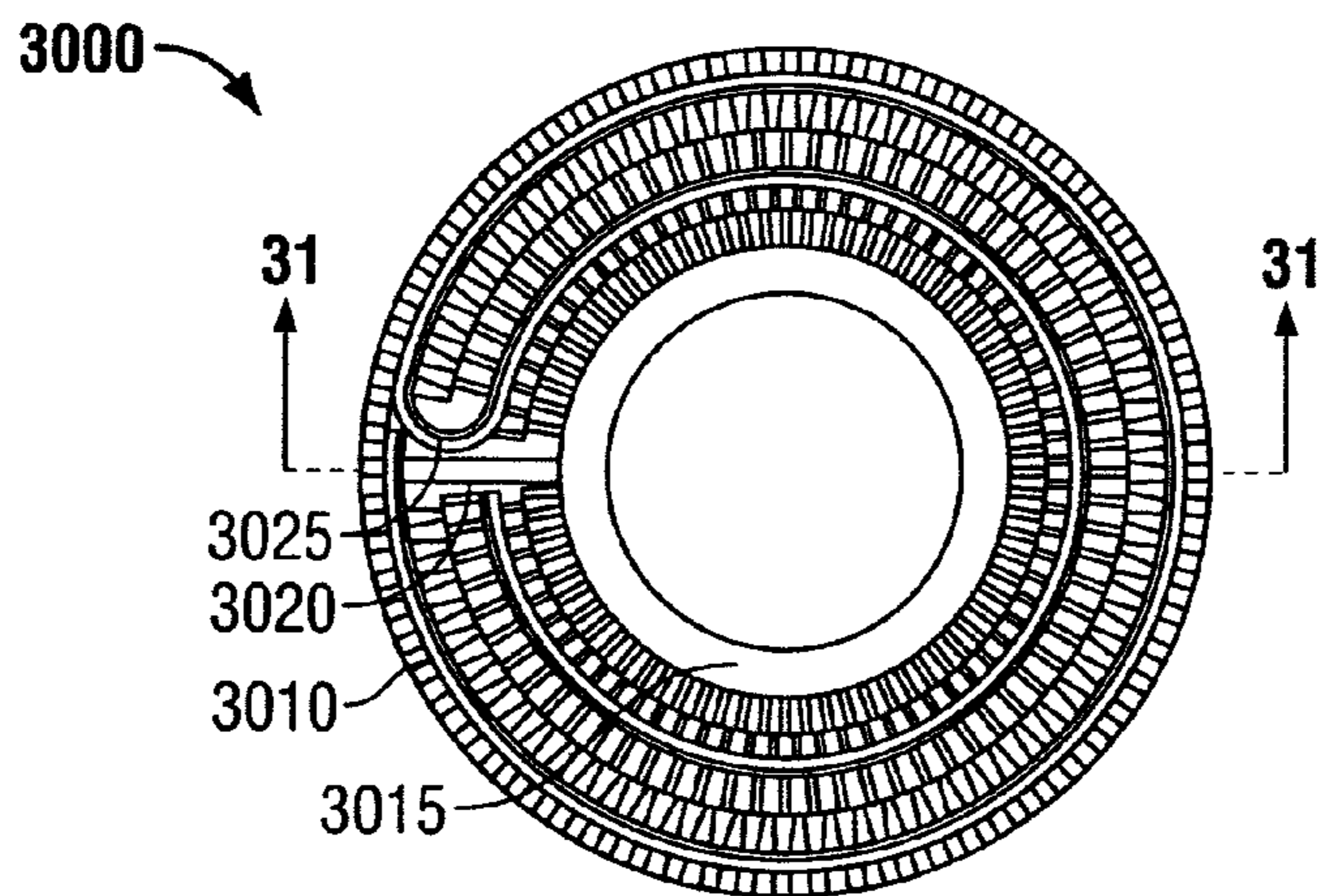
FIG. 30
