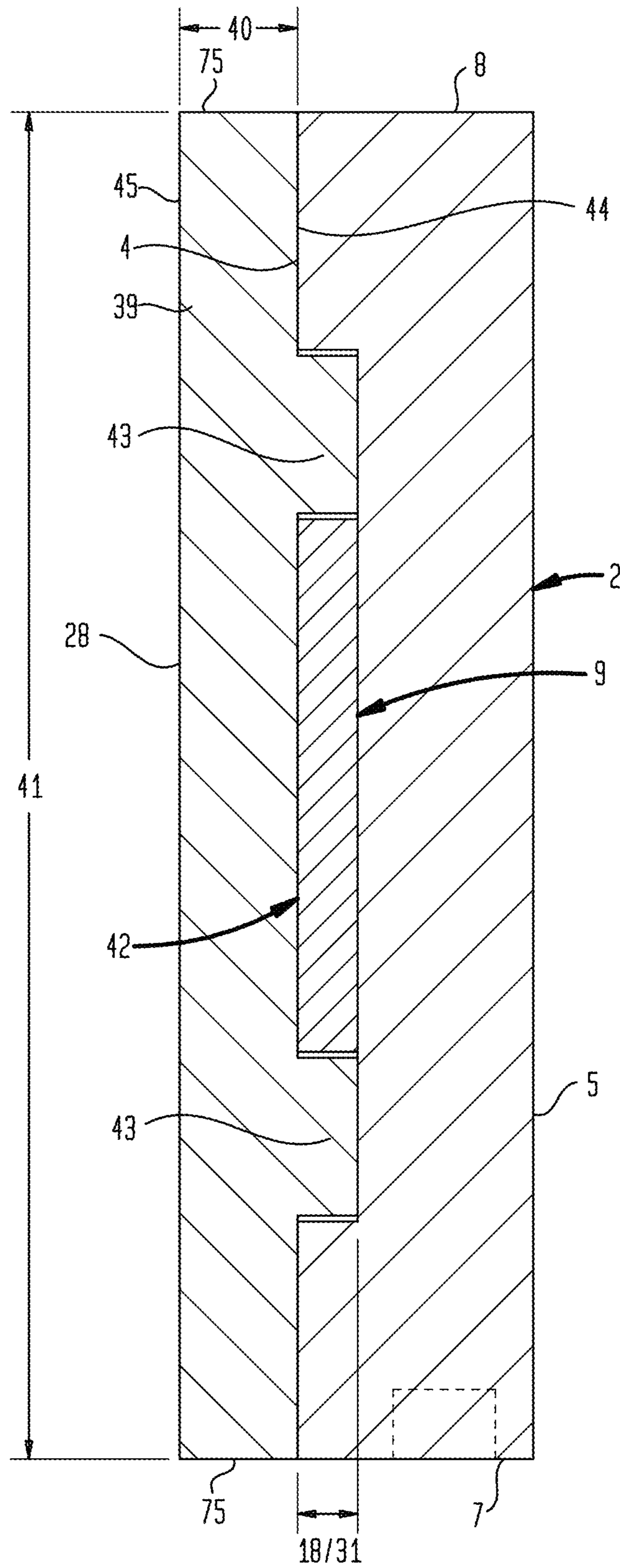
FIG. 9
