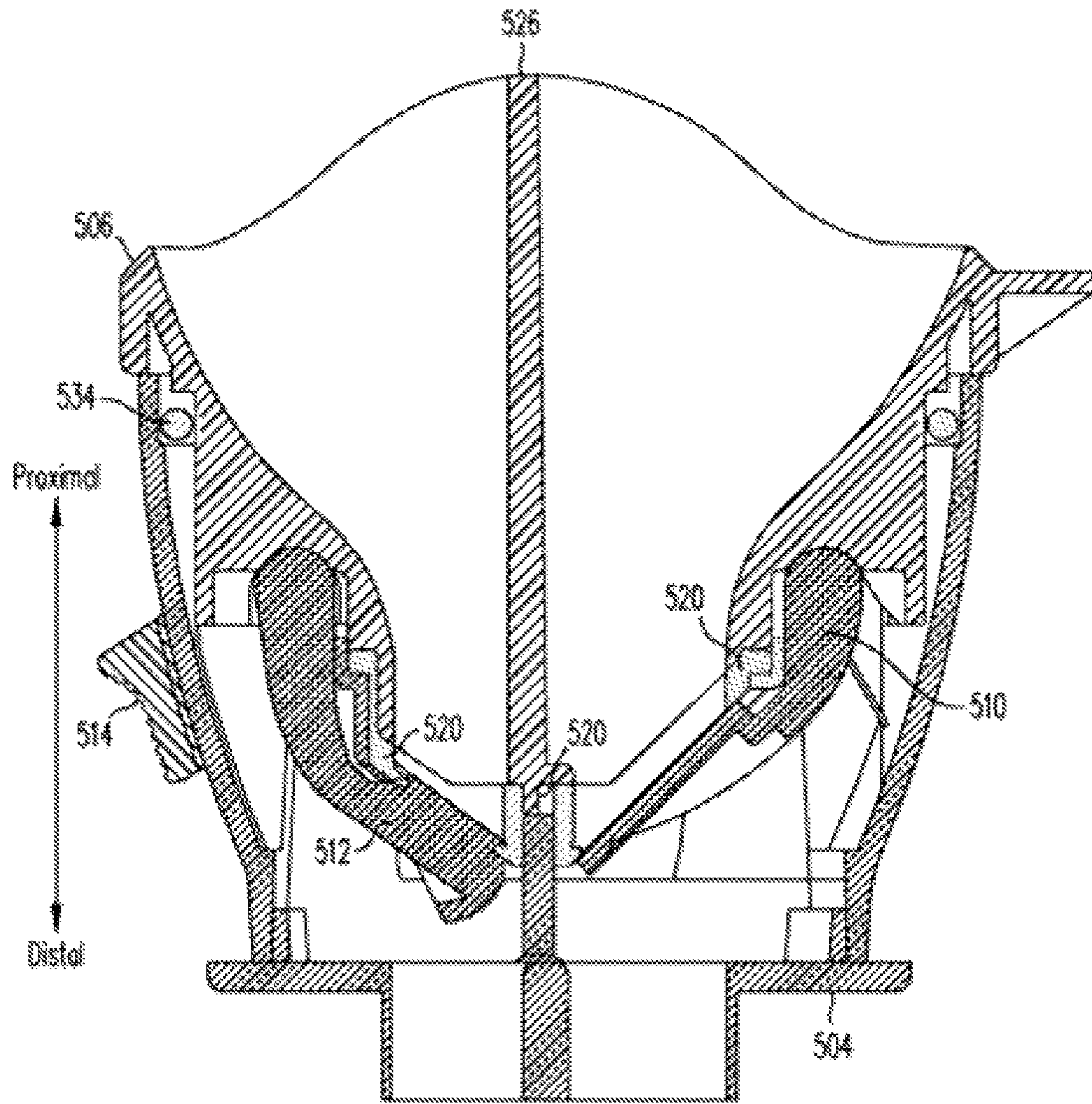
SECTION A-A
