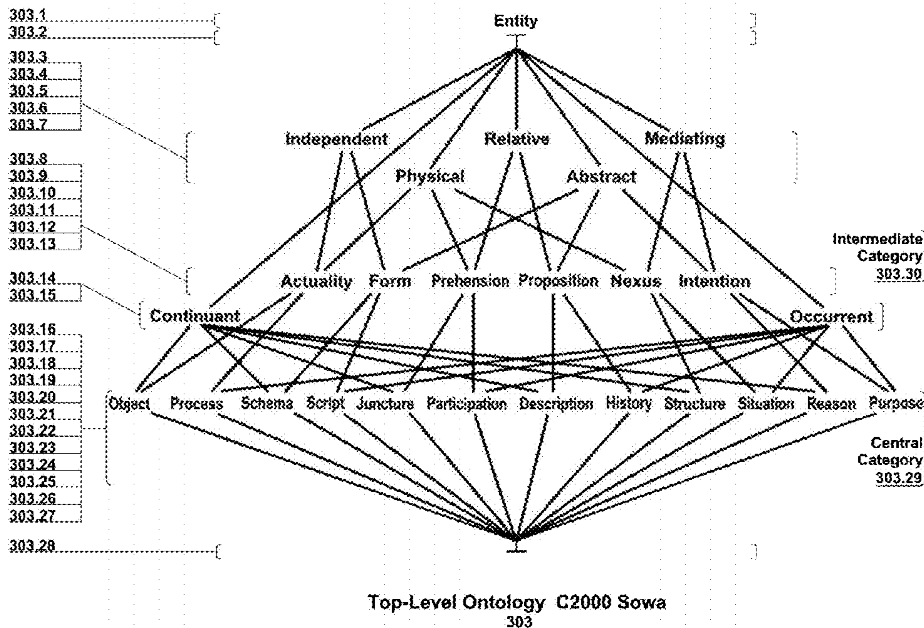
FIG. 24 Entity Ontology
