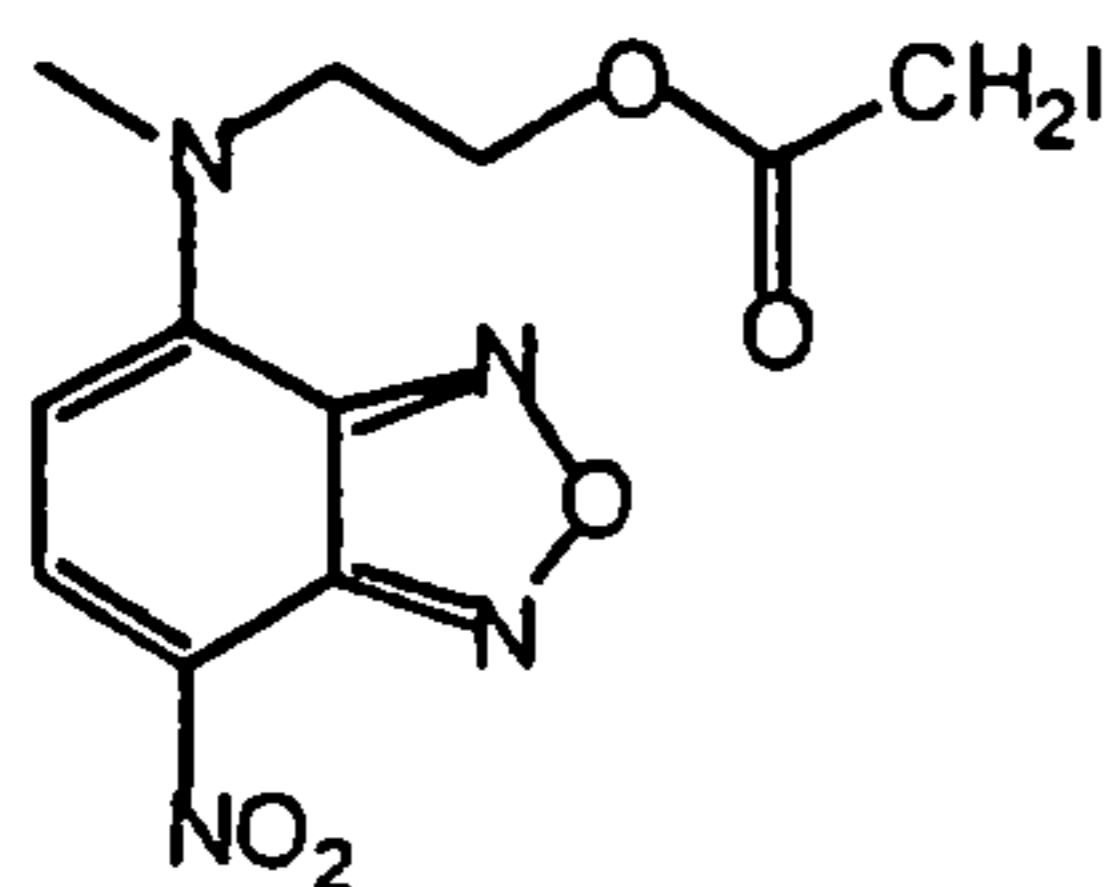
NBDE
