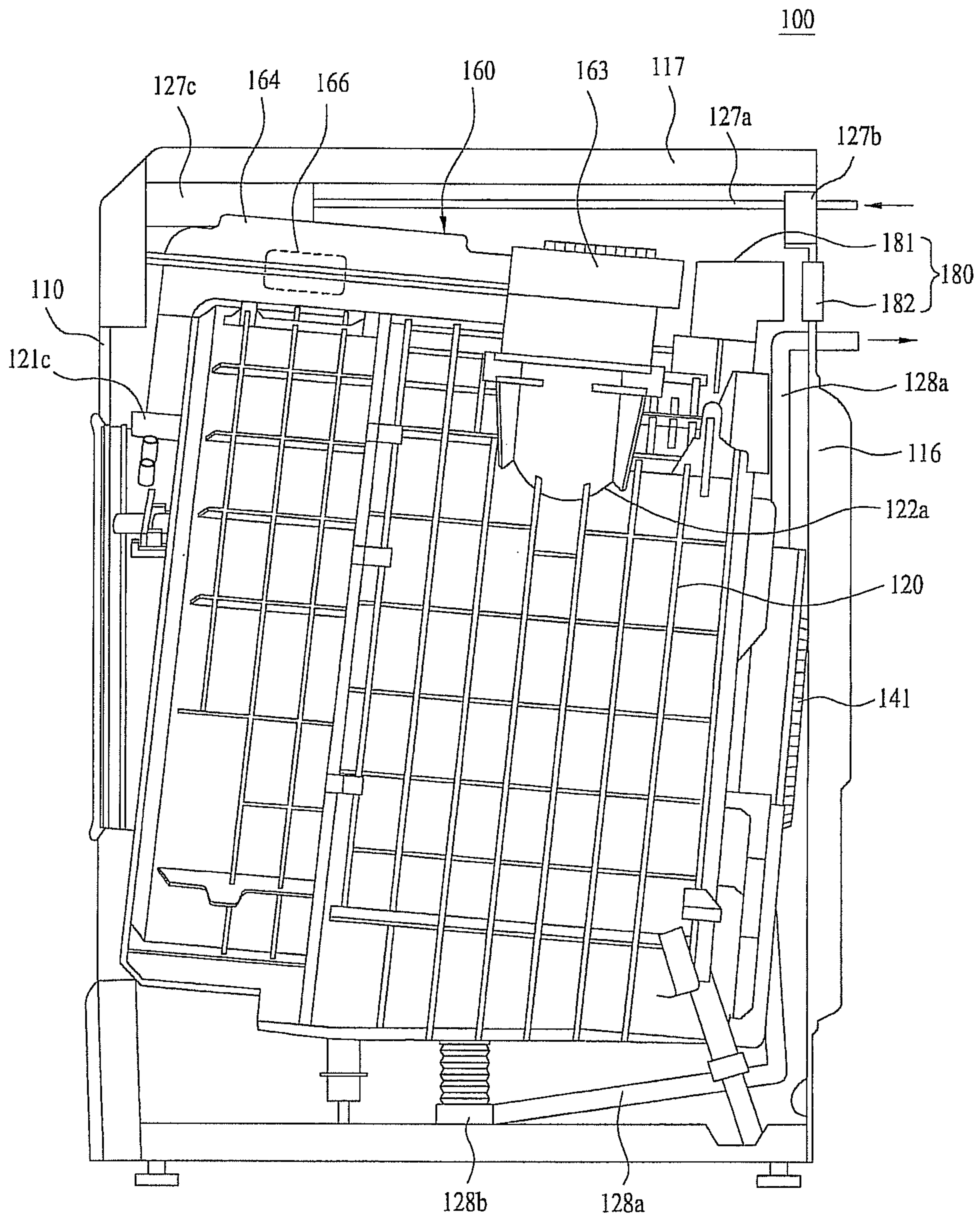
FIG. 9
