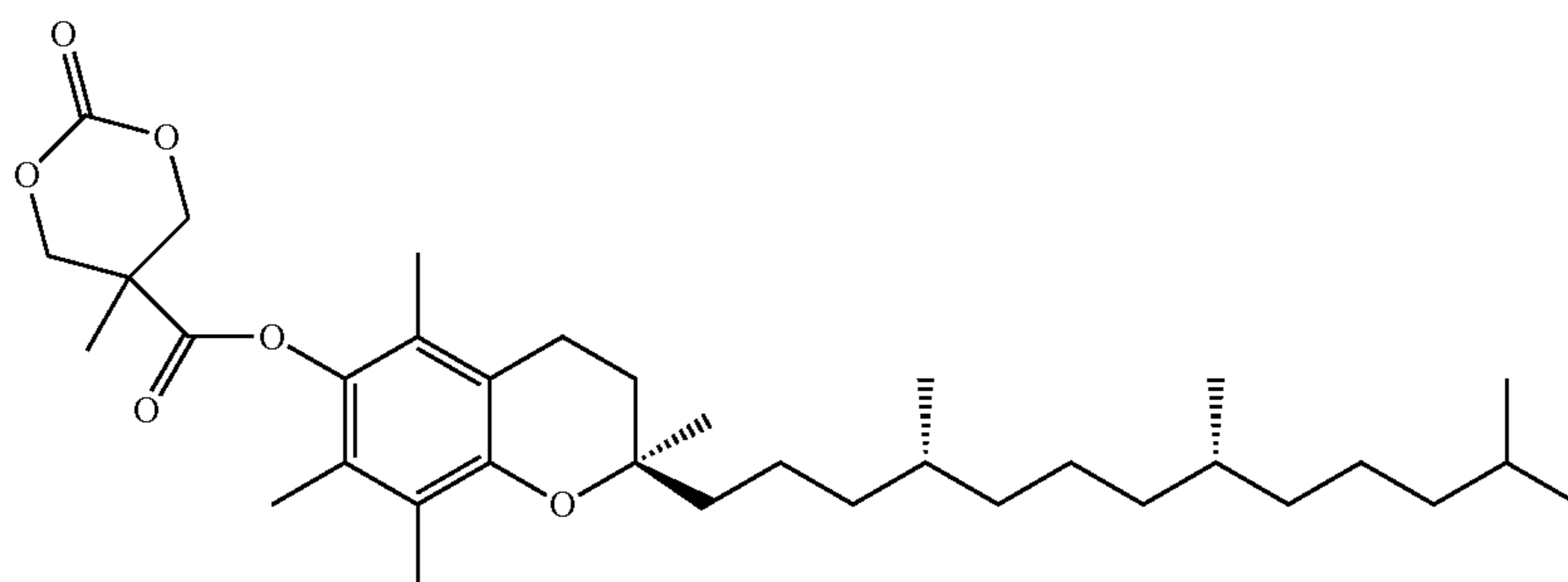
(MTC-VitE)
