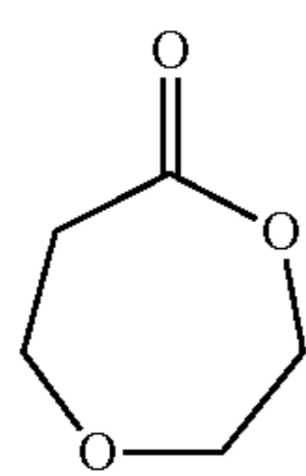
1,5-Dioxepan-2-one (DXO)
