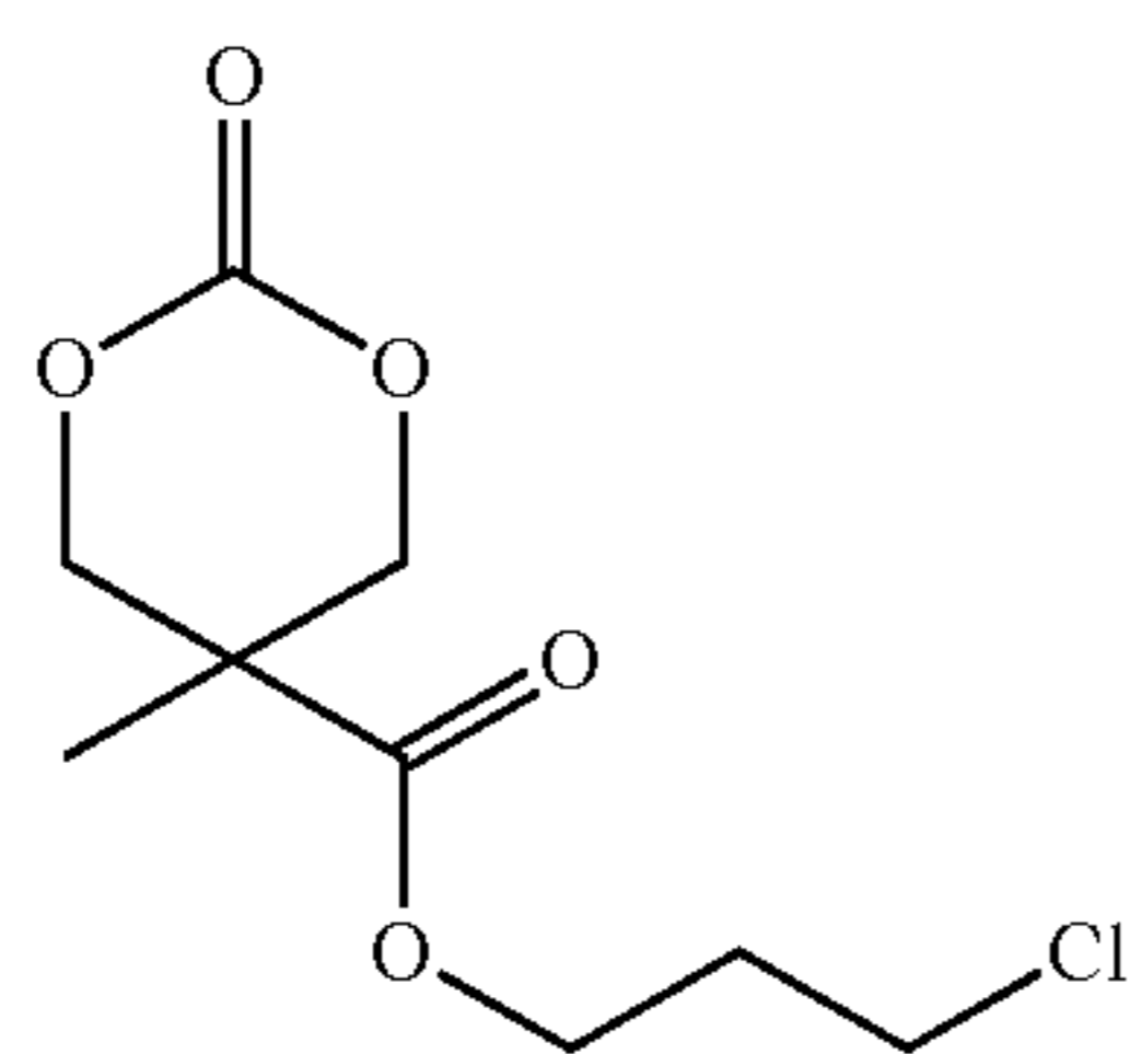
(MTC-PrCl)
