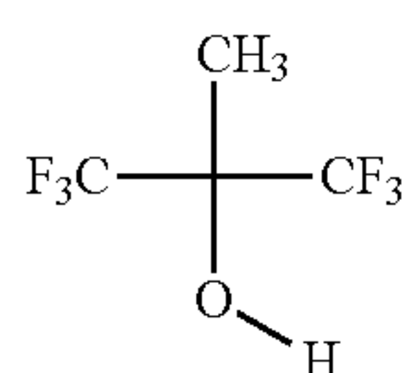
HFTB
