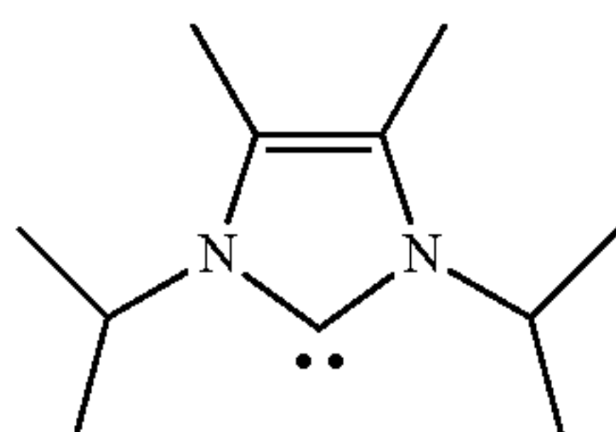
1,3-Bis(2-propyl)-4,5-dimethylimidazol-2-ylidene (Im-1)
