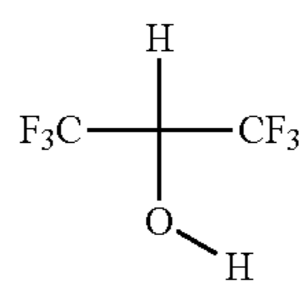
HFIP
