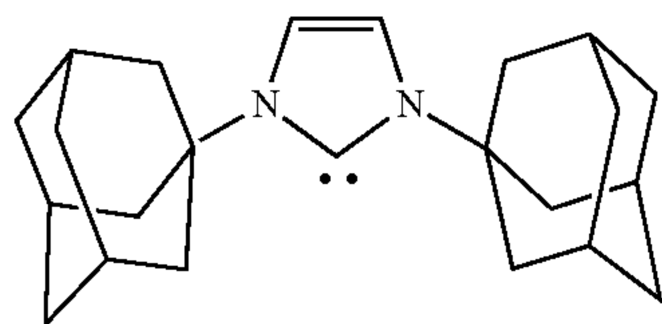
1,3-Bis(1-adamantyl)imidazol-2-ylidene (Im-4)
