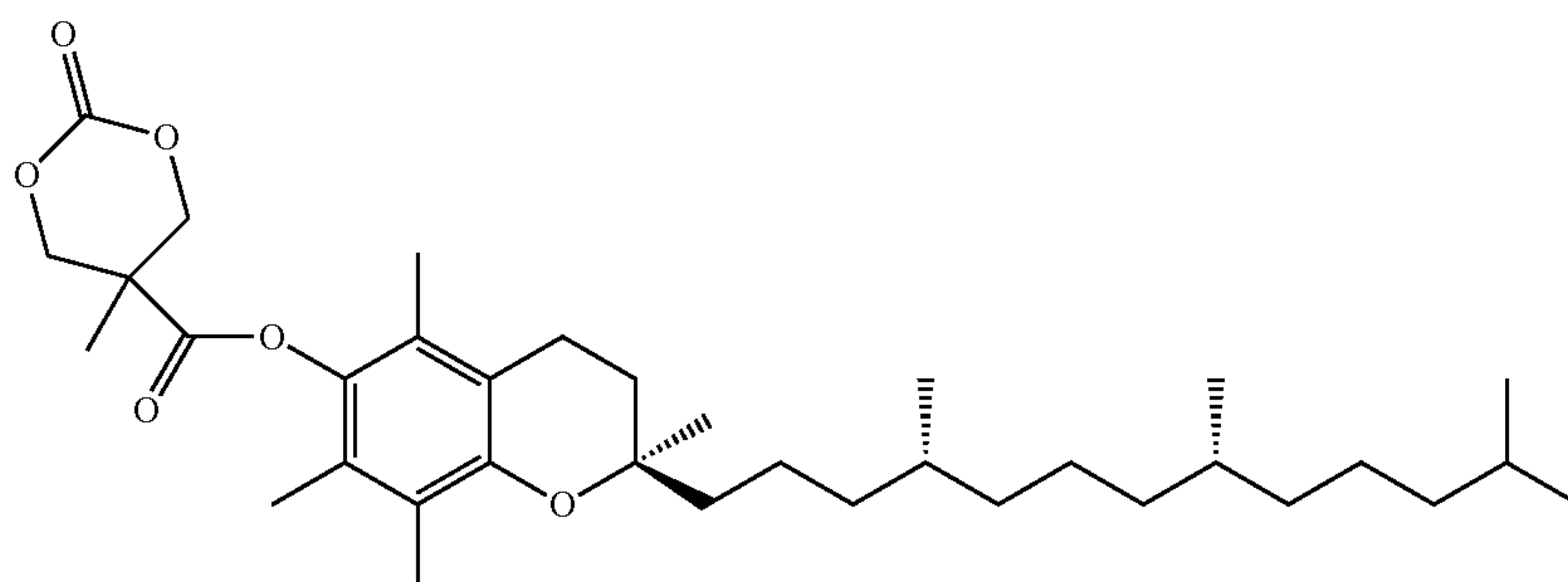
(MTC-VitE)
