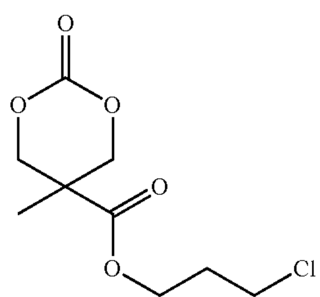
(MTC-PrCl)
