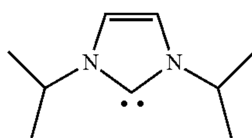
1,3-Di-i-propylimidazol-2-ylidene (Im-5)
