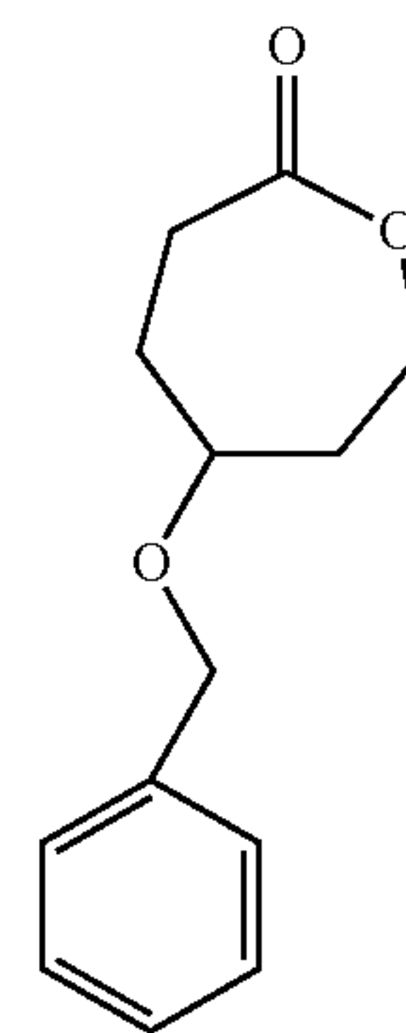
5-(Benzyloxy)oxepan-2-one (BXO)
