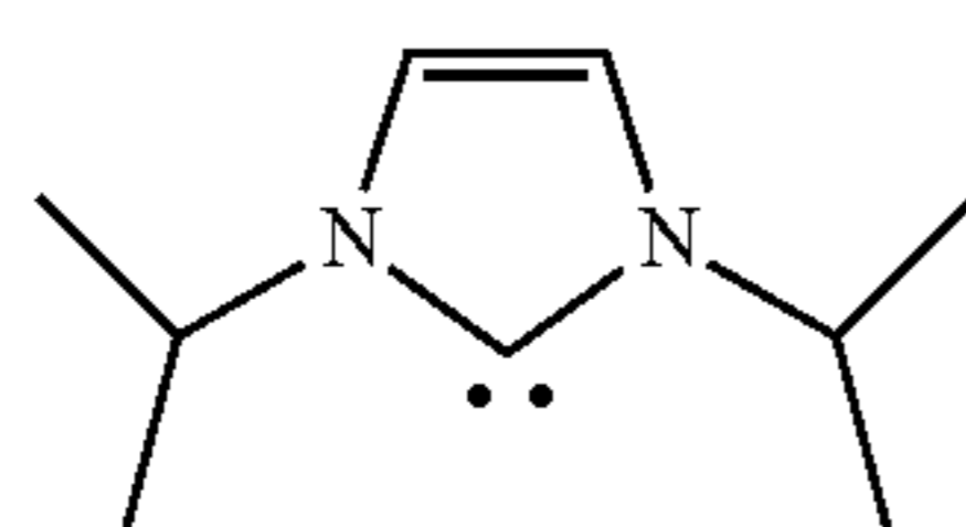
1,3-Di-i-propylimidazol-2-ylidene (Im-5)
