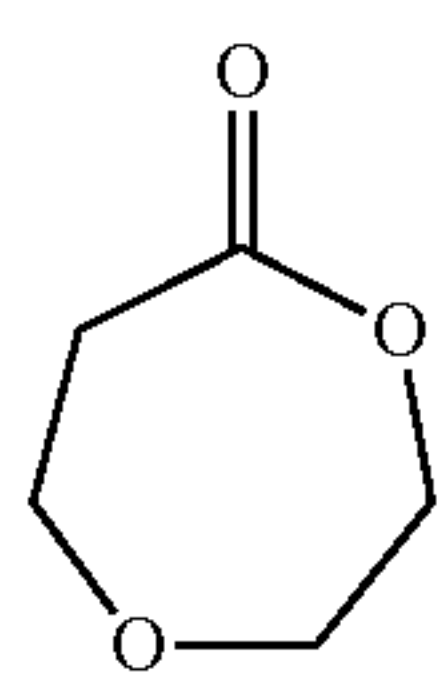
1,5-Dioxepan-2-one (DXO)
