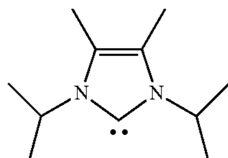
1,3-Bis(2-propyl)-4,5-dimethylimidazol-2-ylidene (Im-1)
