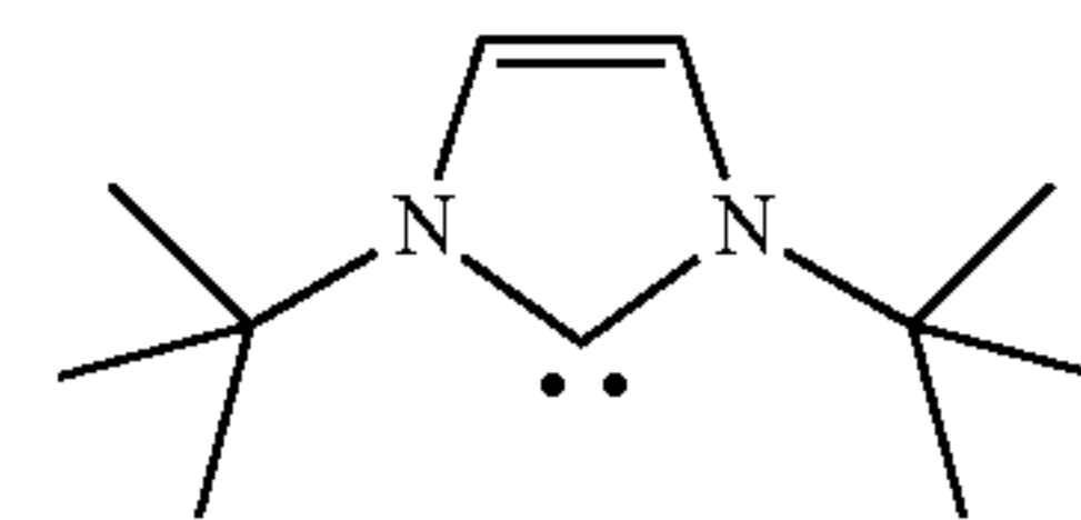
1,3-Di-t-butylimidazol-2-ylidene (Im-6)
