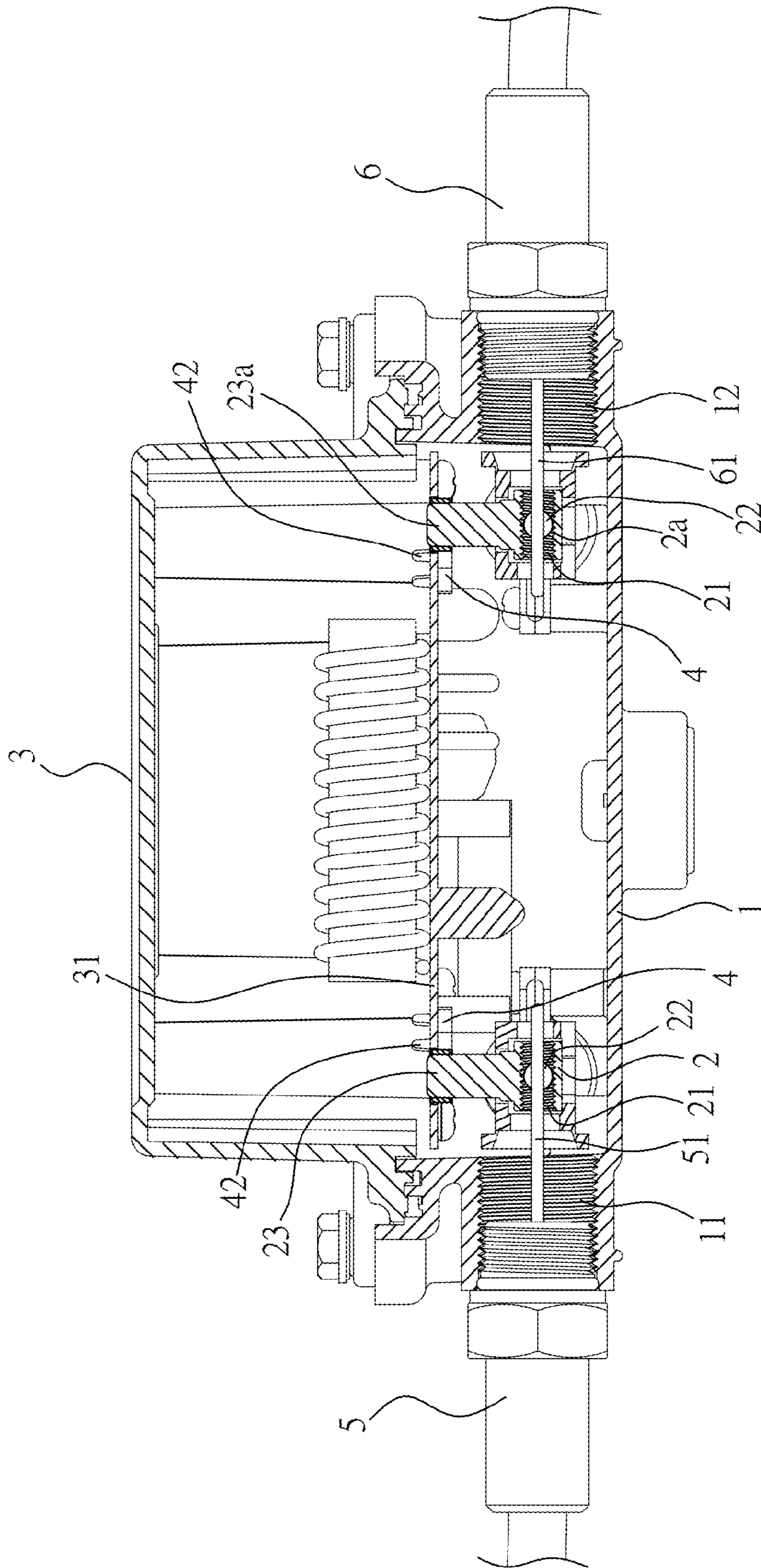
A-A FIG. 5
