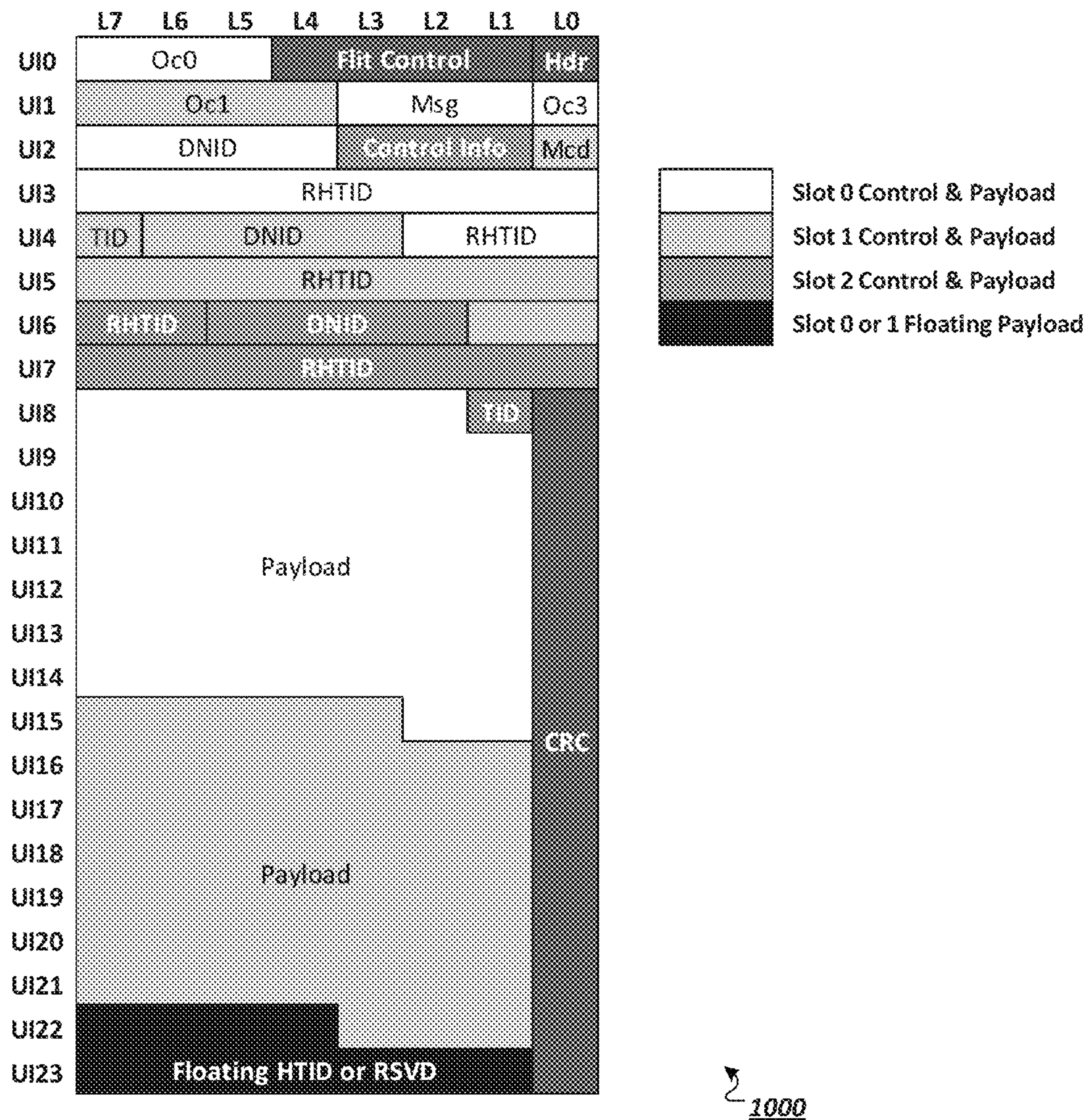
FIG. 10
