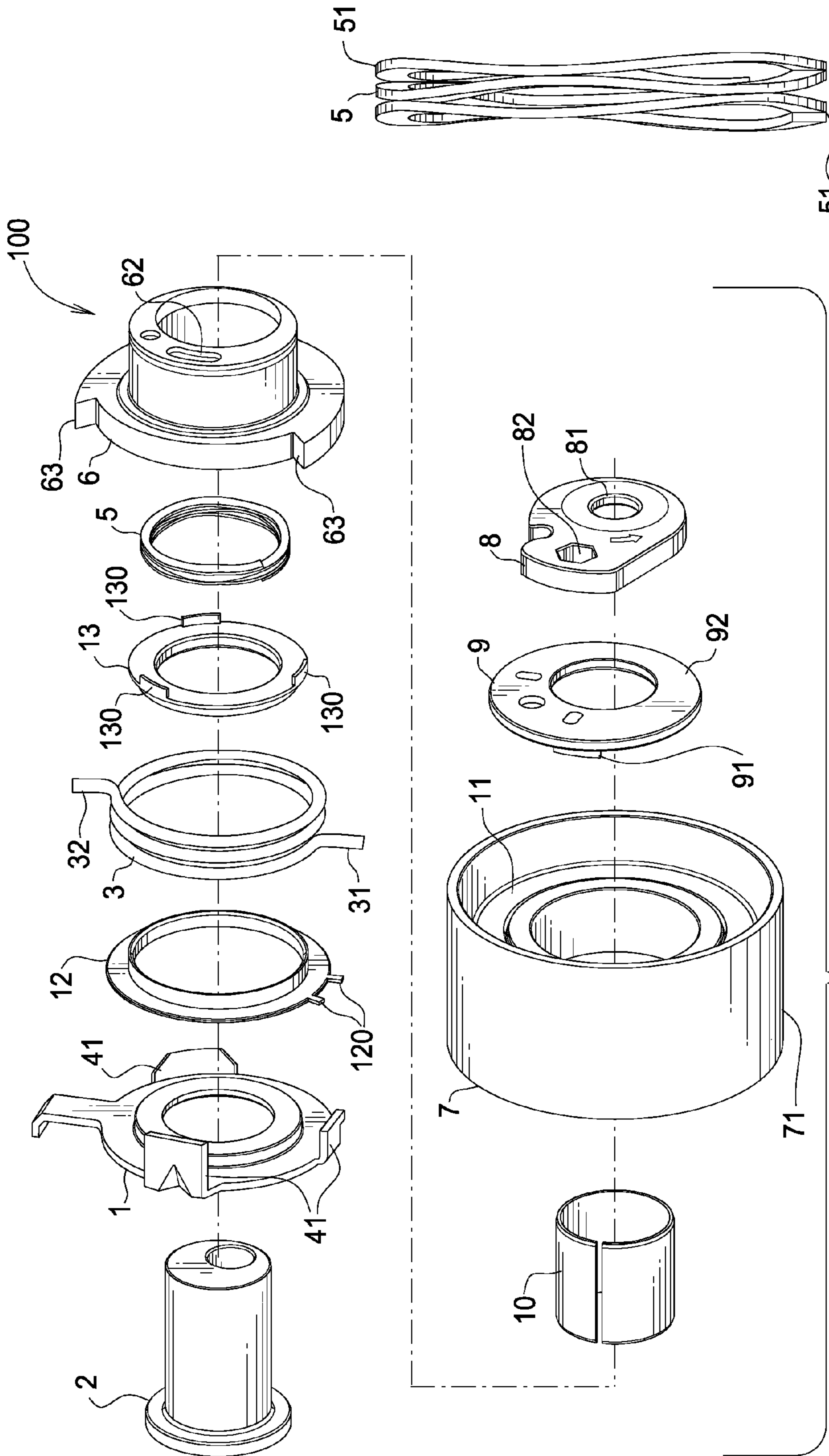
FIG.2B
