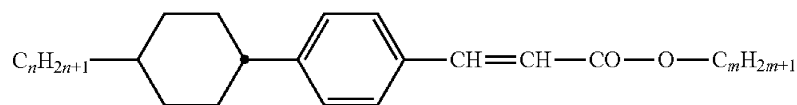
CP-n-VZm
