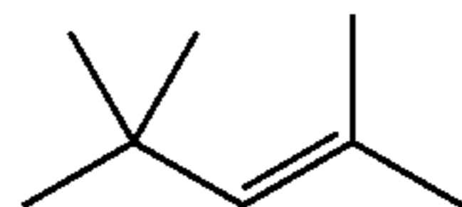
2,4,4-trimethylpent-2-ene (β-DIB)
