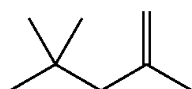
2,4,4-trimethylpent-1-ene (α-DIB)
