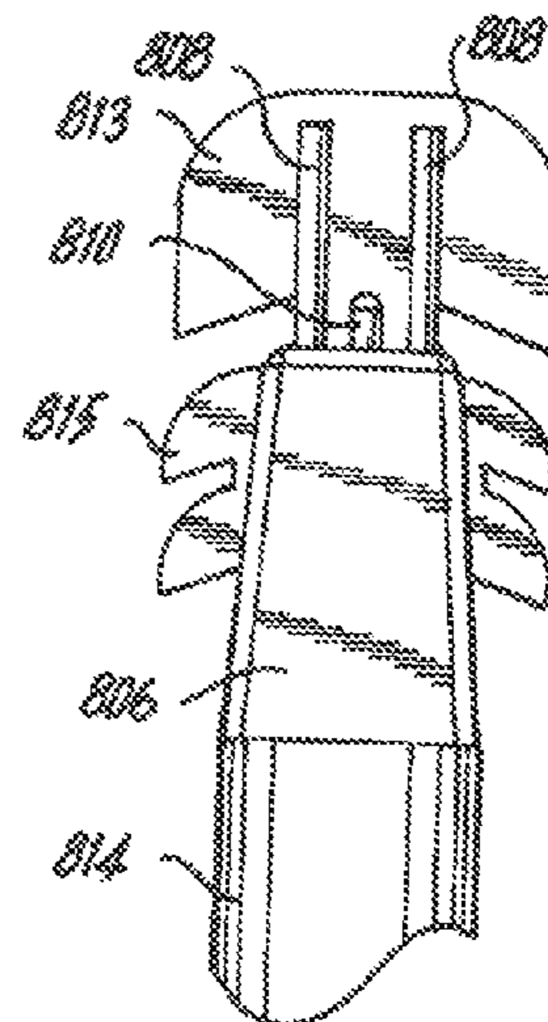
Fig. 68B
