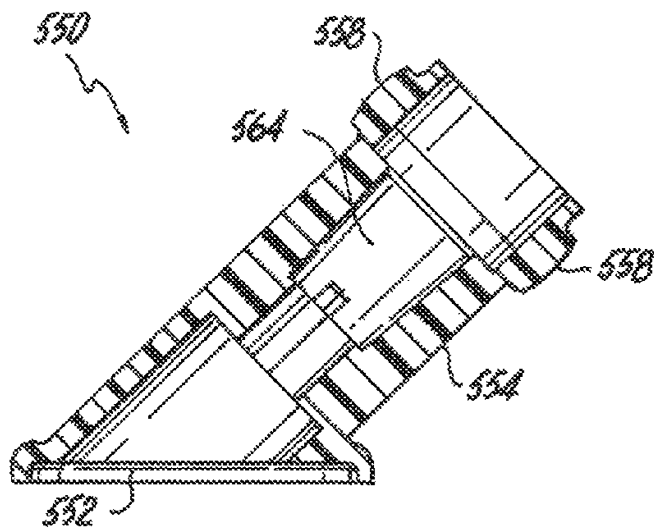
Fig. 41B
