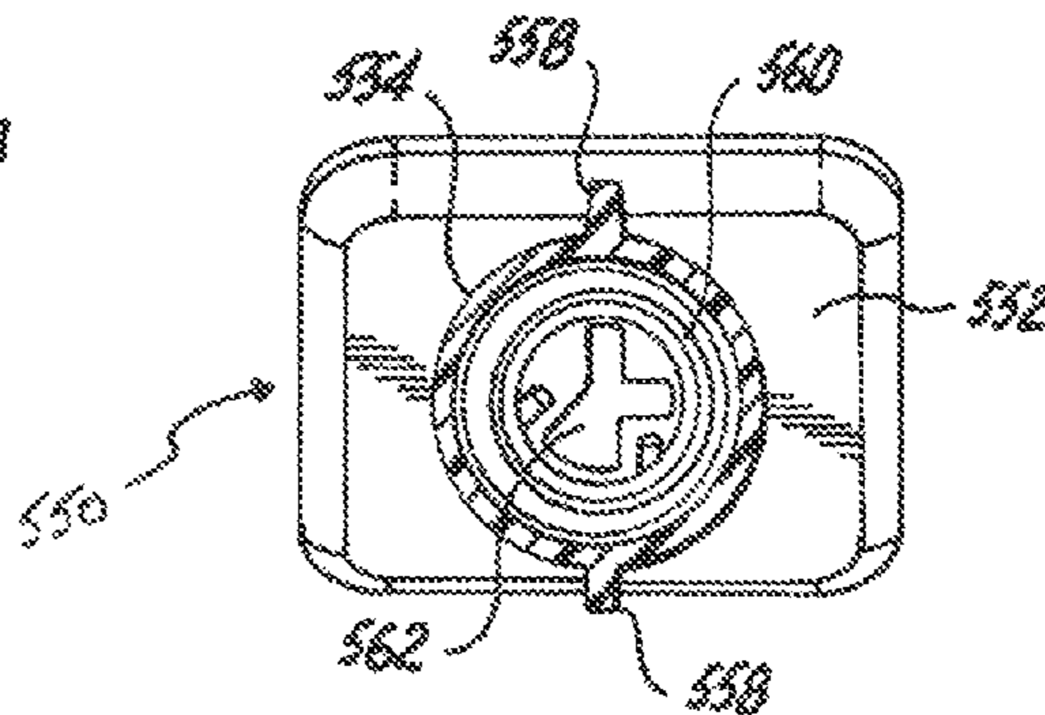
Fig. 41C
