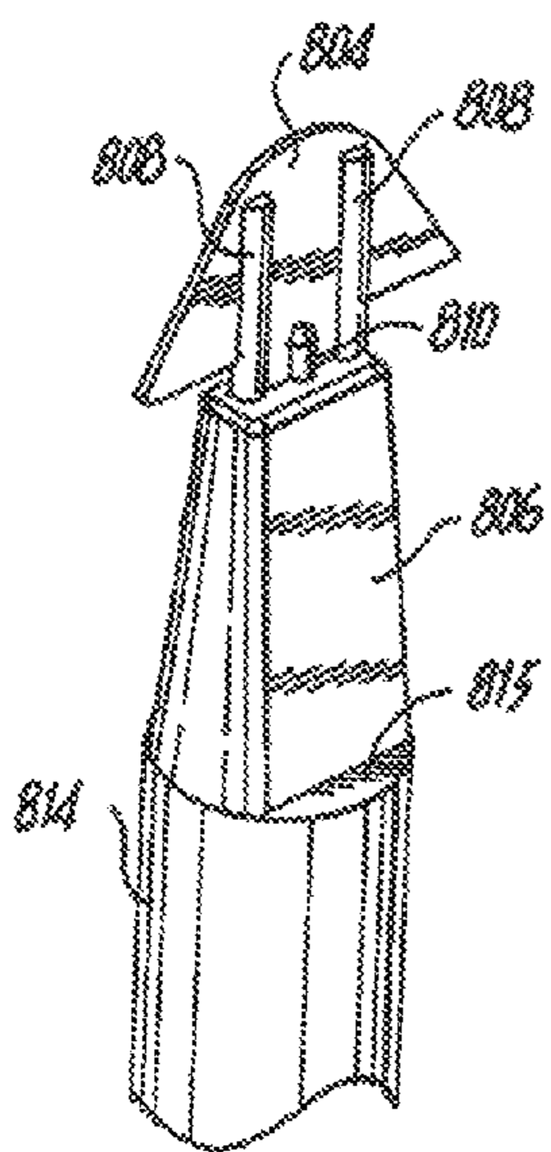
Fig. 66A
