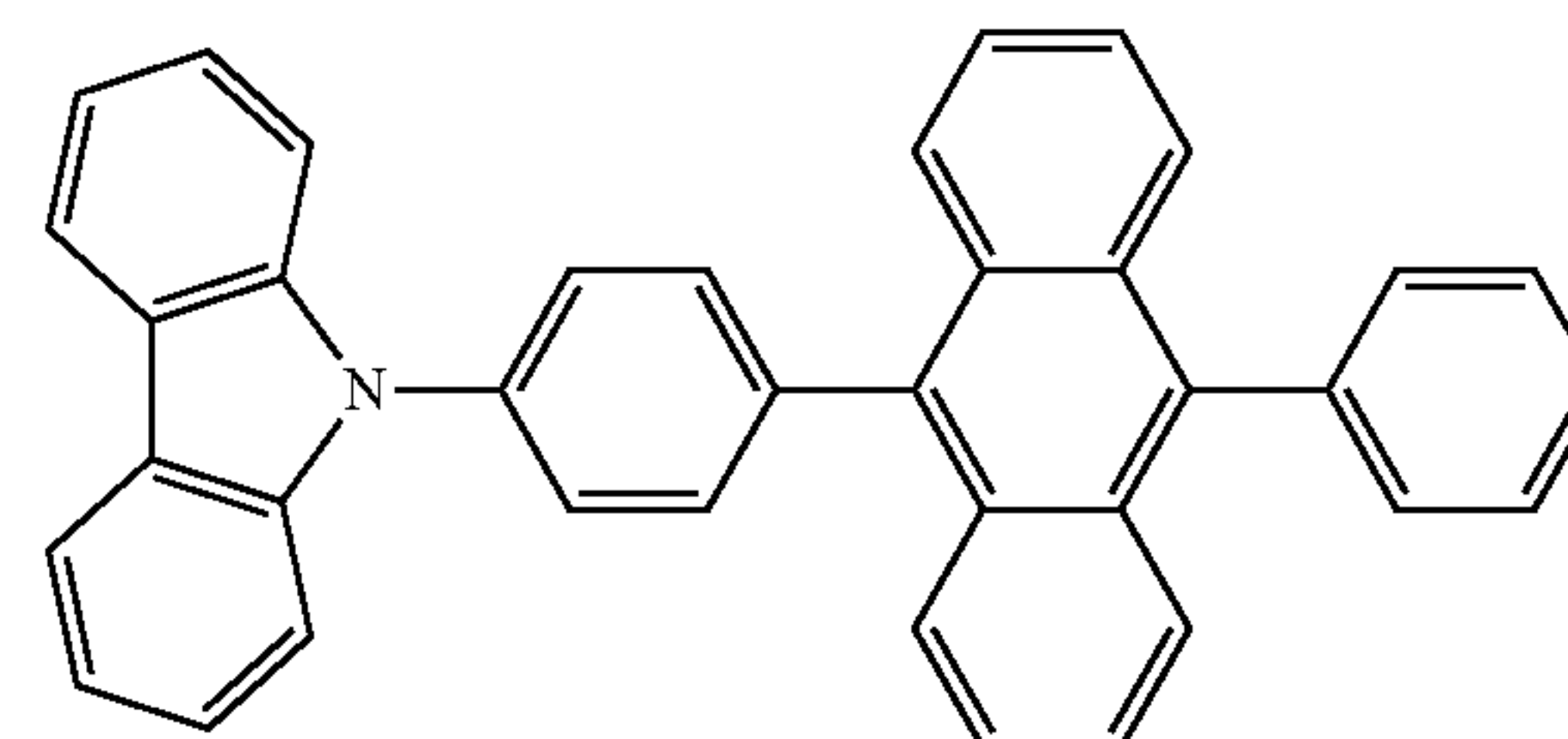
CzPA
