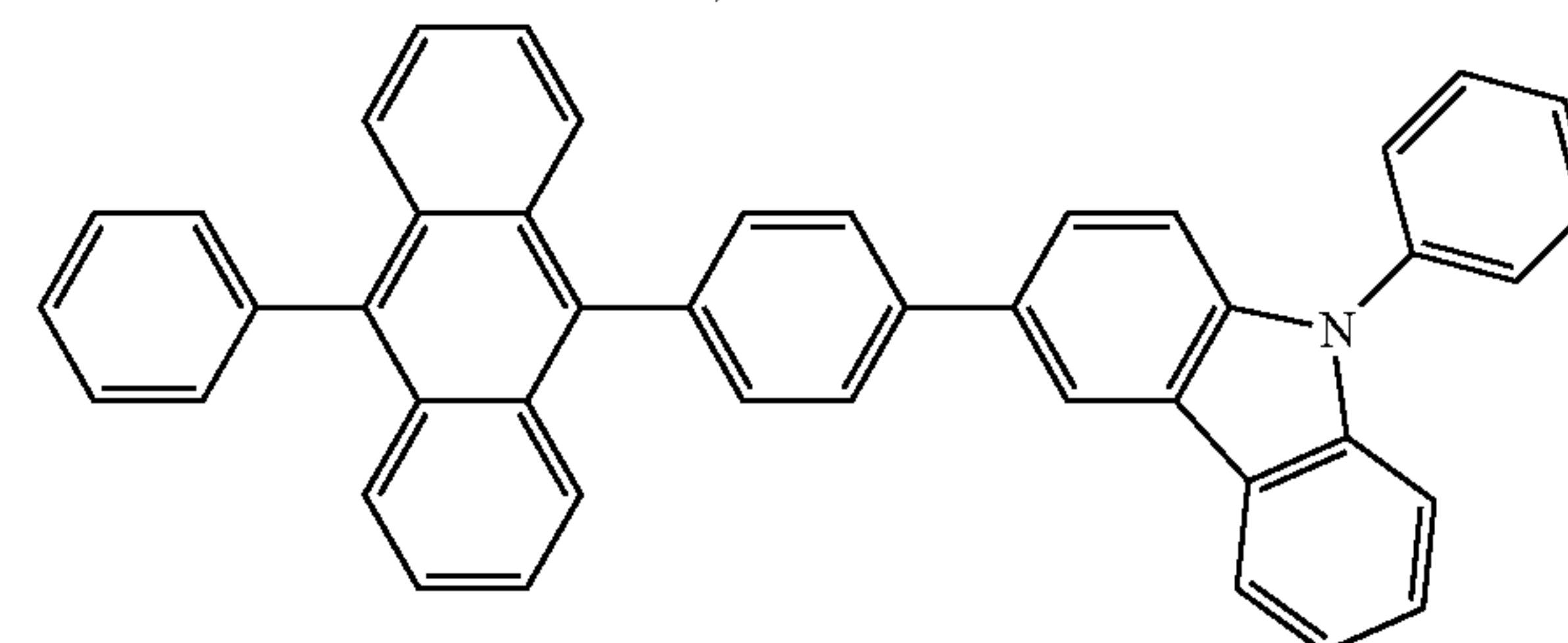
PCzPA
