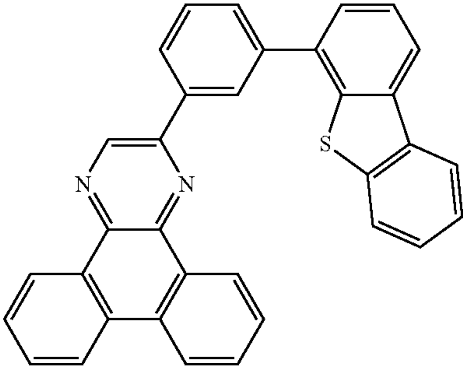
2mDBTPDBq-II
