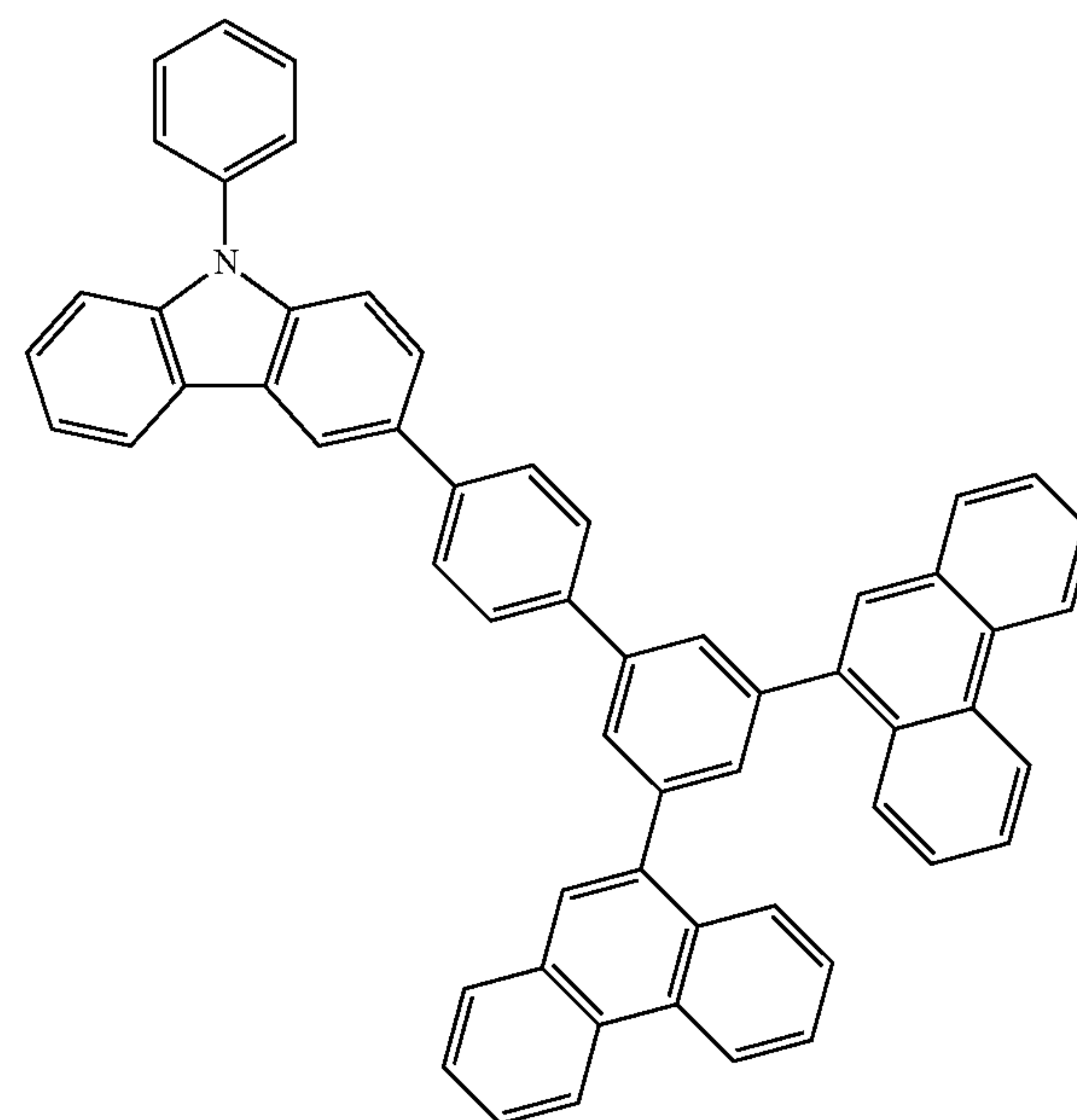
Pn2BPPC
