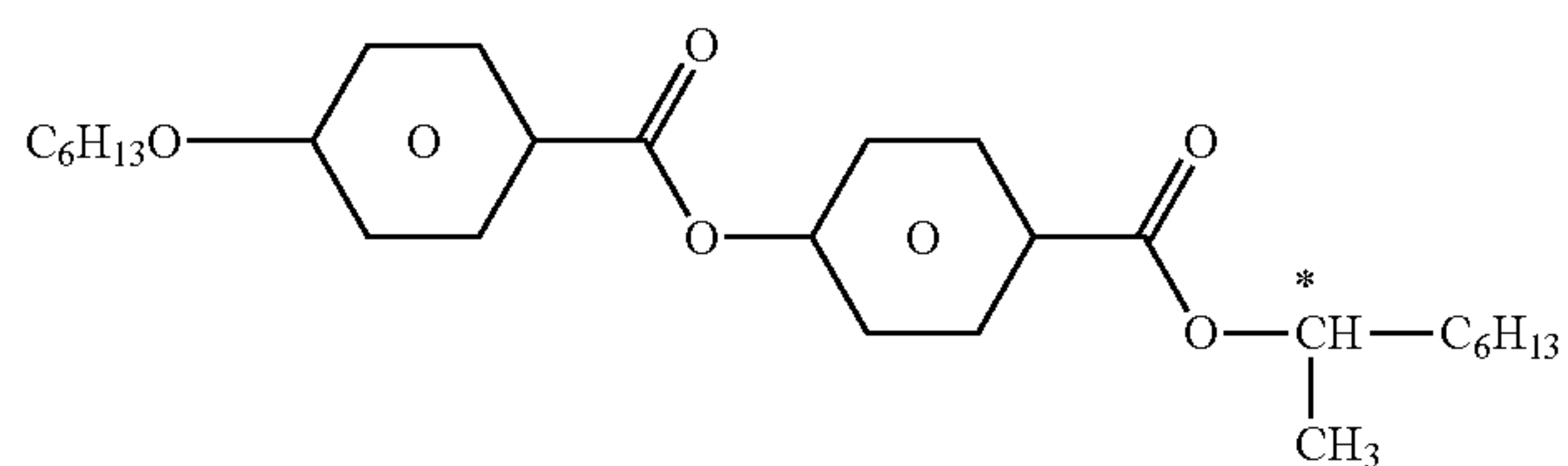
R/S-811
