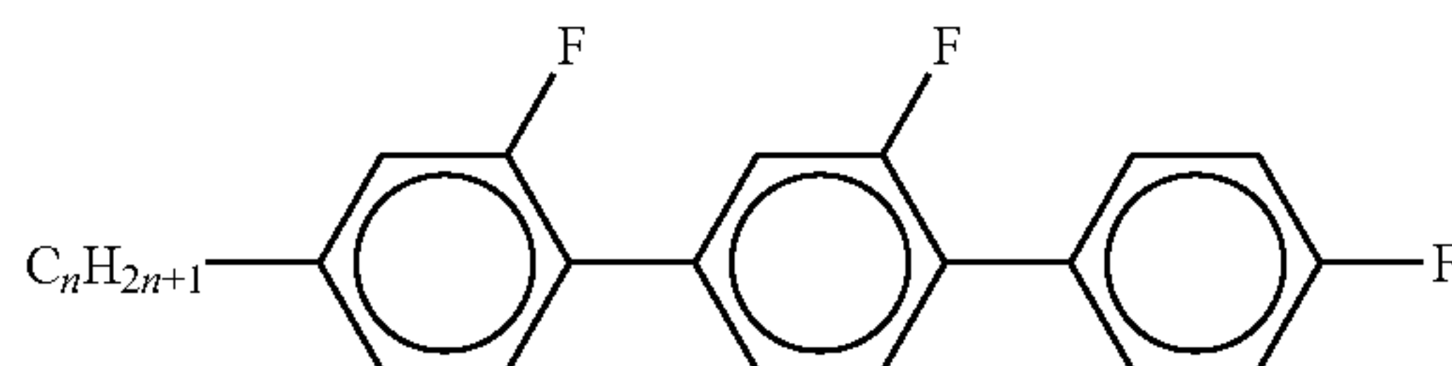
GGP-n-F
