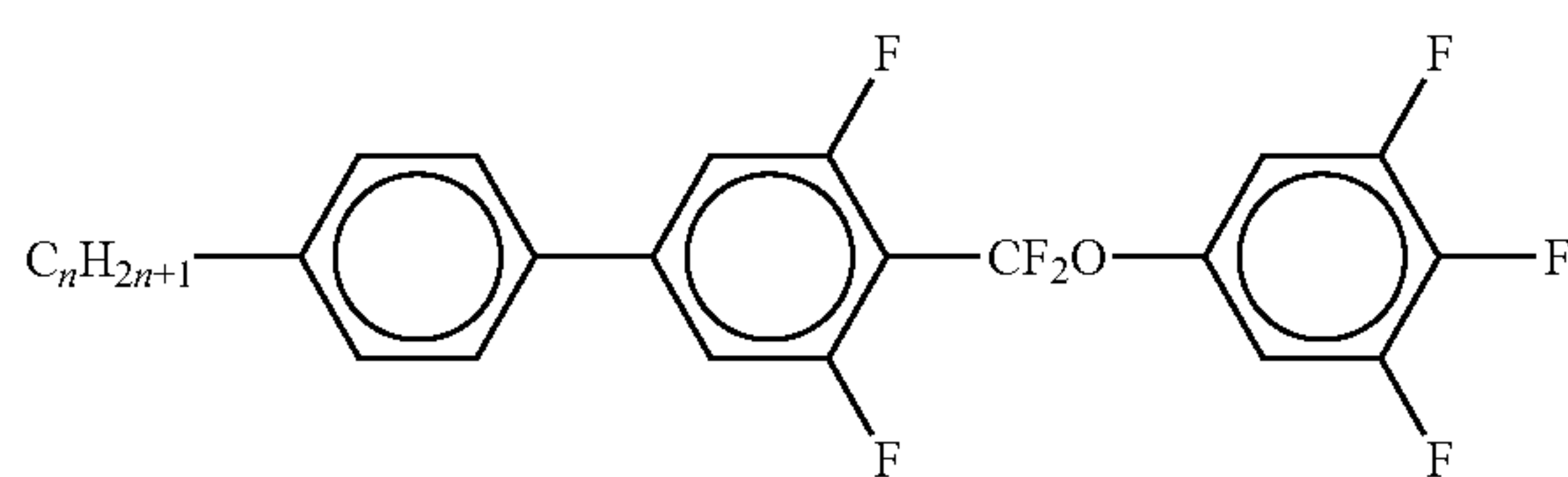
PUQU-n-F
