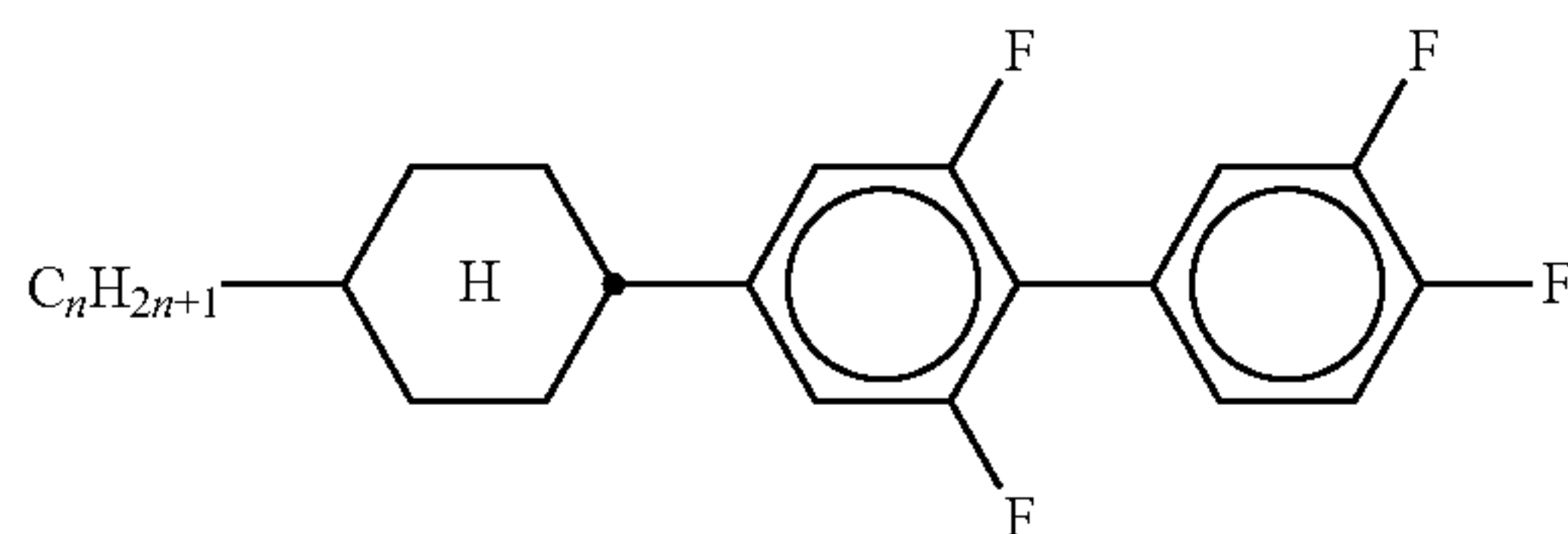
CUP-nF•F
