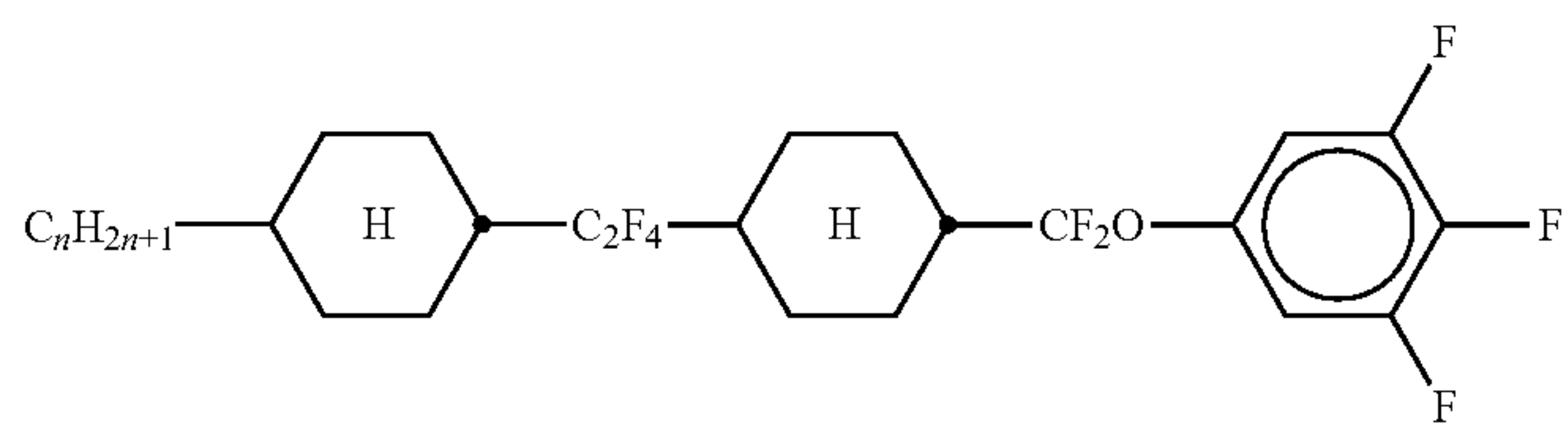
CWCQU-n-F
