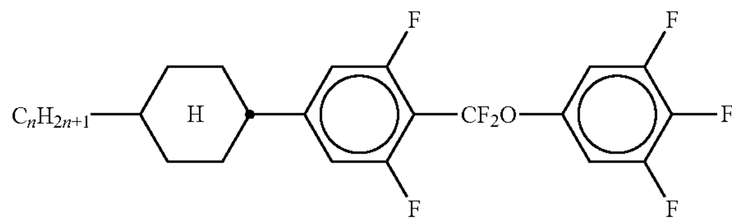
CUQU-n-F
