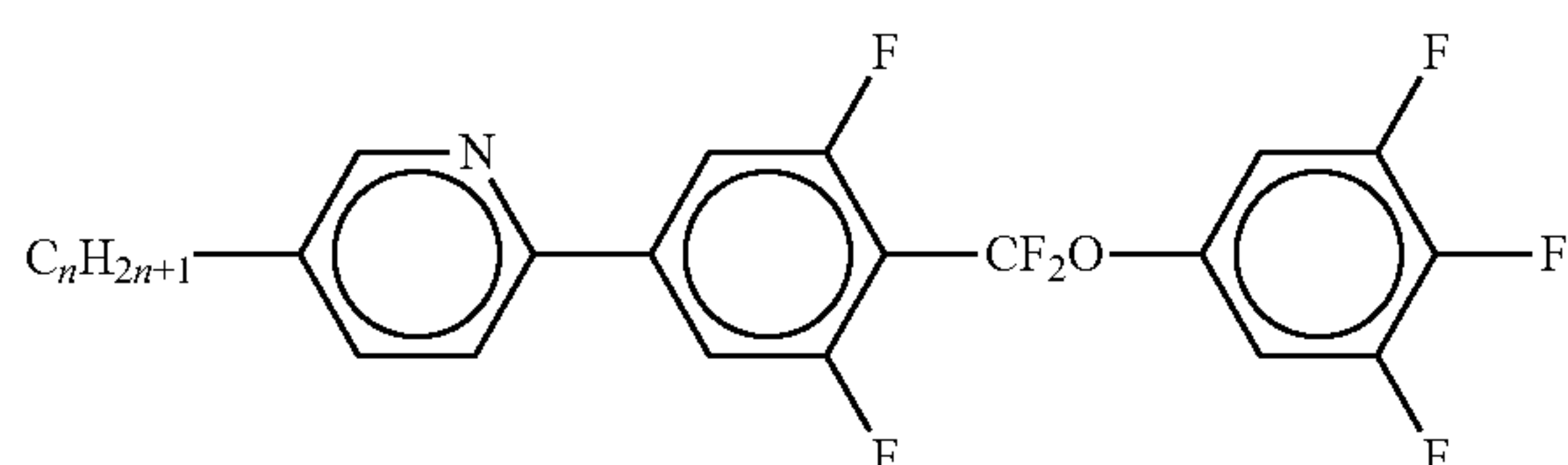
NUQU-n-F
