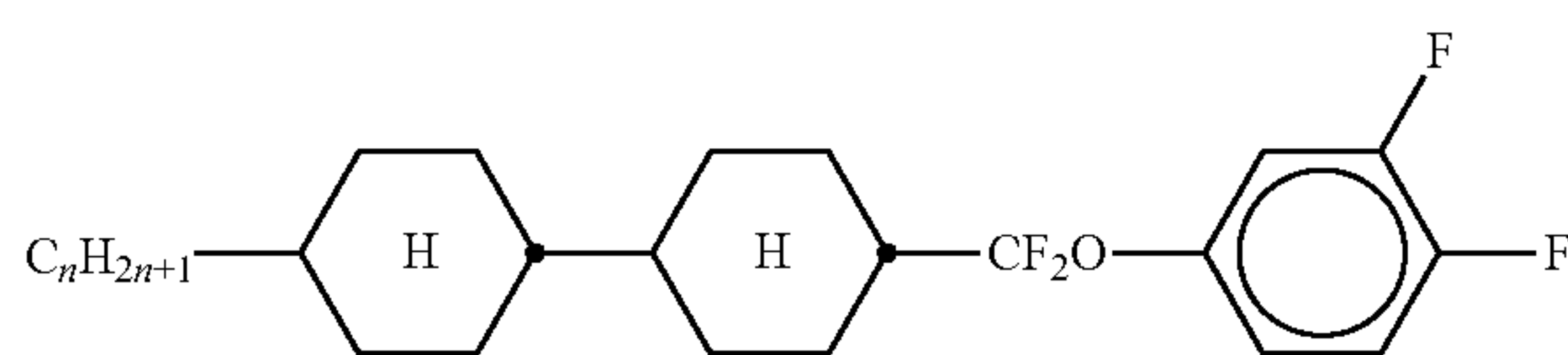
CCQG-n-F
