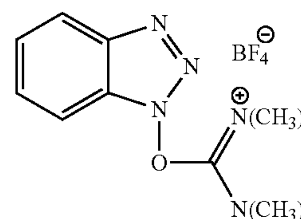
TBTU
