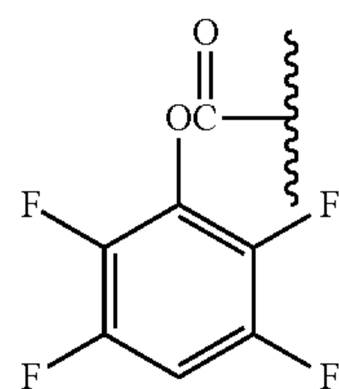
TFP
