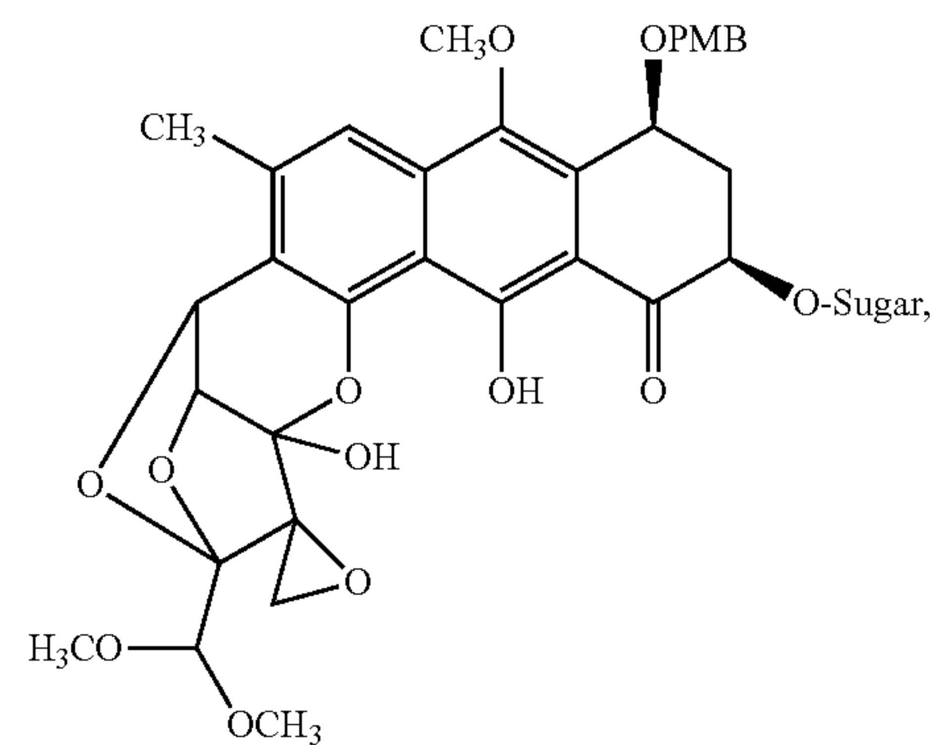
Sugar-Hemiketal 2
