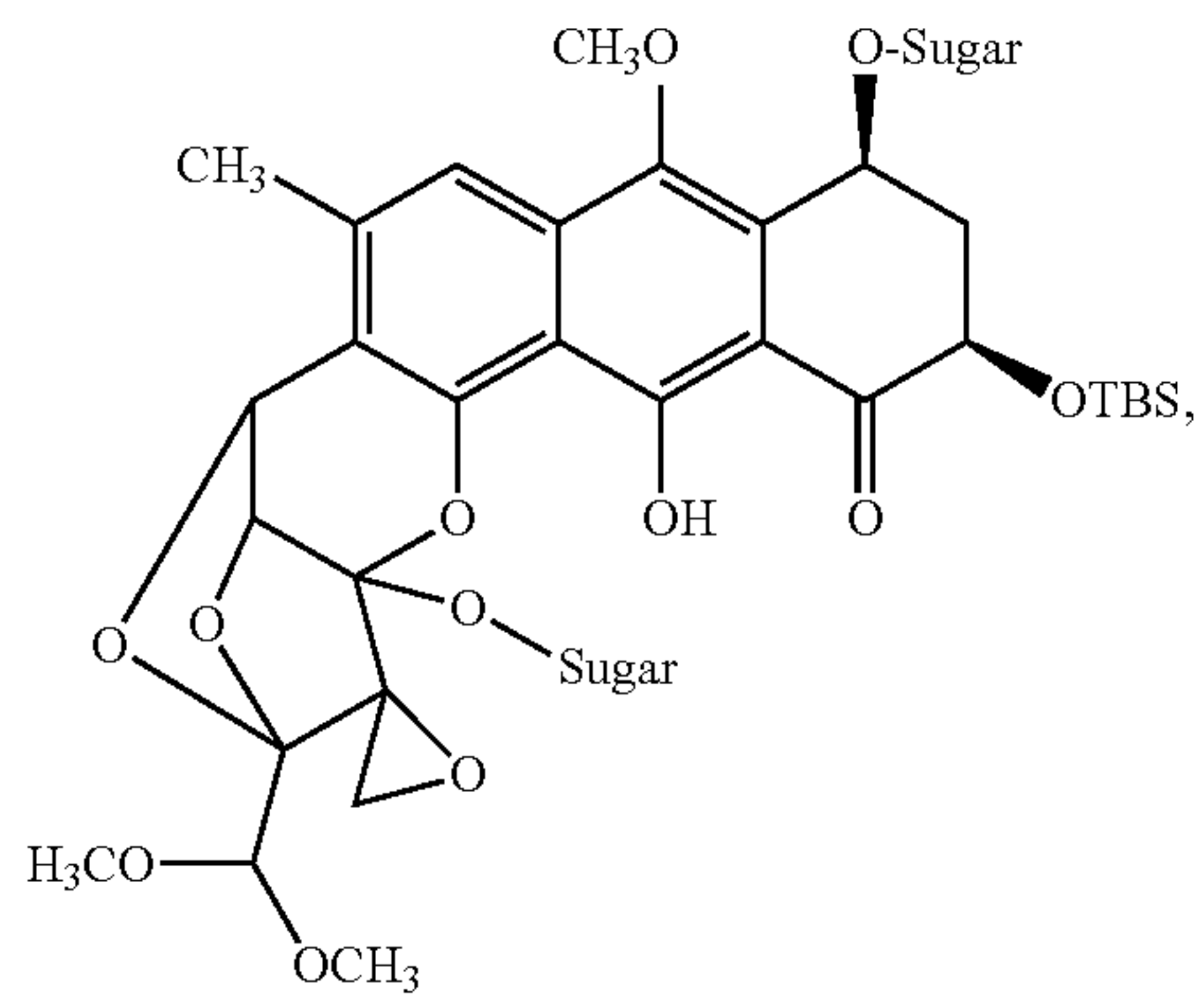
Sugar-Hemiketal 4
