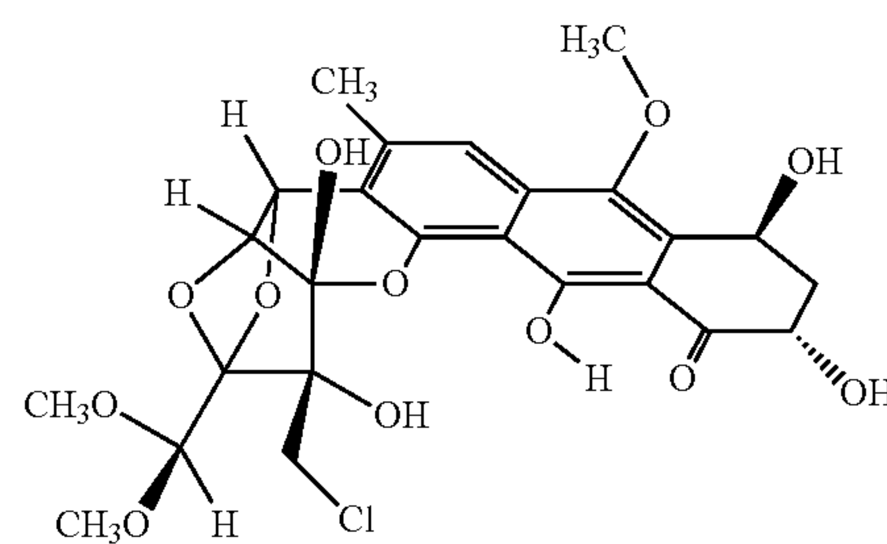
chlorohydrin
