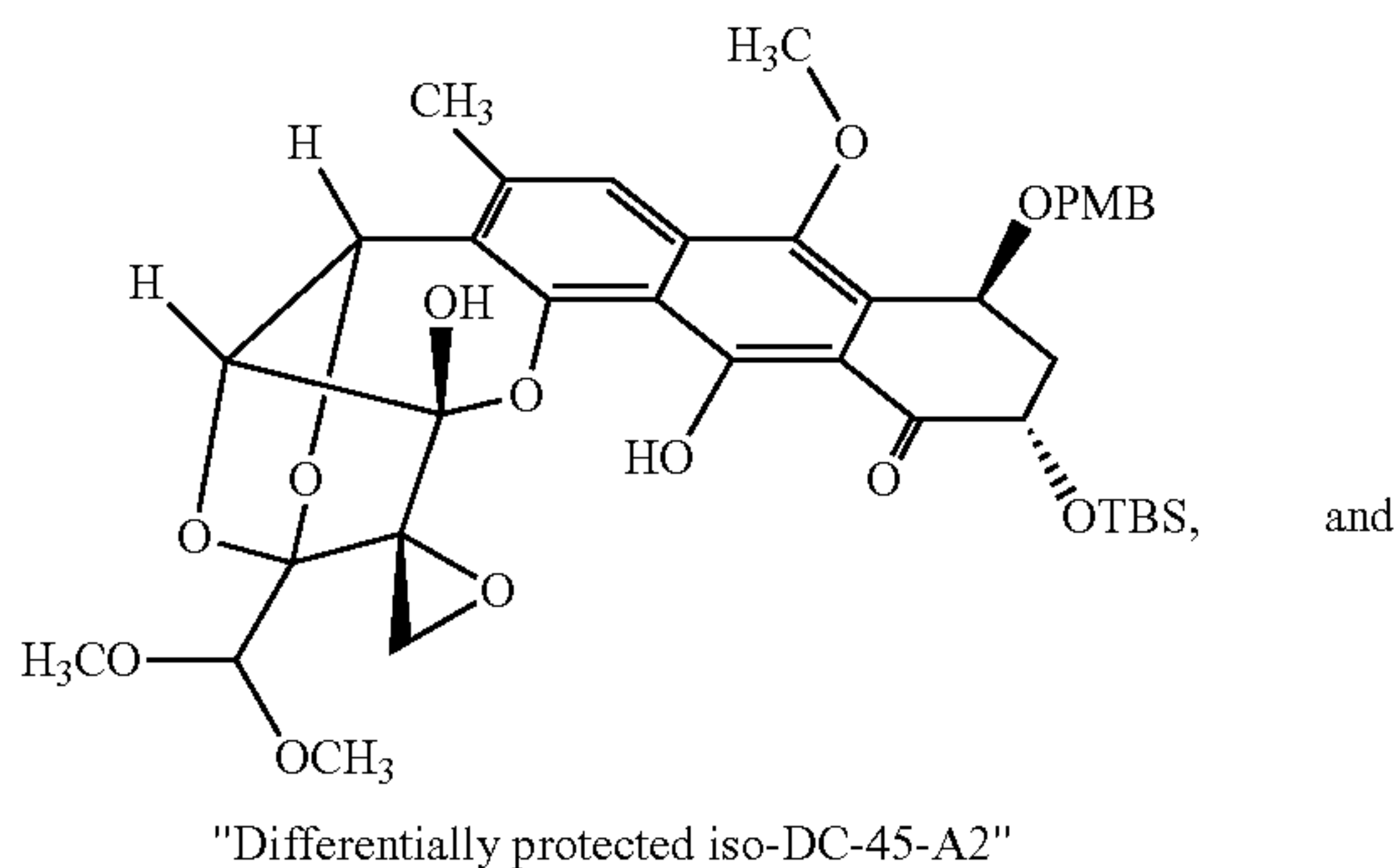
Endo 2 hemiketal
