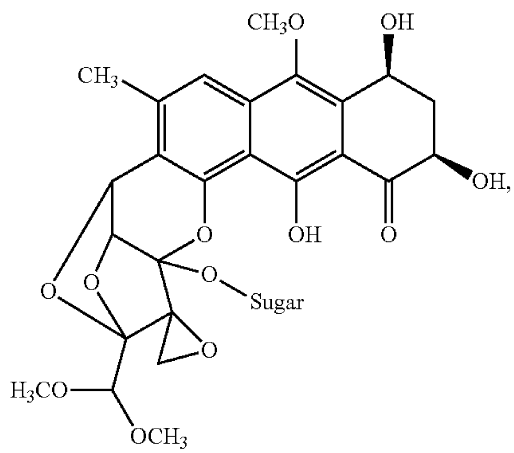
Sugar-Hemiketal 5
