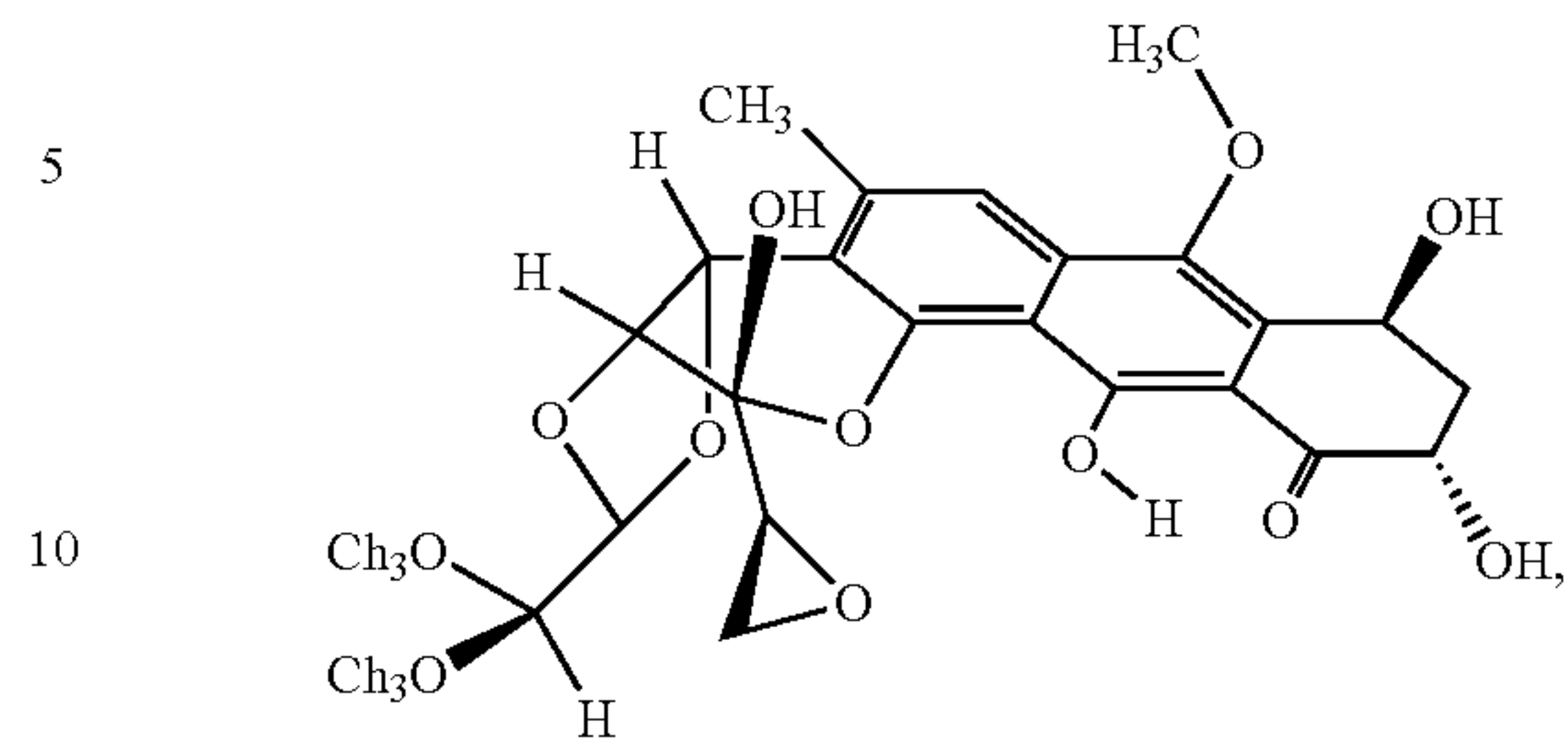
Iso-DC-45-A2
