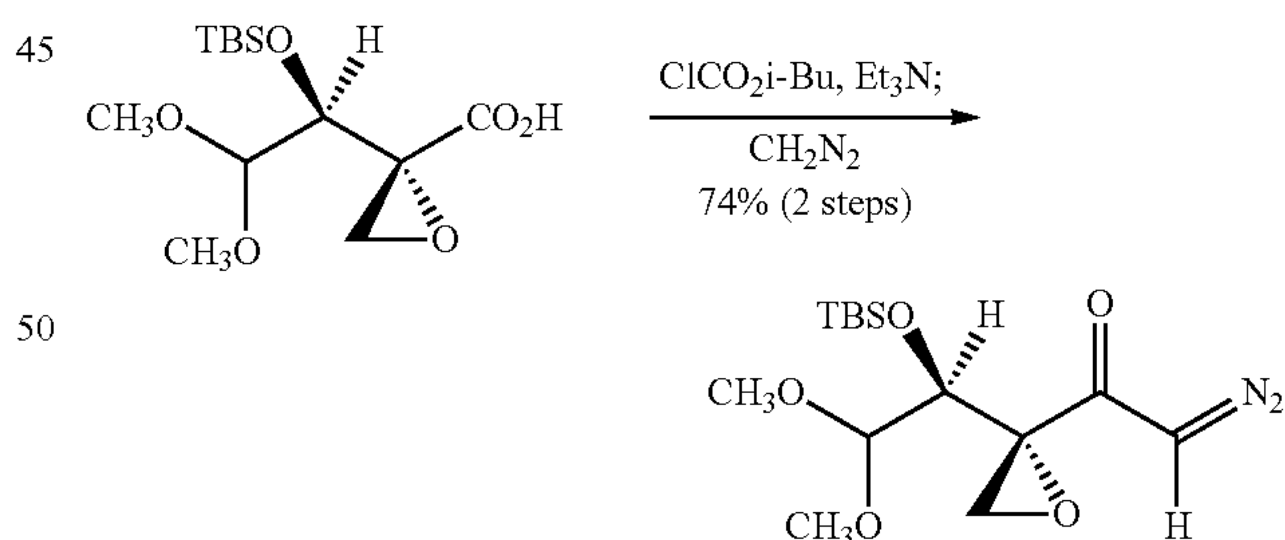
(2R,3S)-4-tert-Butyl dimethylsilyloxy-1-diazo-3-epoxy-5,5-dimethoxypenta-2-one
