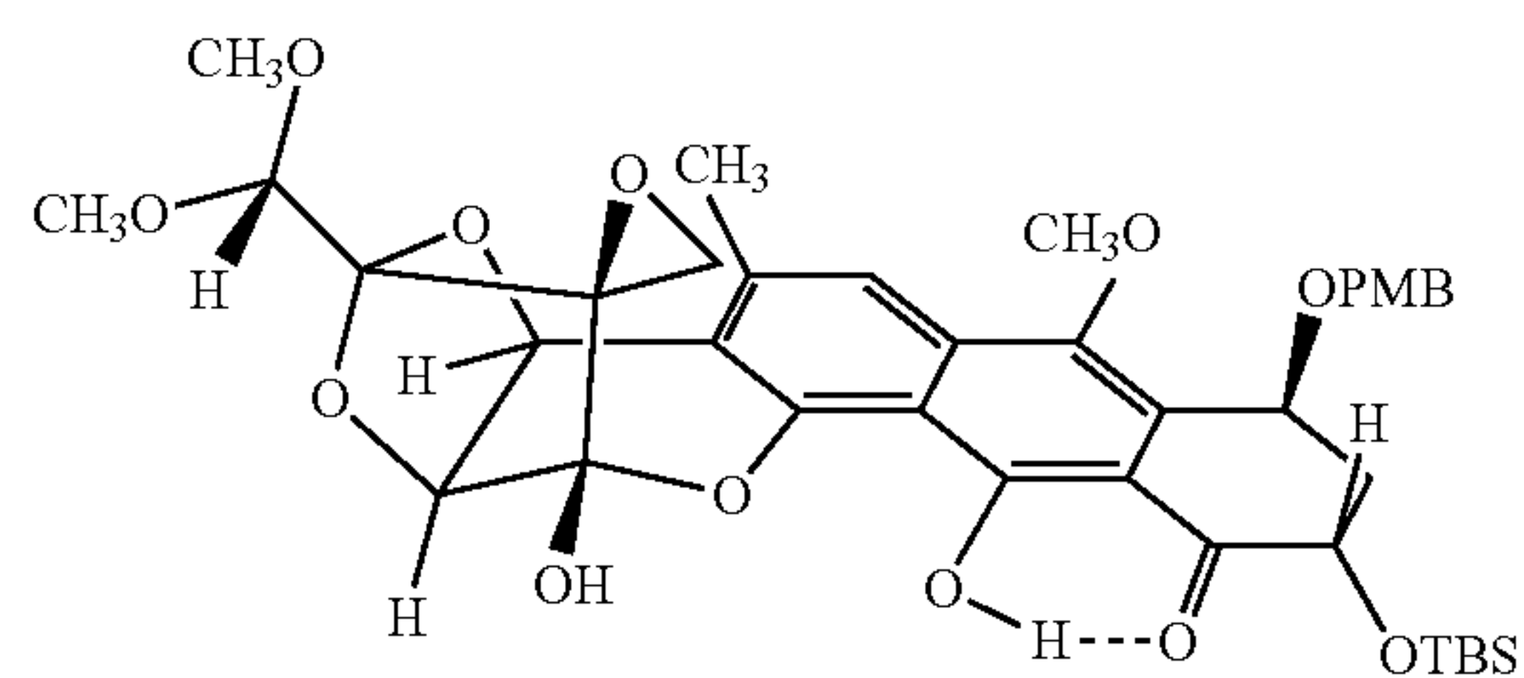
endo 2 hemiketal
