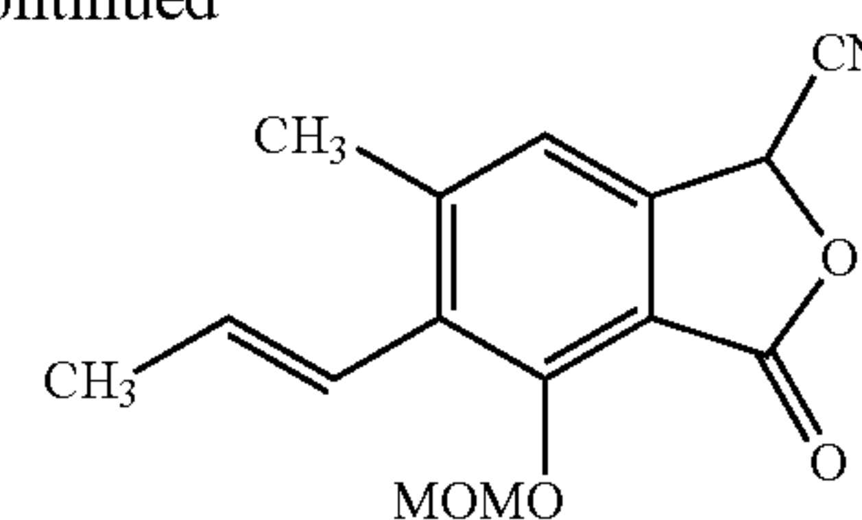
(E)-4-(Methoxymethoxy)-6-methyl-3-oxo-5-(prop-1-enyl)-1,3-dihydroisobenzofuran-1-carbonitrile
