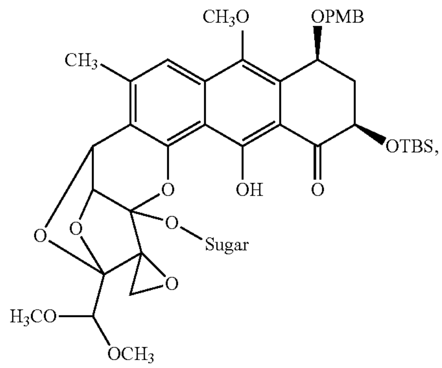
Sugar-Hemiketal 3
