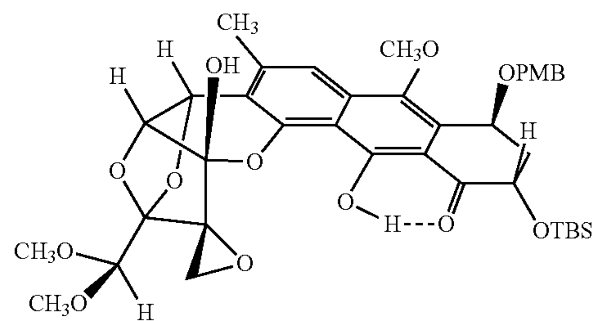
endo 1 hemiketal
