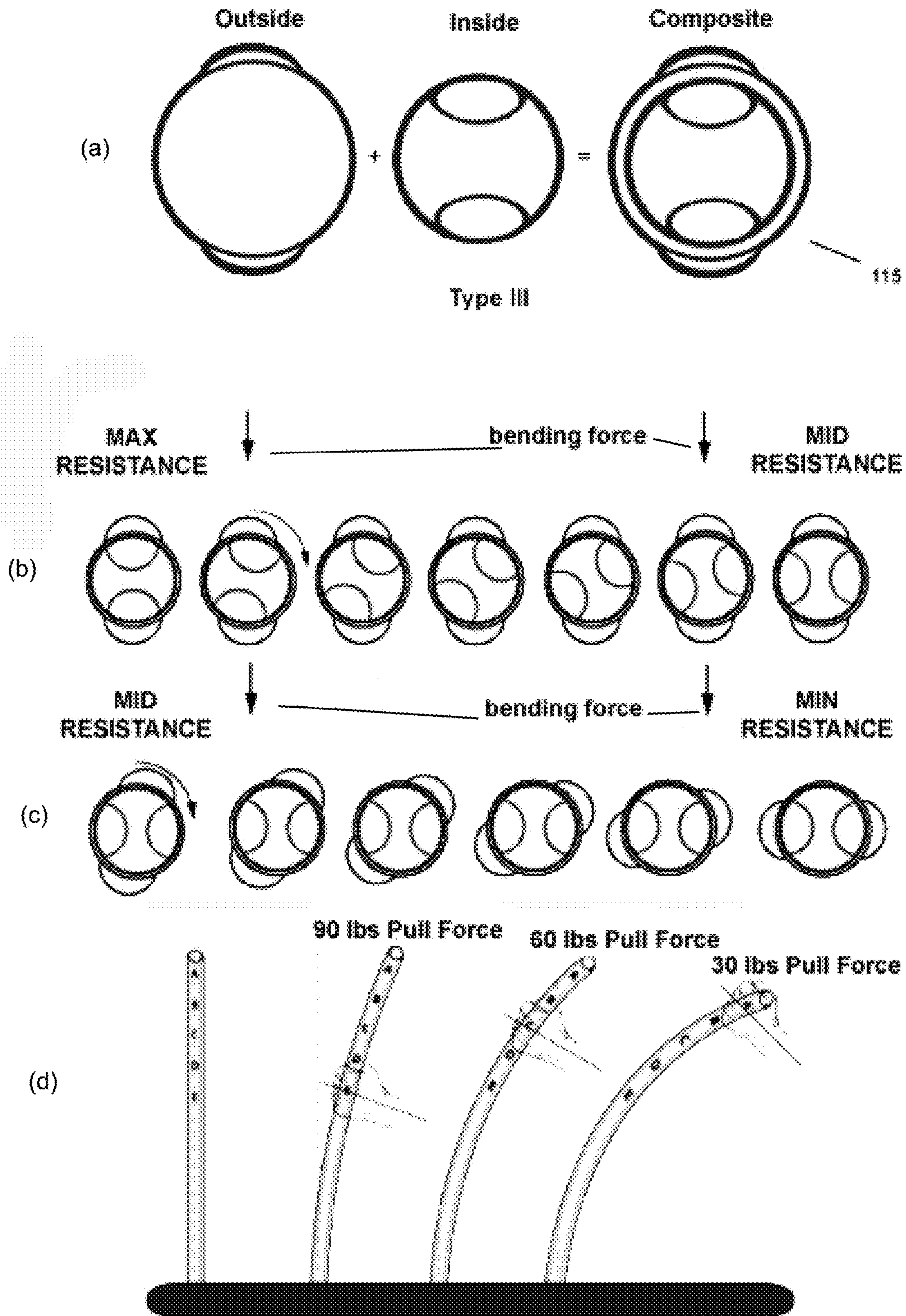
Fig. 1C
