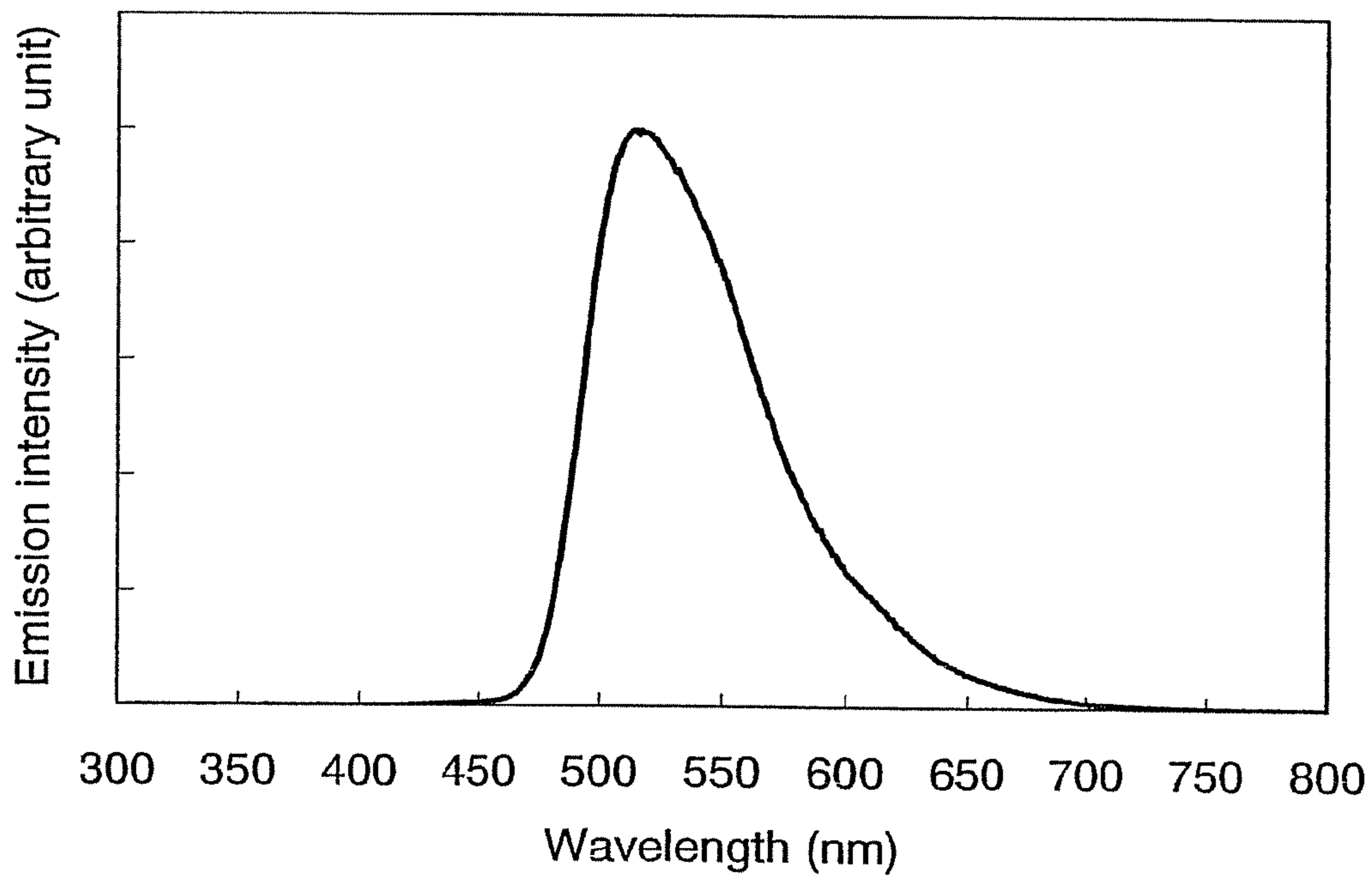
FIG. 14
