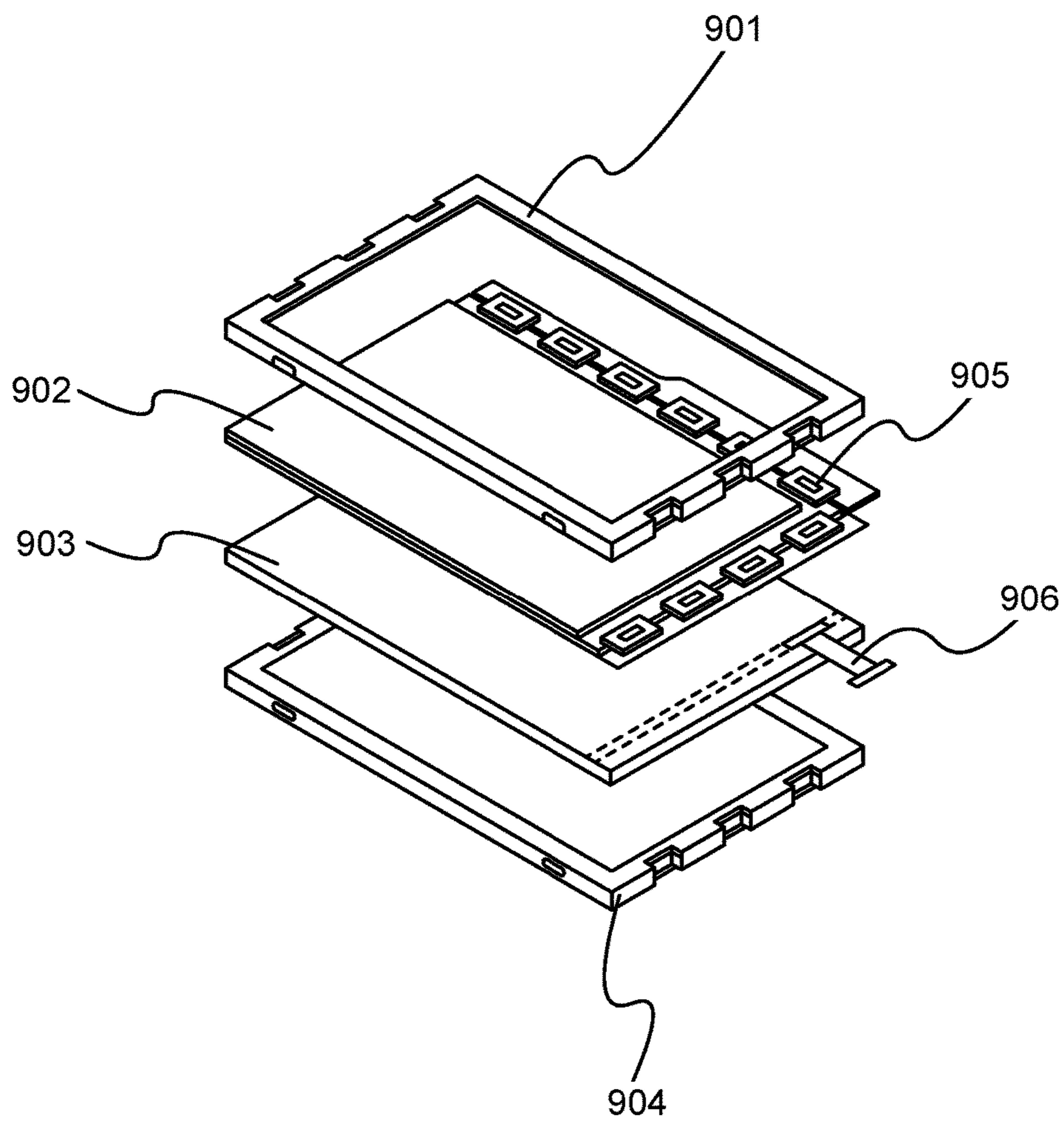
FIG. 7
