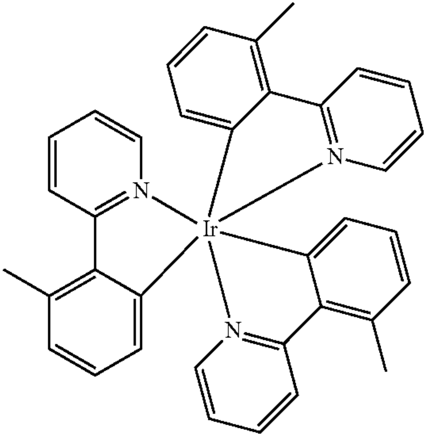
Dopant 1
