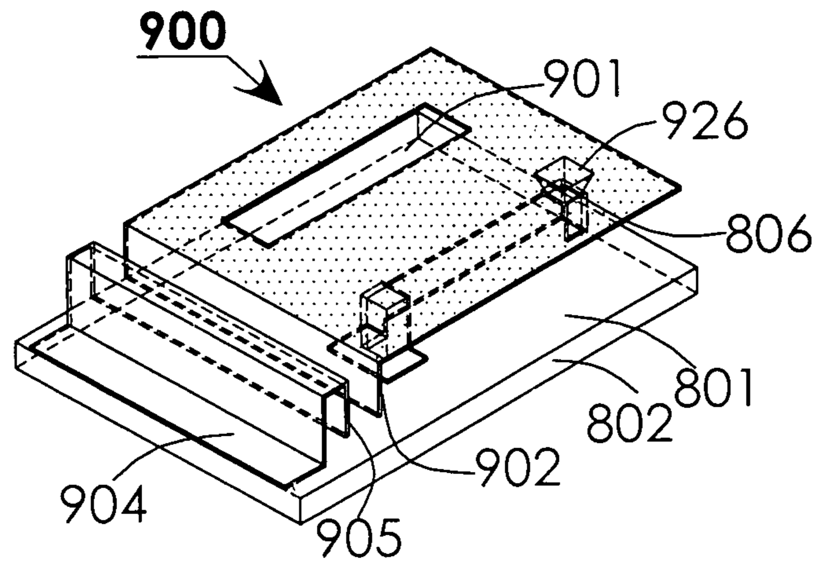
Fig. 9A
