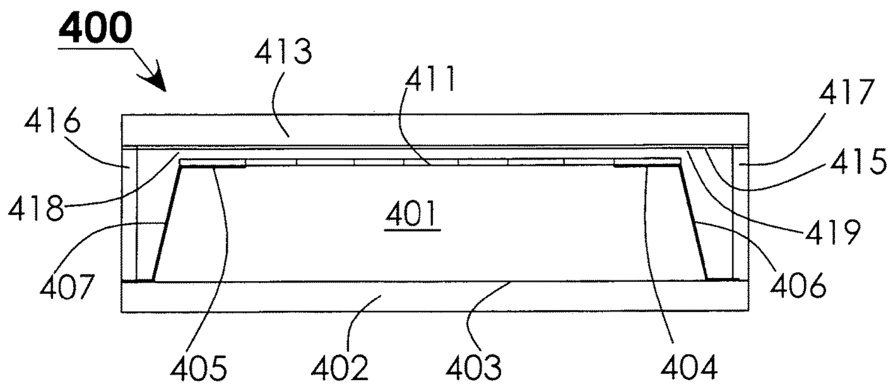
Fig. 4A
