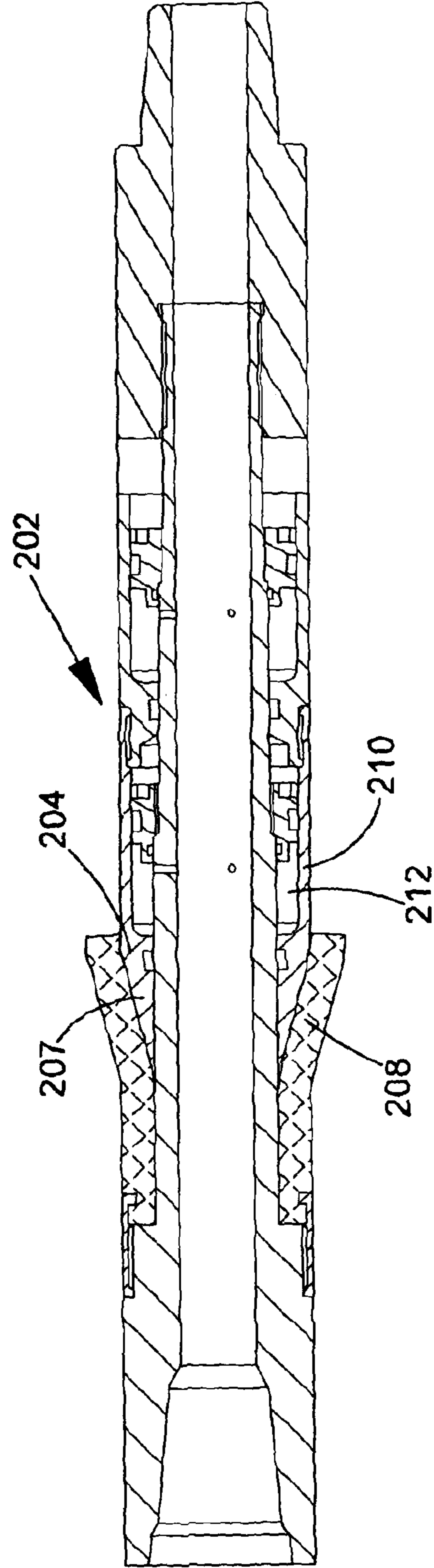
FIG. 20b
