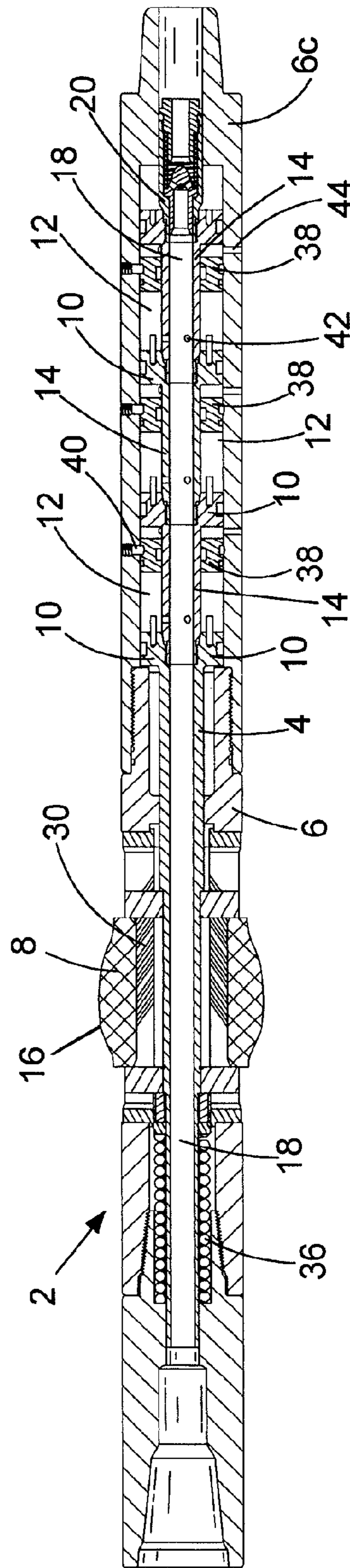
FIG.1b
