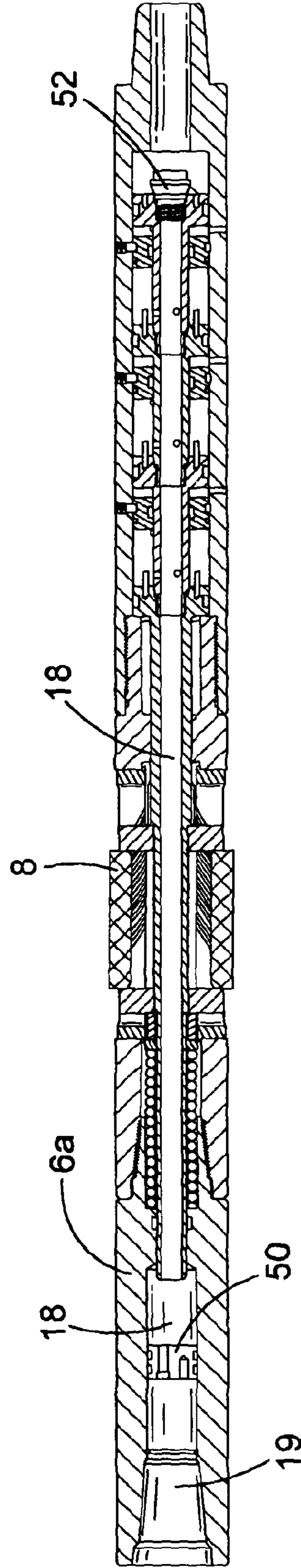
FIG. 7b
