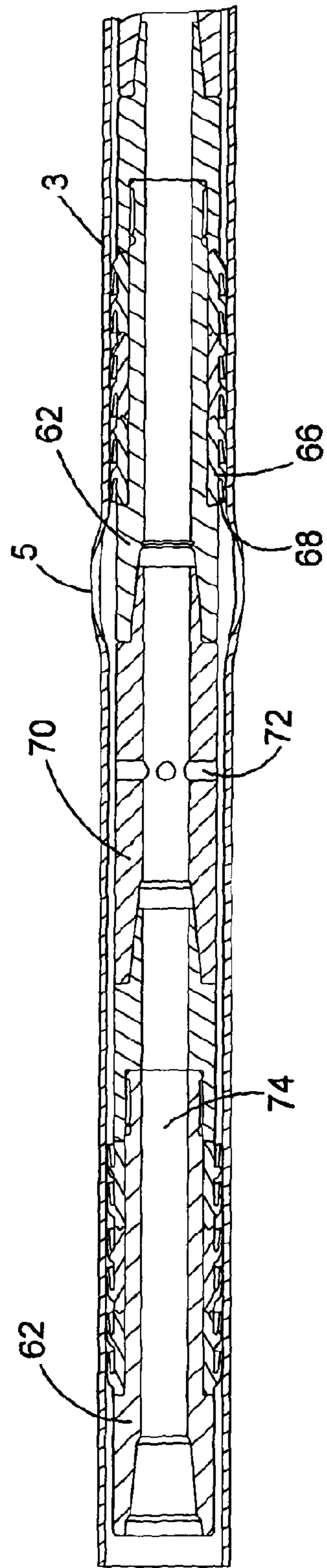
FIG. 13
