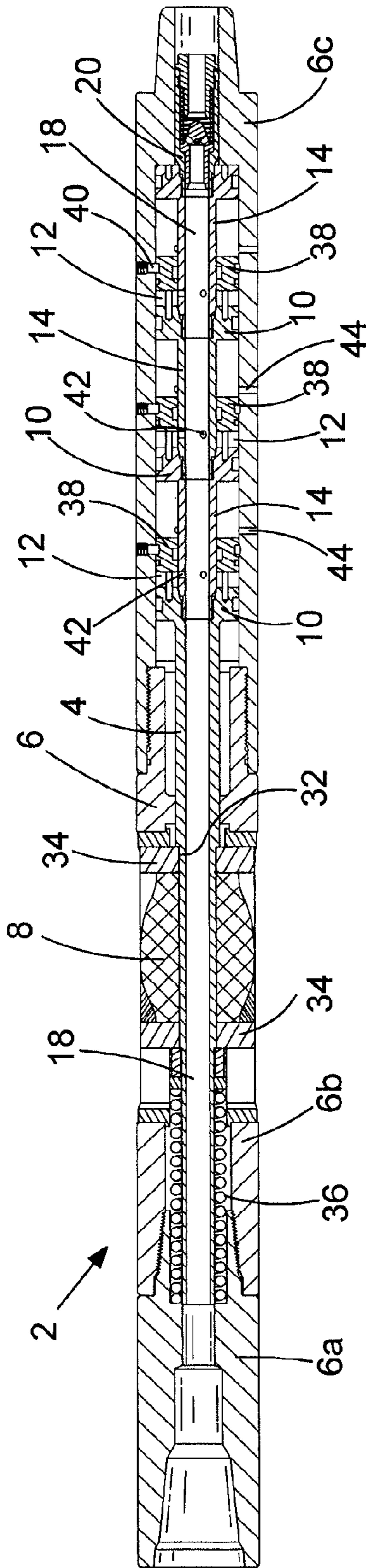
FIG.1a
