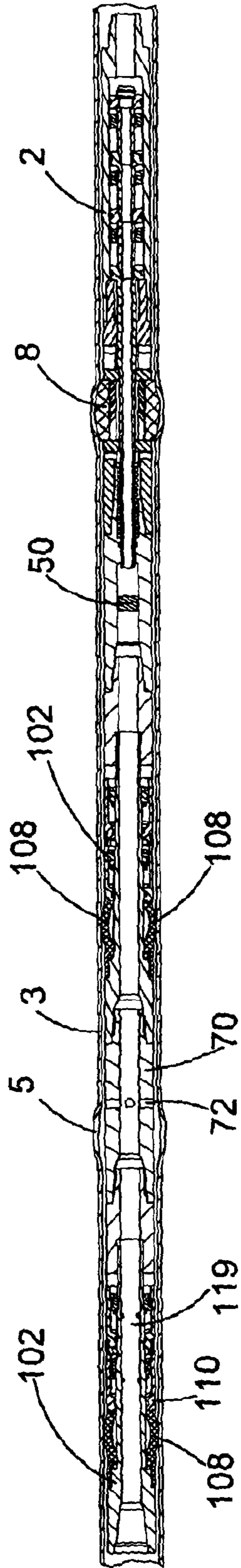
FIG. 17
