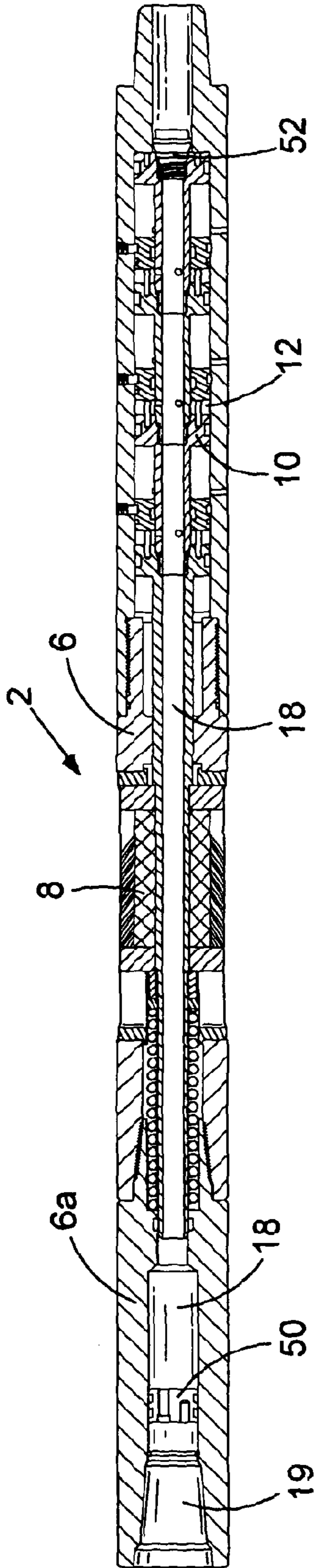
FIG. 7a
