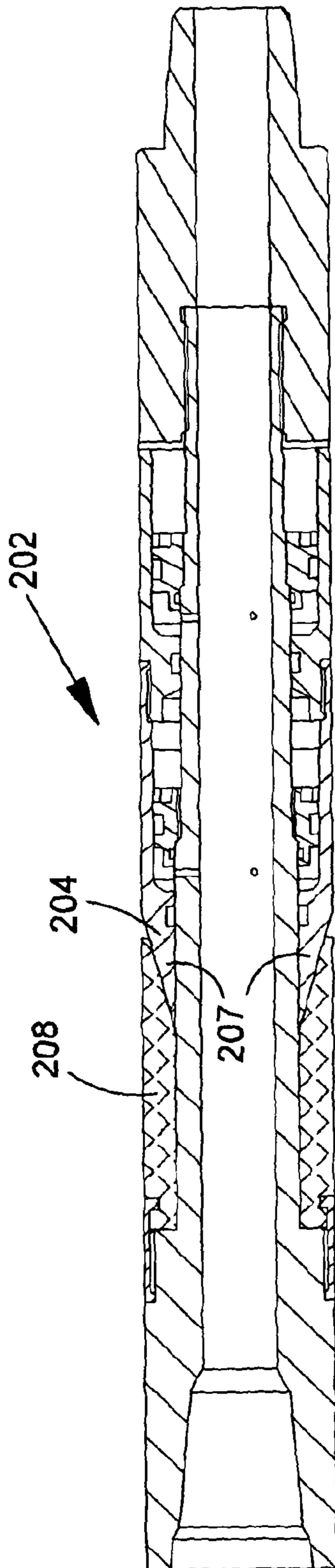
FIG. 20a
