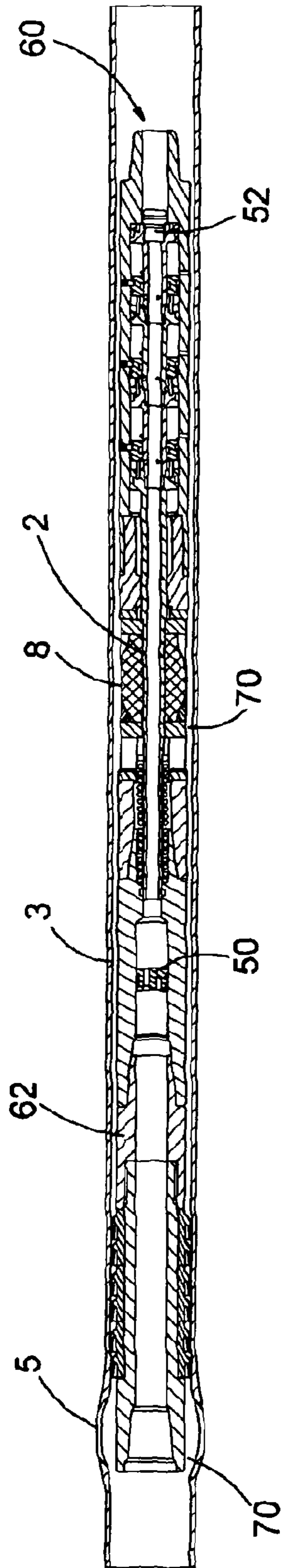
FIG. 10a
