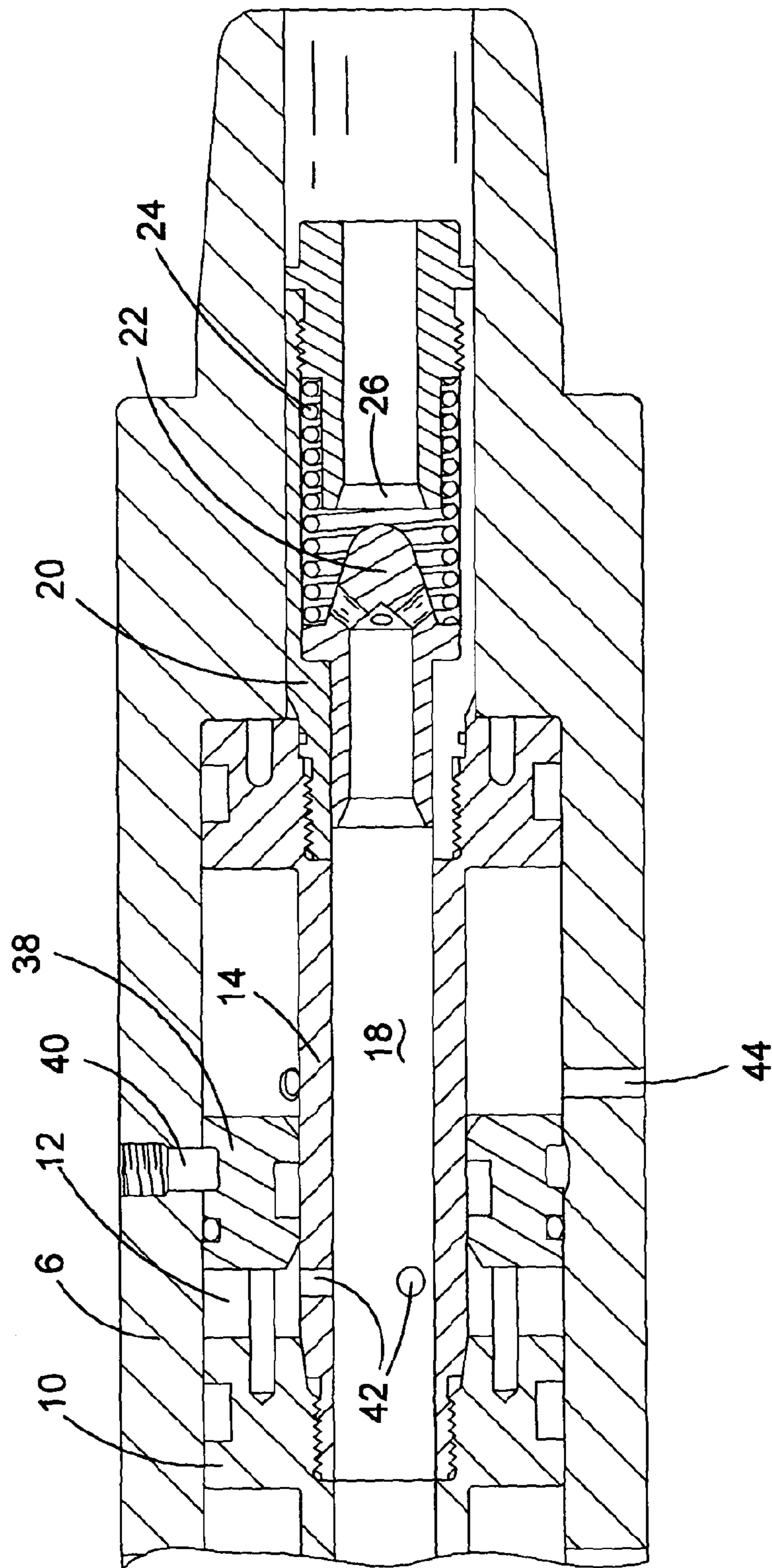
FIG. 5a
