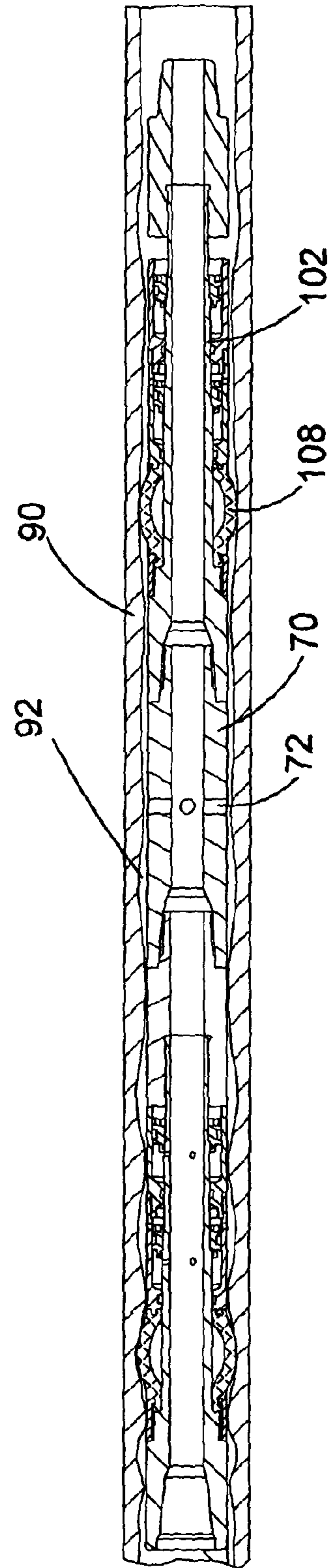
FIG. 19b
