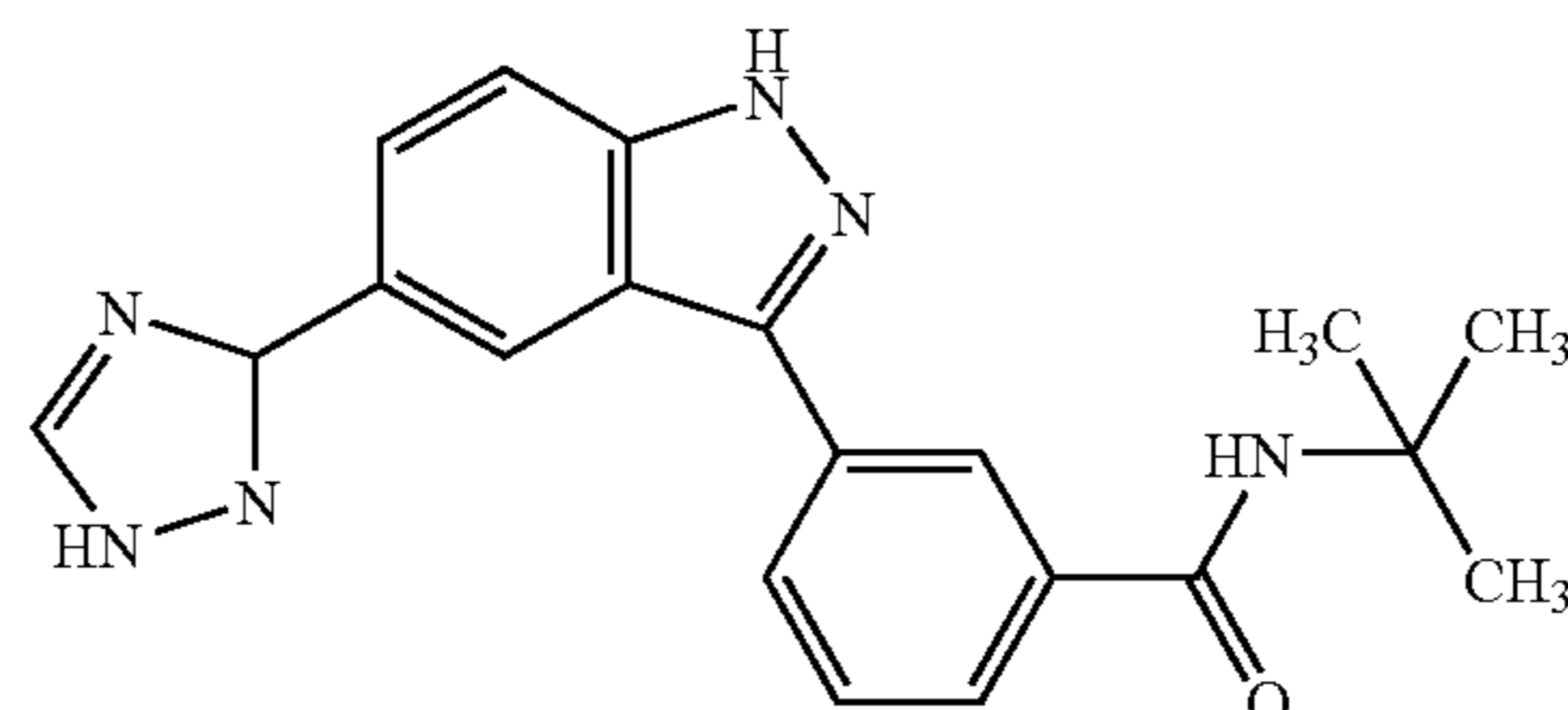
N-tert-Butyl-3-[5-(1H-[1,2,4]triazol-3-yl)-1H-indazol-3-yl]-benzamide
