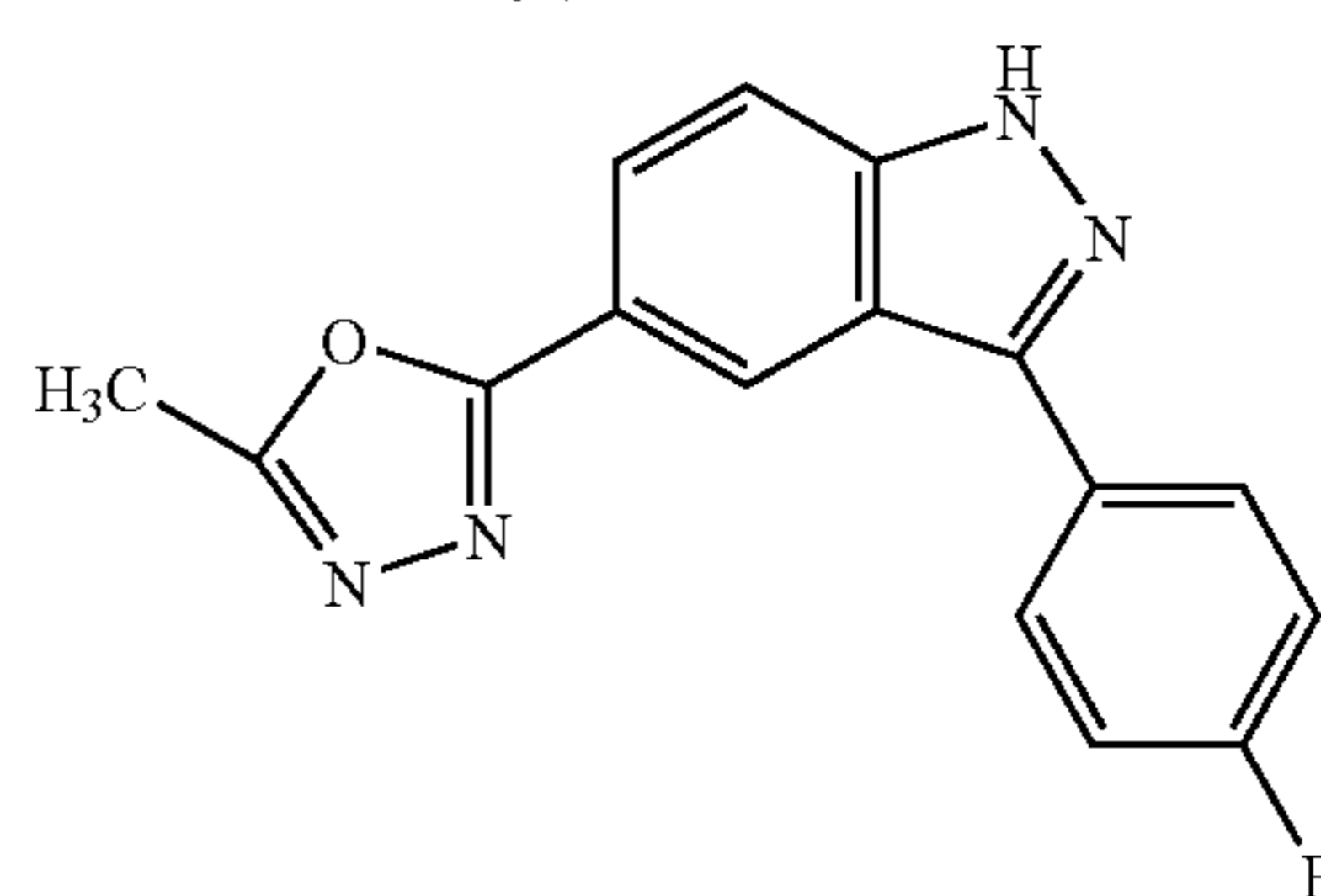
3-(4-Fluoro-phenyl)-5-(5-methyl-[1,3,4]oxadiazol-2-yl)-1H-indazole
