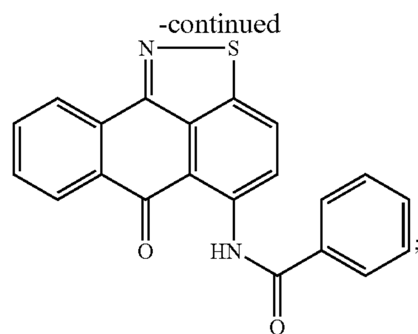
N-(6-Oxo-6H-anthra[9,1-cd]isothiazol-5-yl)-benzamide
