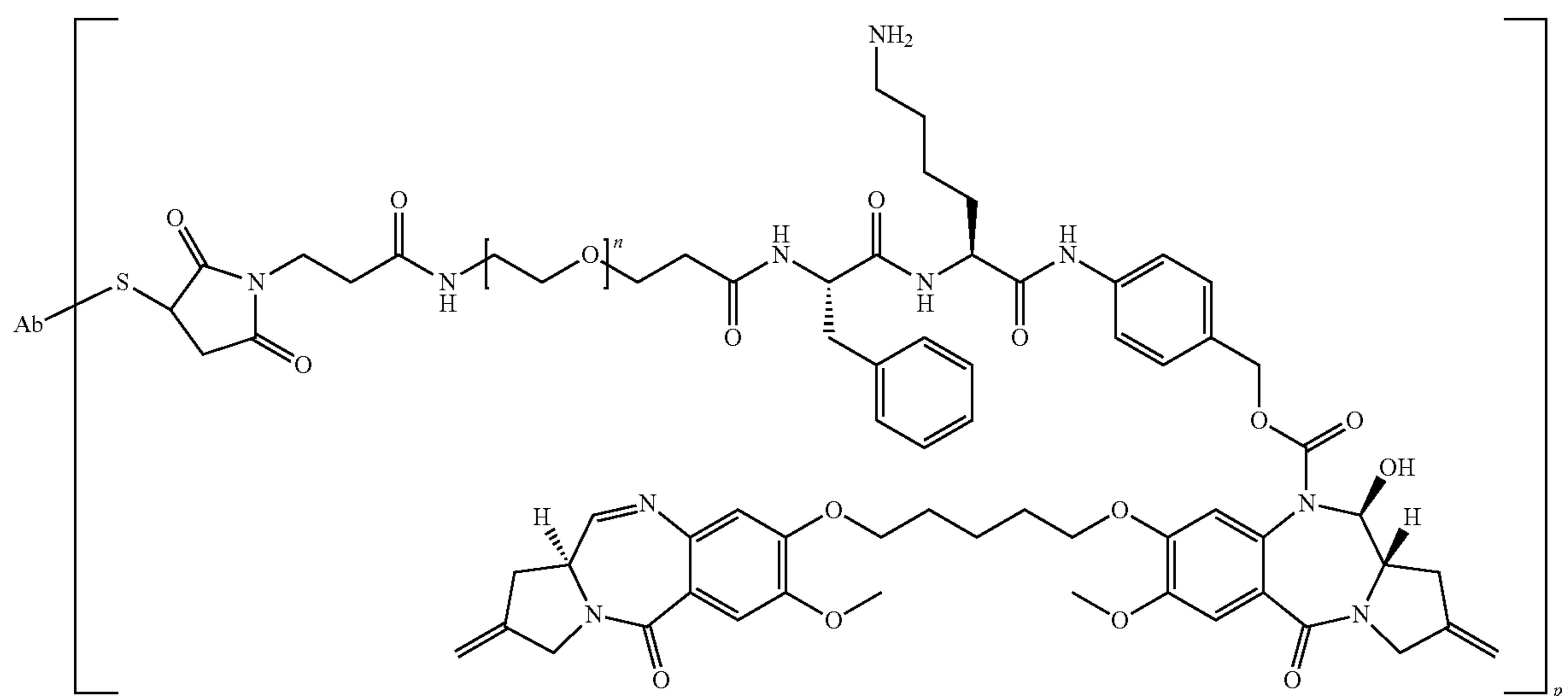
PBD dimer-Phe-Lys-PAB-Ab
