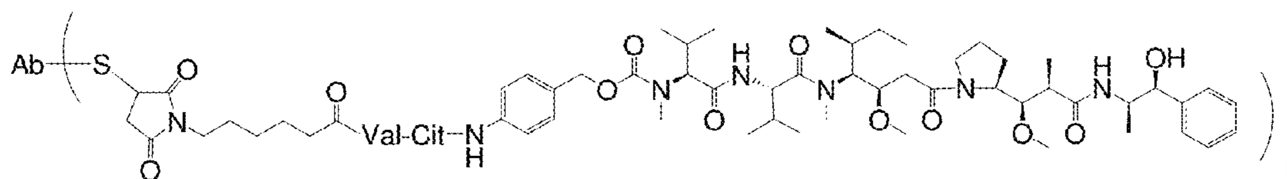
FIG. 15A Ab-MC-val-cit-PAB-MMAE
