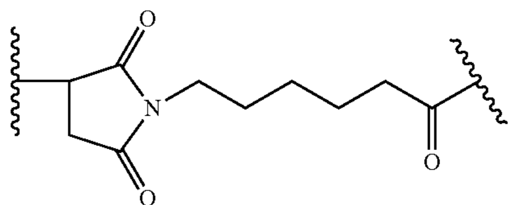
MC
