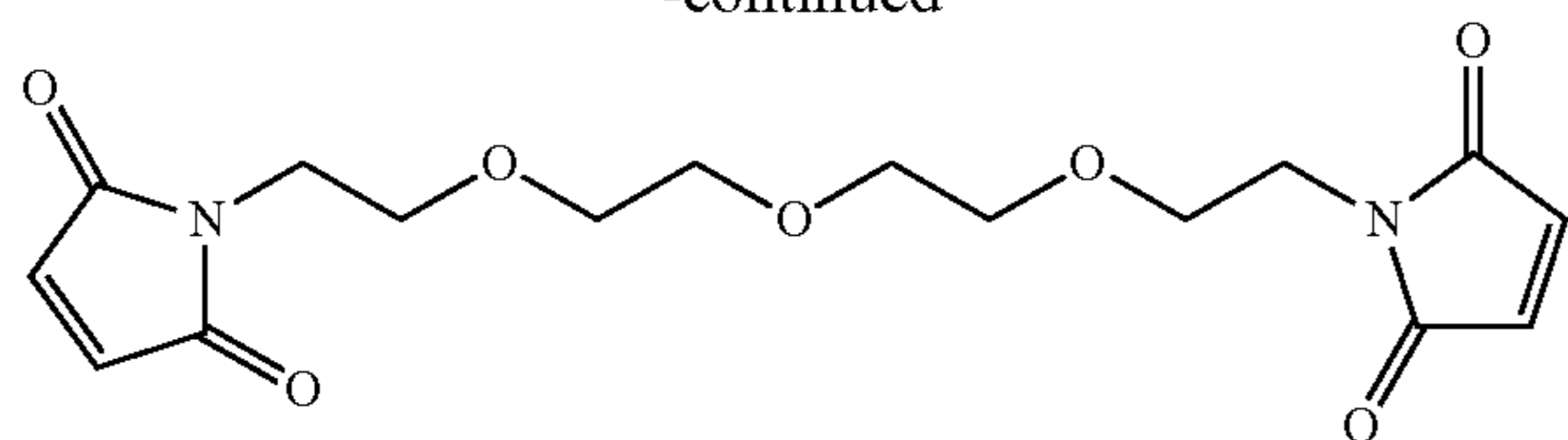
BM(PEG) 3
