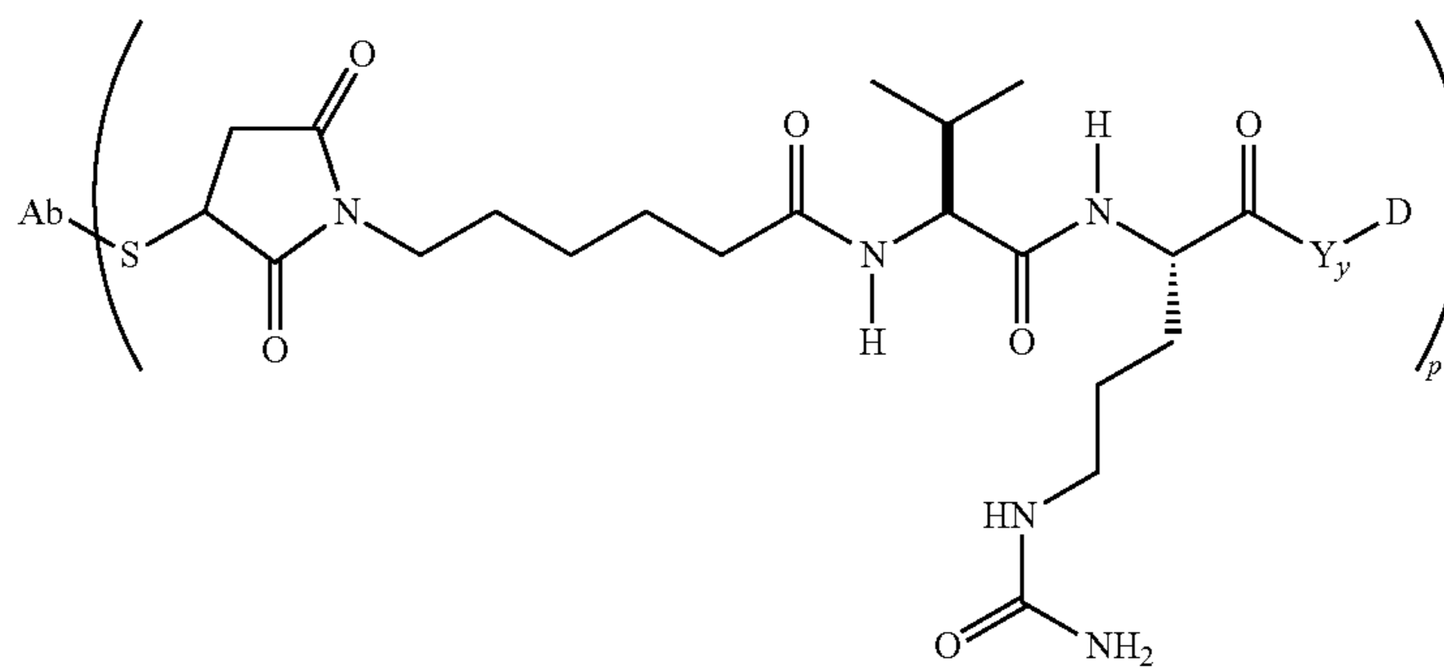
val-cit
