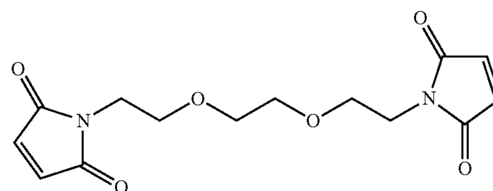
BM(PEG) 2
