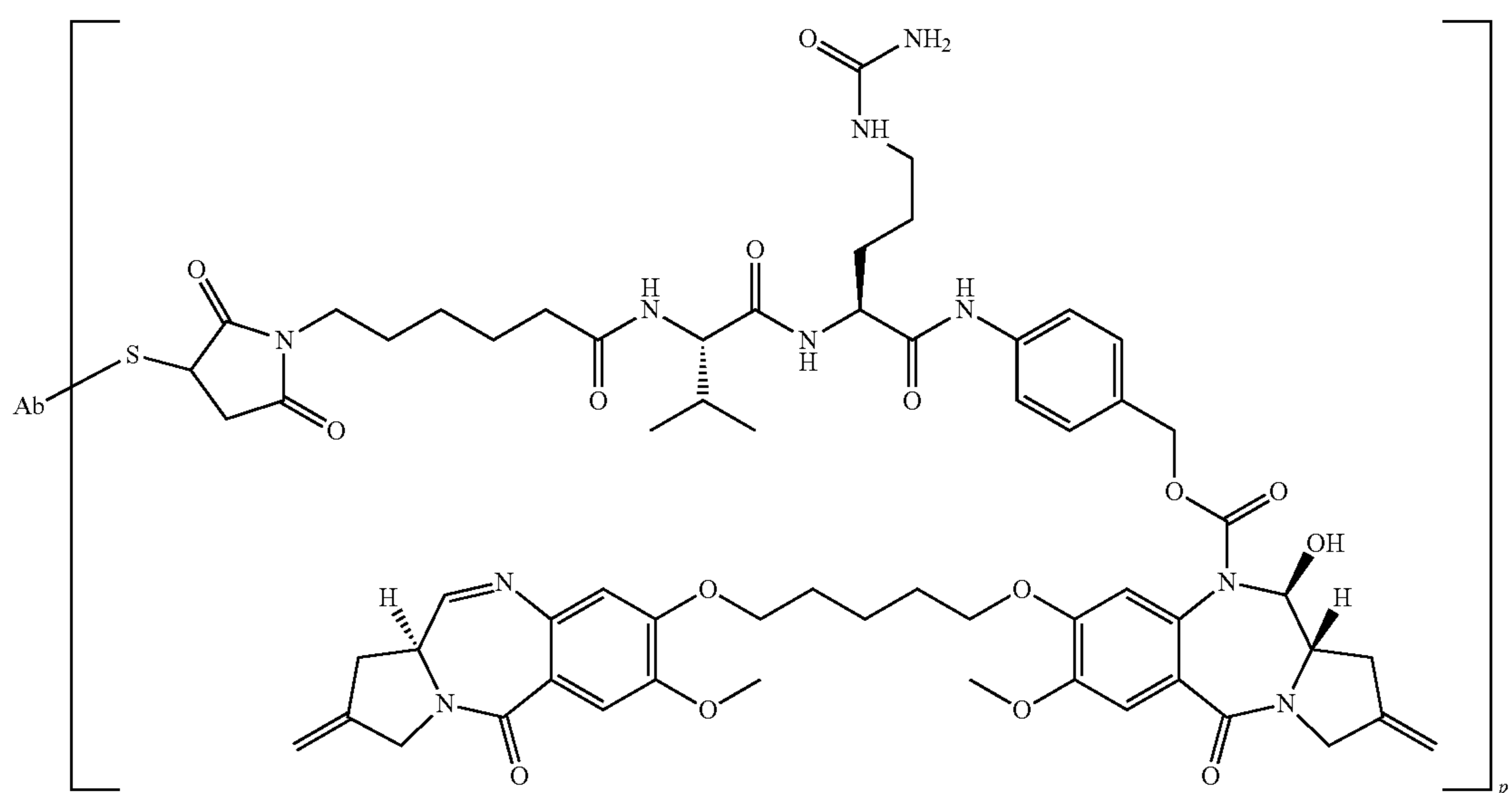
PBD dimer-val-cit-PAB-Ab
