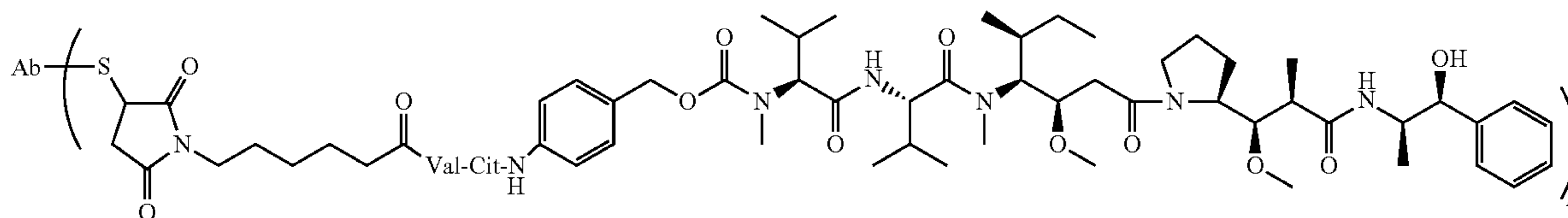
Ab-MC-vc-PAB-MMAE
