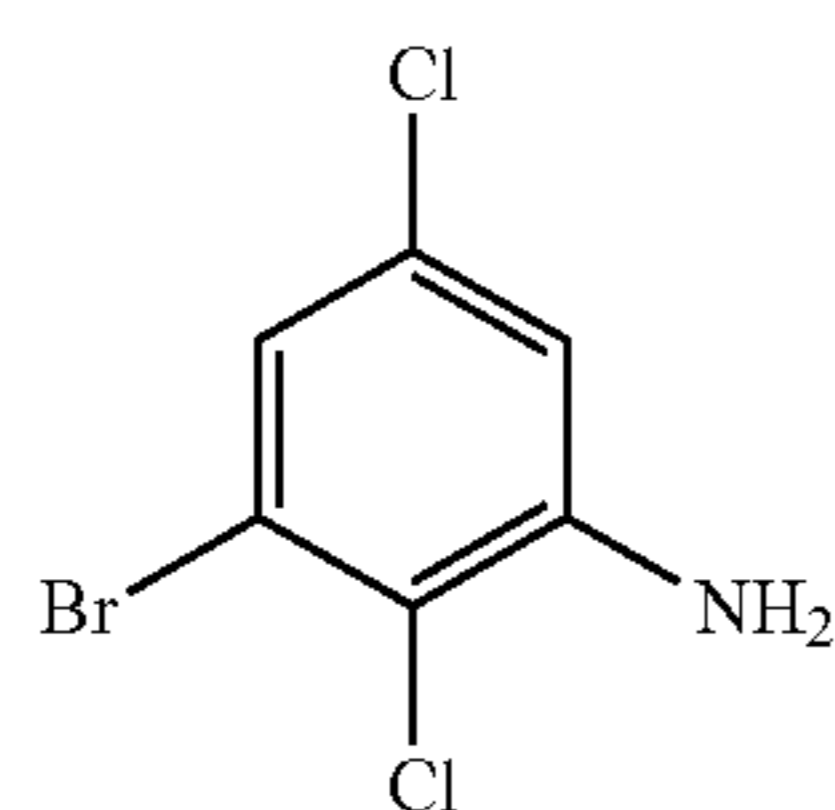
3-bromo-2,5-dichloroaniline
