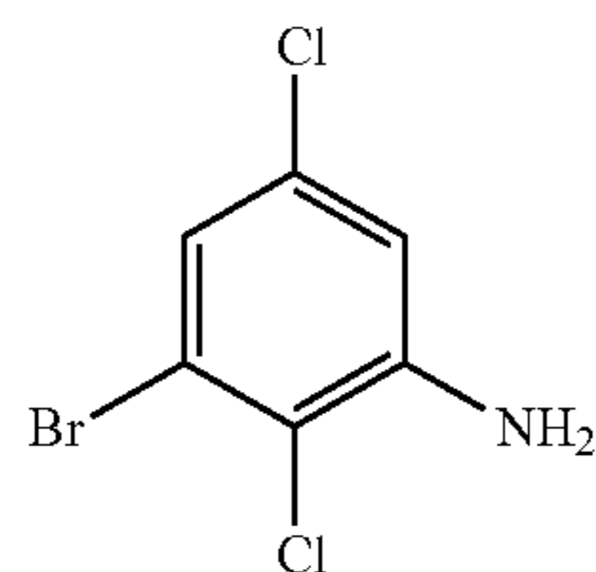
3-bromo-2,5-dichloroaniline
