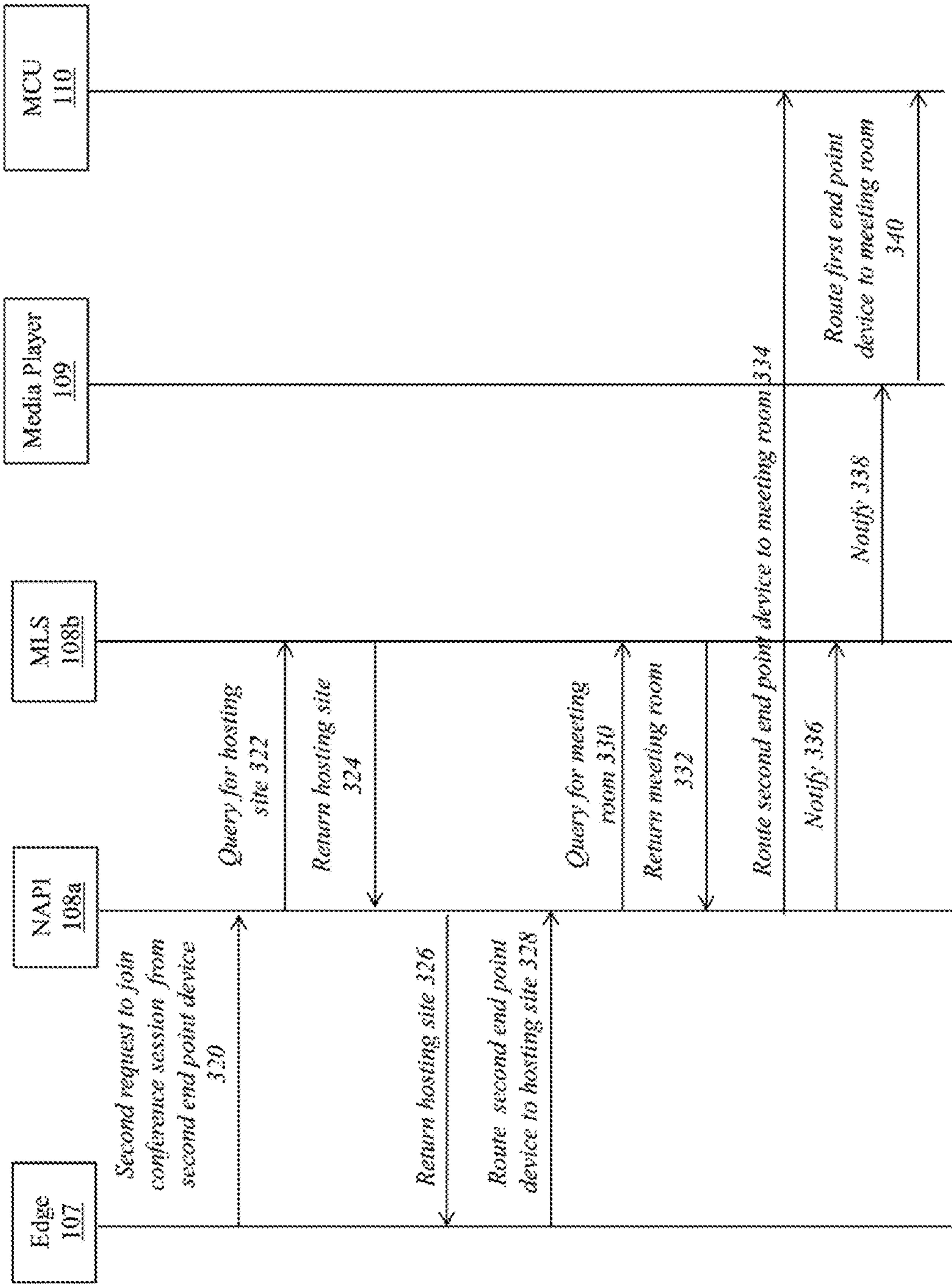
FIG. 3B
