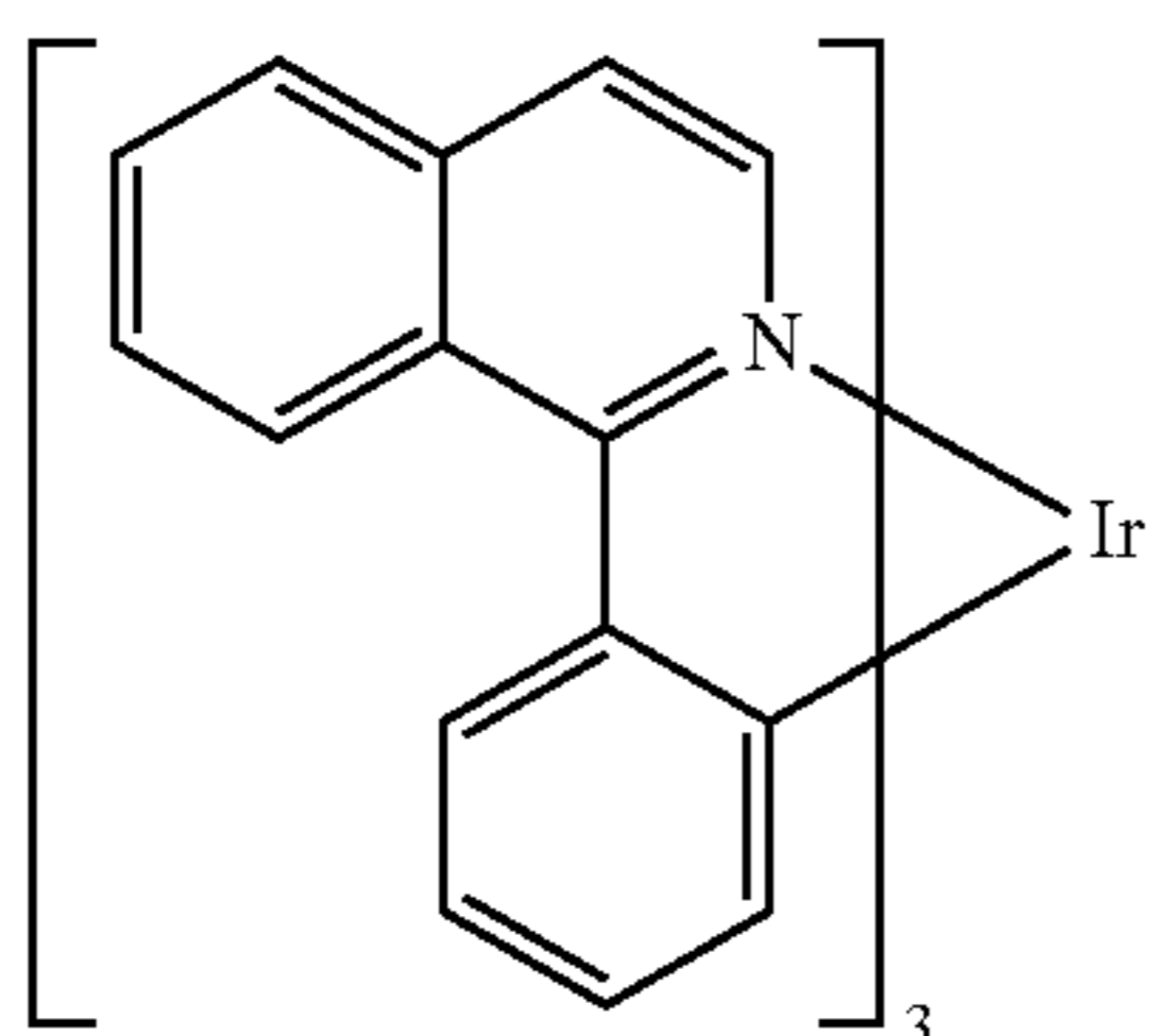
Ir(piq) 3
