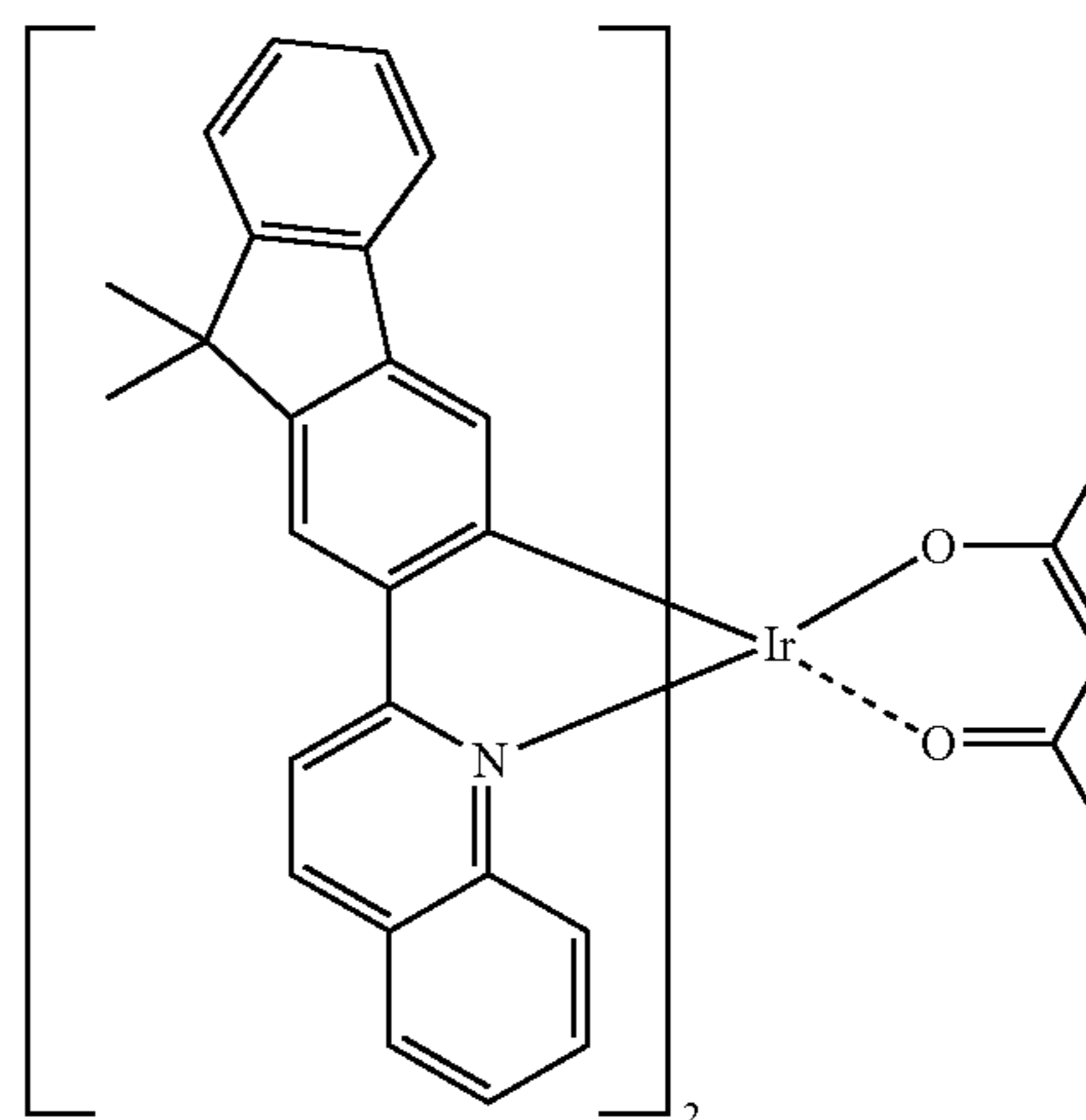
Ir(flq) 2 (acac)
