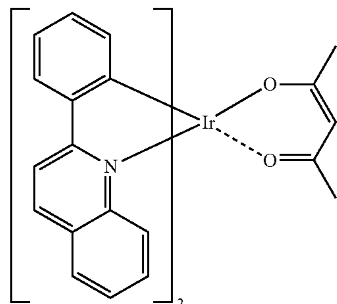
Ir(pq) 2 (acac)
