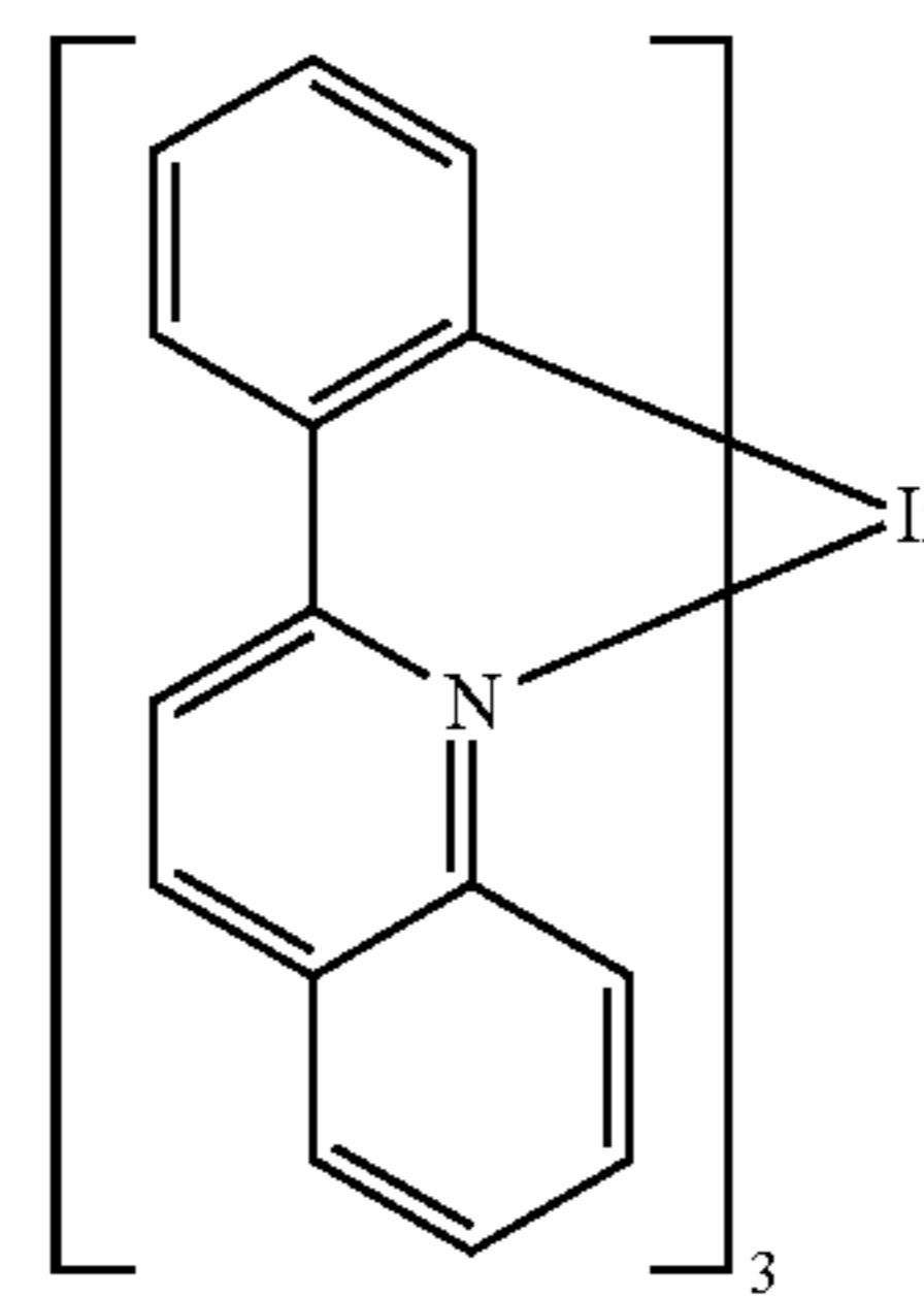
IR(2-phq) 3
