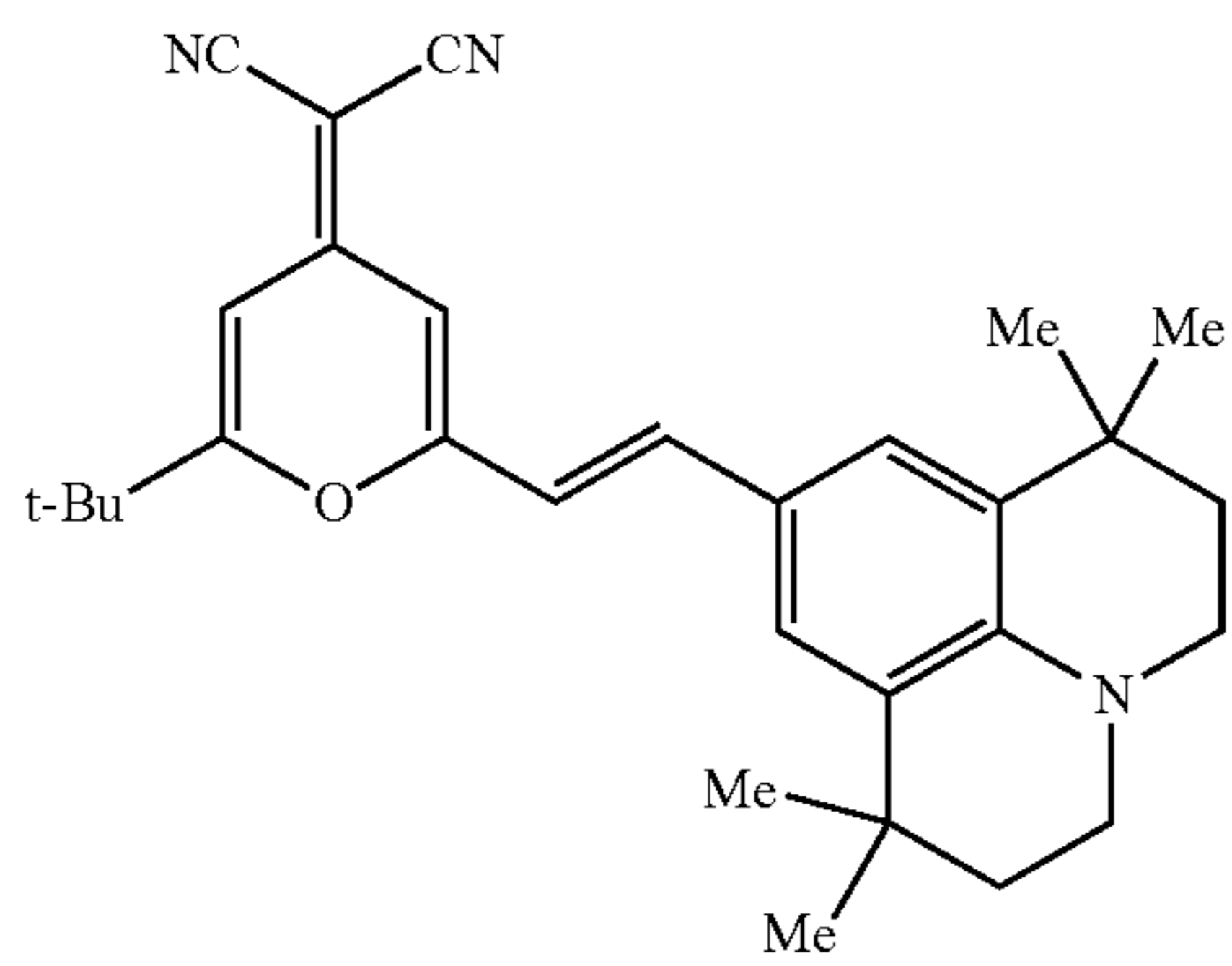
DCJTb
