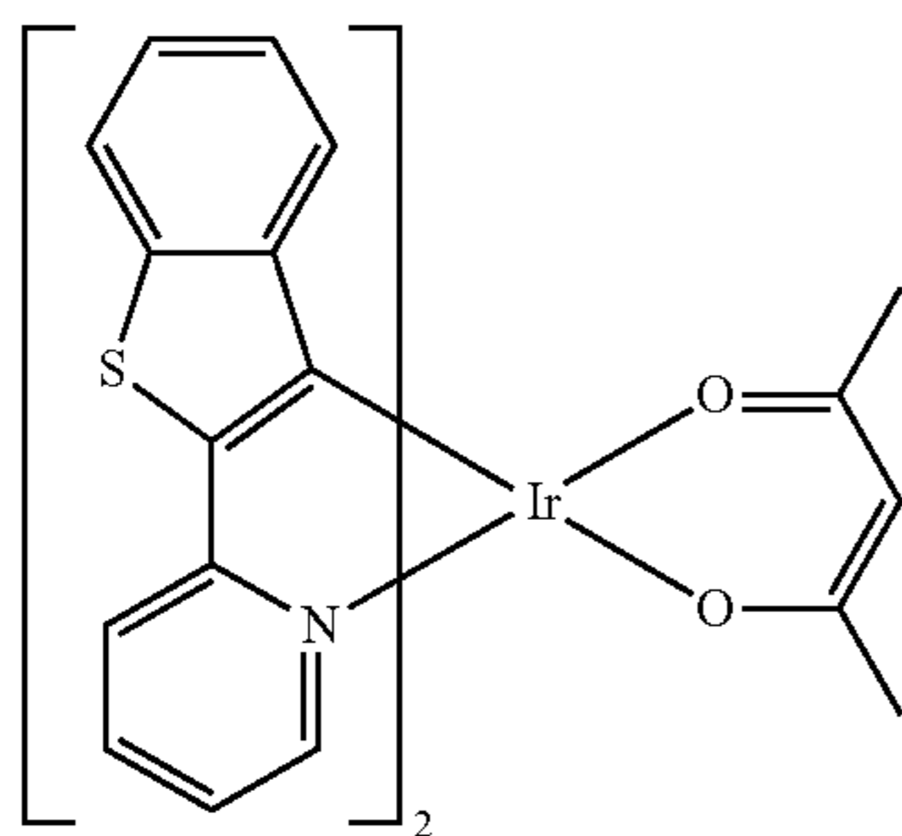
Btp 2 Ir(acac)
