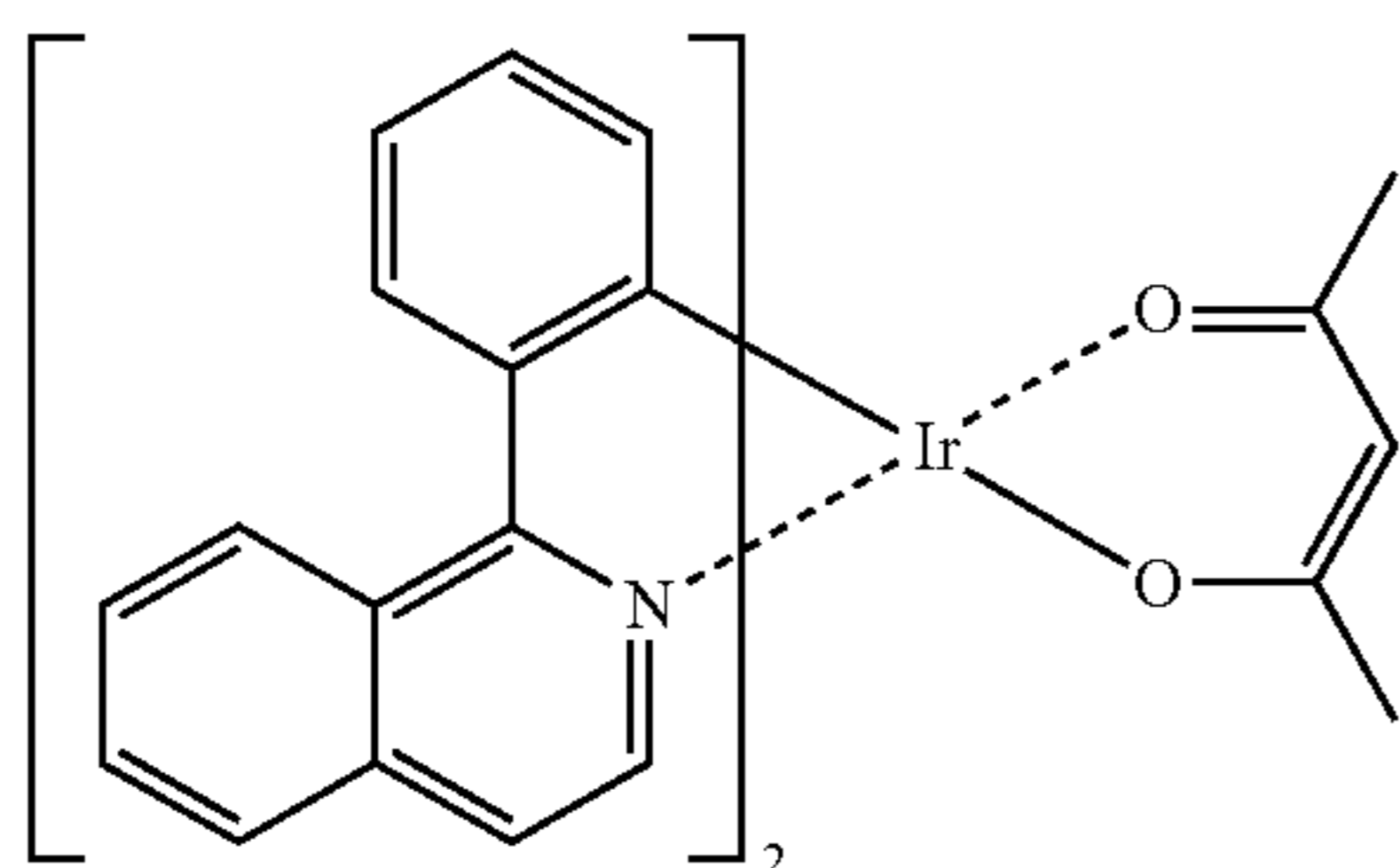
Btp 2 Ir(acac)
