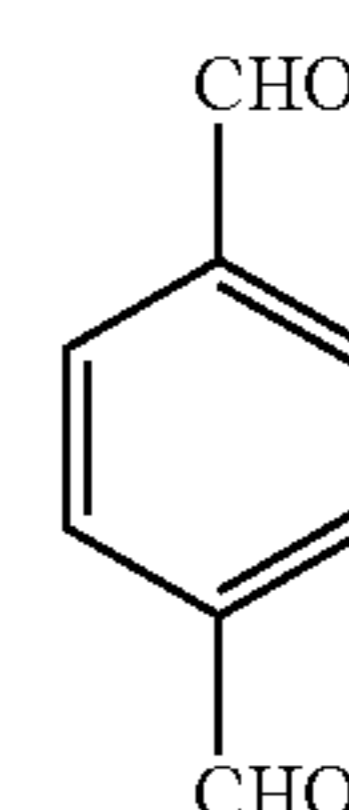
p-Benzylaldehyde
