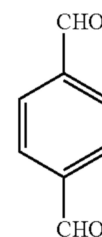
p-Benzylaldehyde
