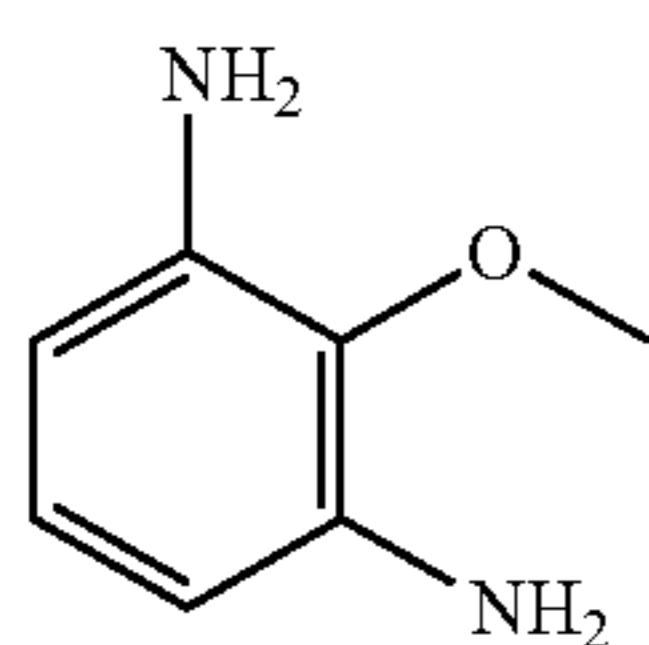
2-methoxybenzene- 1,3-diamine
