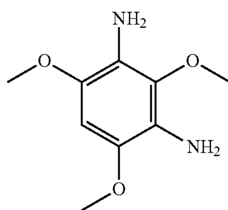
2,4,6-trimethoxybenzene- 1,3-diamine
