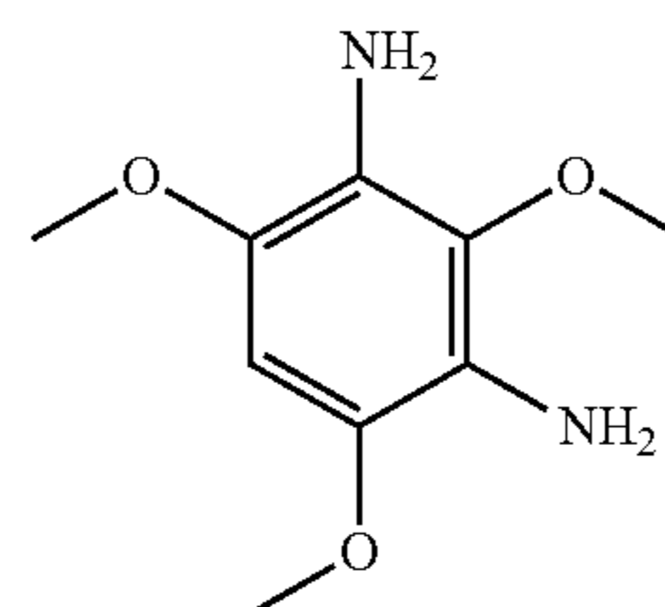
2,4,6-trimethoxybenzene-1,3-diamine
