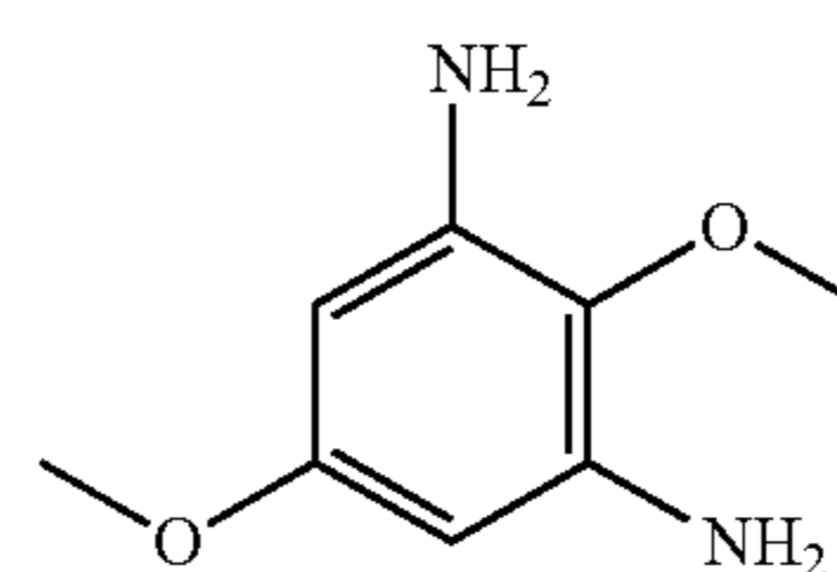
2,5-dimethoxybenzene-1,3-diamine
