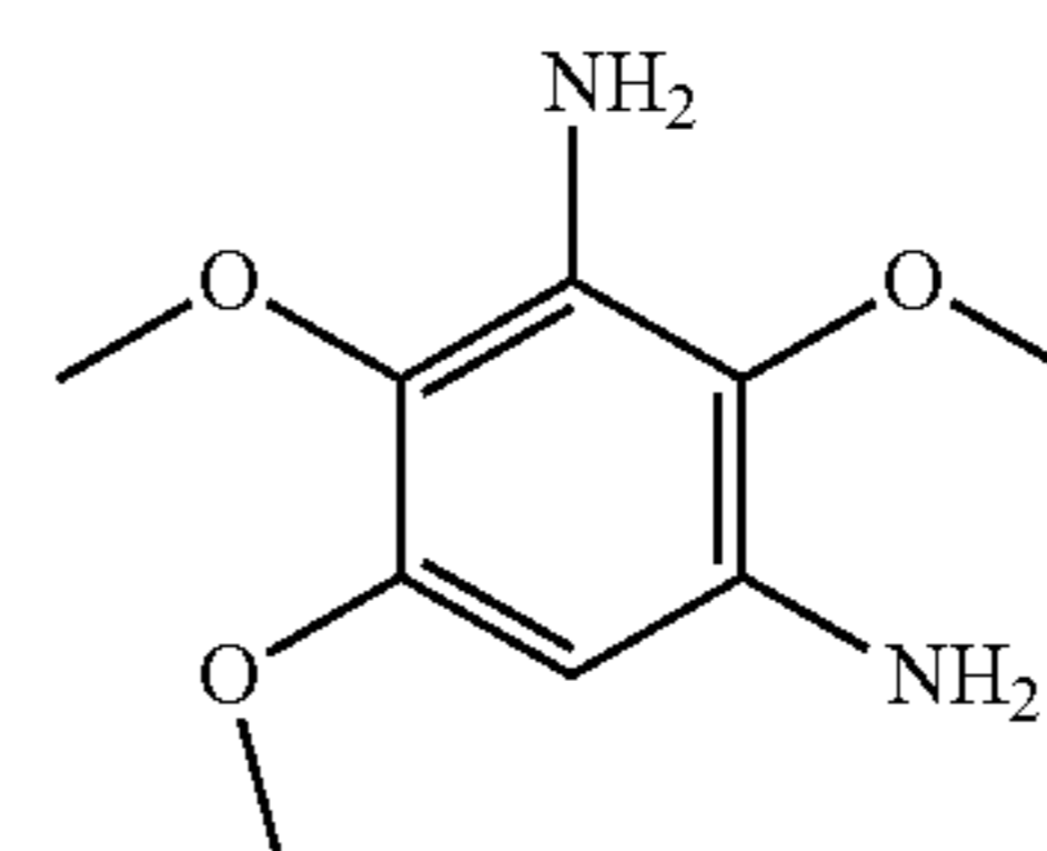
2,4,5-trimethoxybenzene-1,3-diamine
