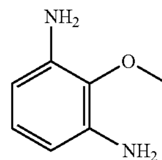
2-methoxybenzene-1,3-diamine
