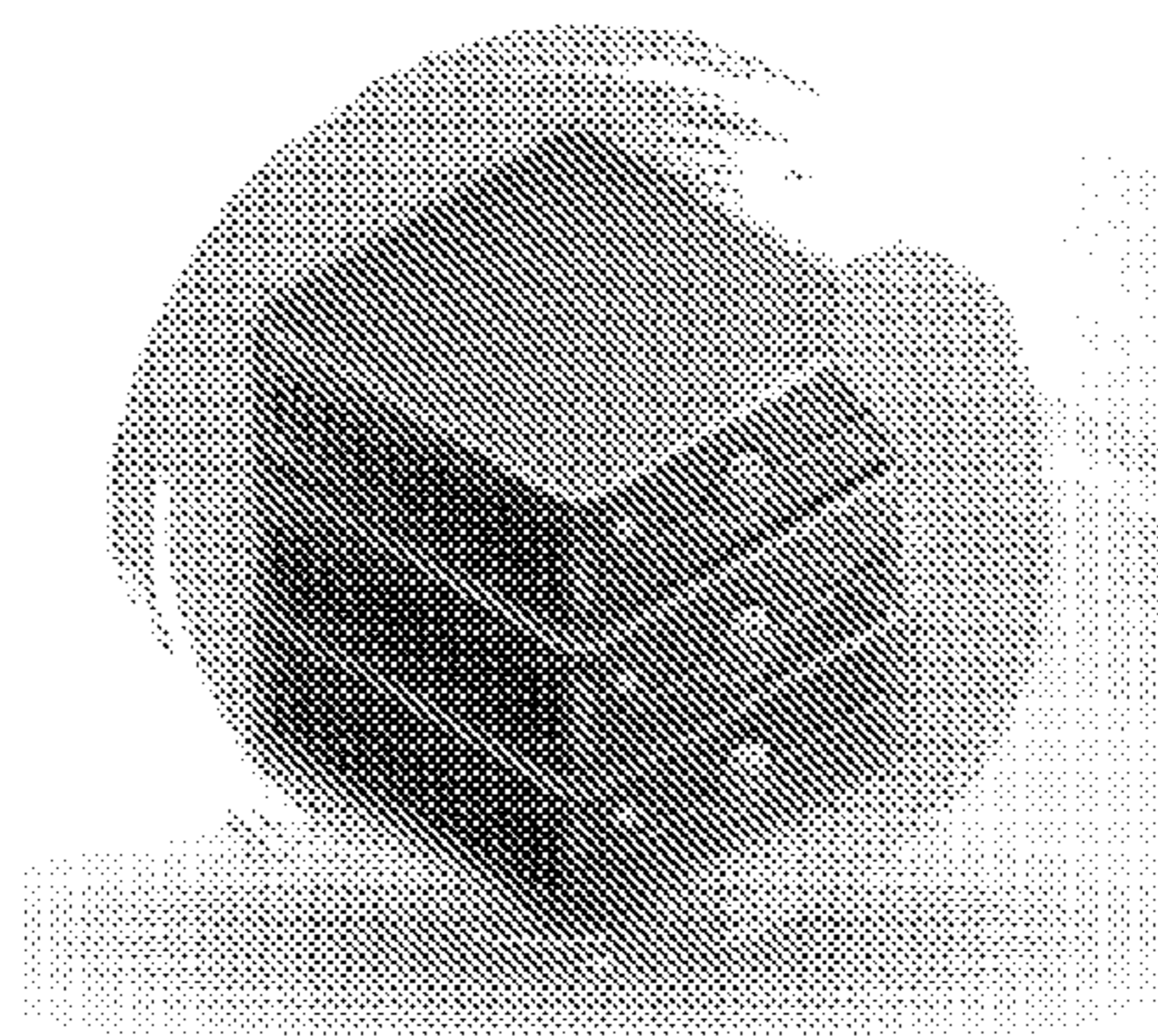
update Server •710
