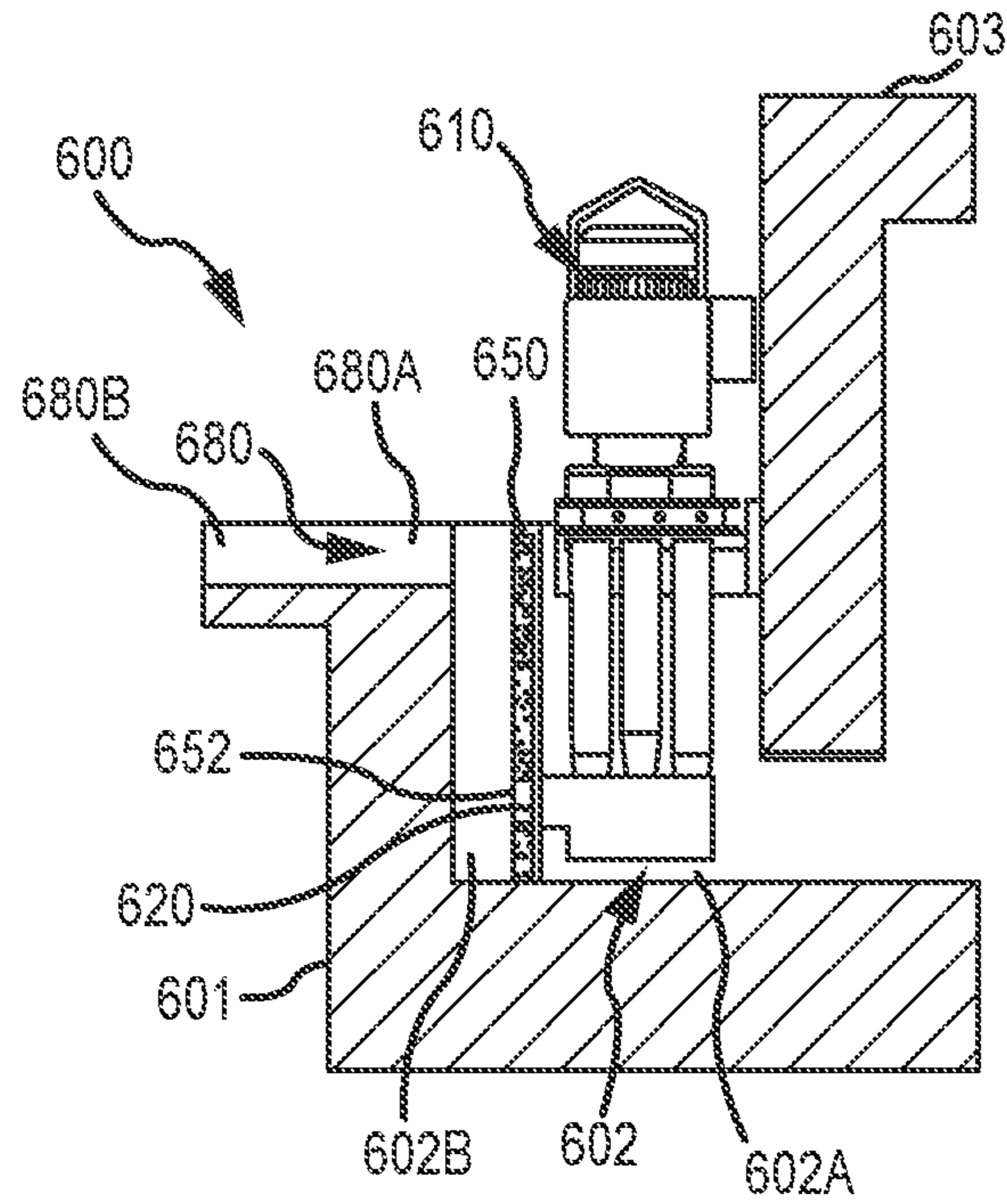
SECTION A-A
