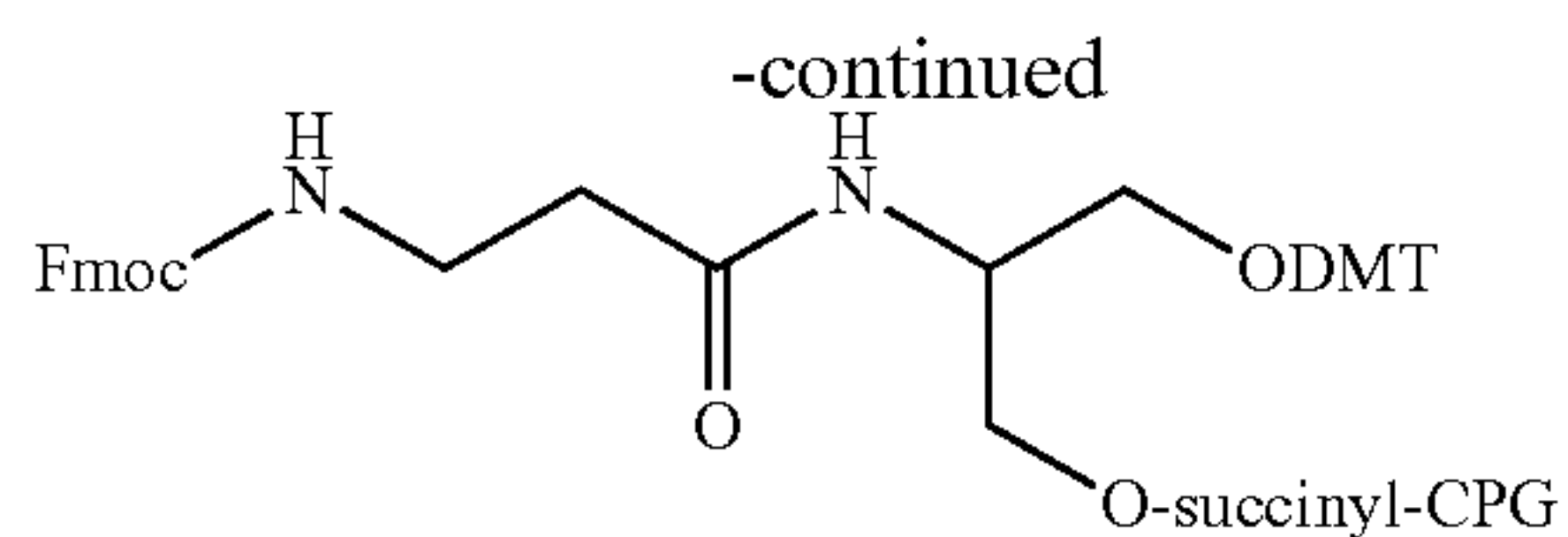
3'-Amino-Modifier Serinol CPG
