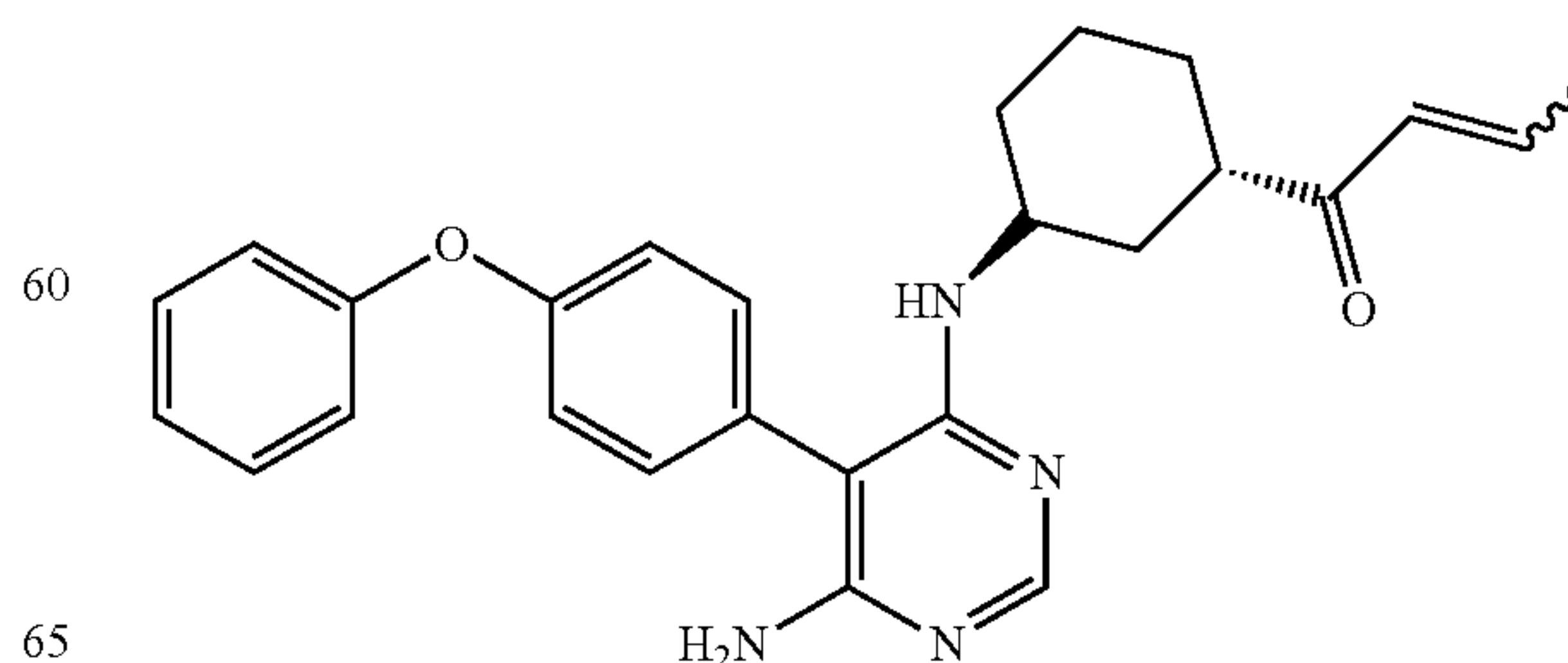
1-3-((6-Amino-5-(4-phenoxyphenyl)-pyrimidin-4-ylamino)-methyl)-phenyl)-but-2-yn-1-one (A141)
