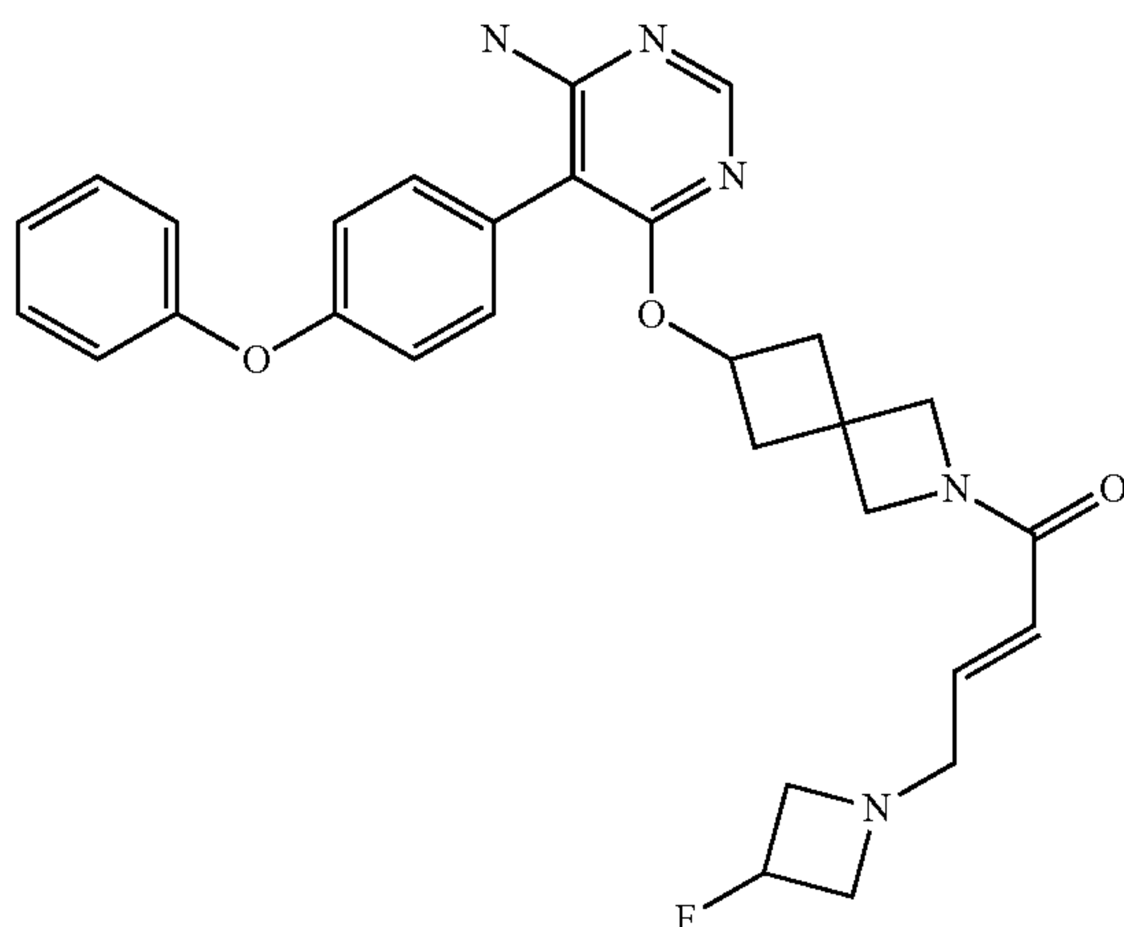
(E)-1-(6-((6-amino-5-(4-phenoxyphenyl)pyrimidin-4-yl)oxy)-2-azaspiro[3.3]heptan-2-yl)-4-(3-fluoroazetidin-1-yl)but-2-en-1-one (A222)
