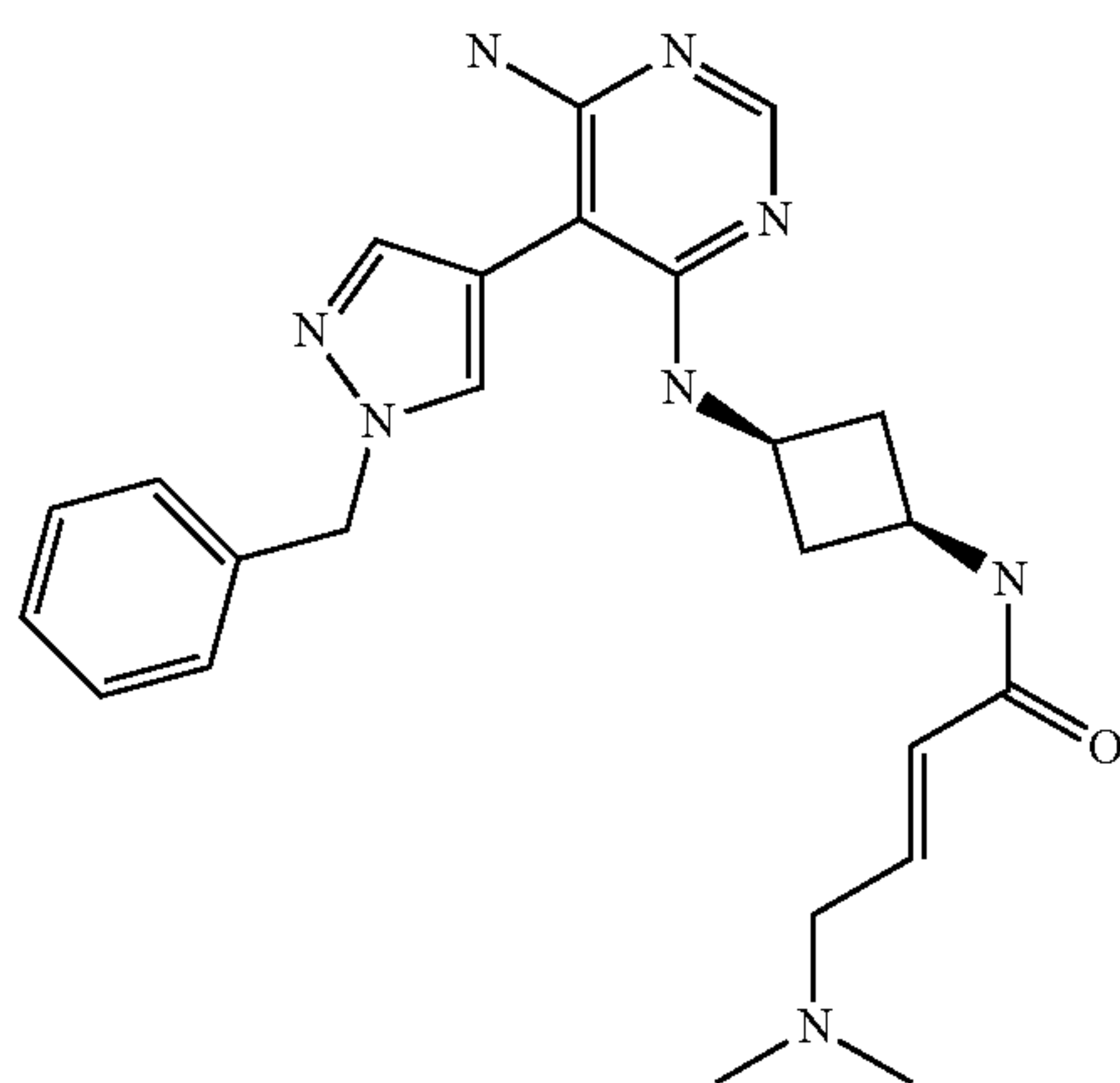
(E)-N-(1,3-cis-3-((6-amino-5-(1-benzyl-1H-pyrazol-4-yl)pyrimidin-4-yl)amino)cyclobutyl)-4-(dimethylamino)but-2-enamide (A230)
