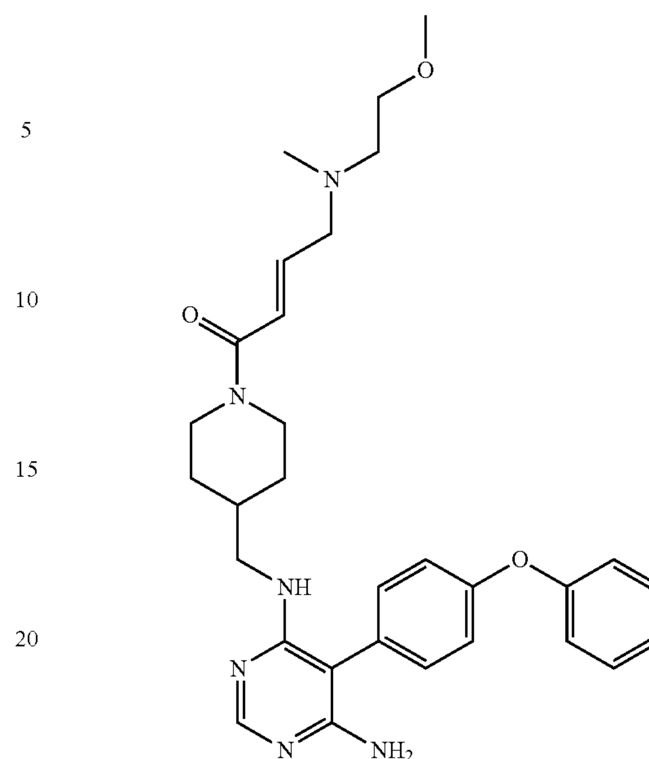
(E)-1-(4-(((6-amino-5-(4-phenoxyphenyl)pyrimidin-4-yl)amino)methyl)piperidin-1-yl)-4-((2-methoxyethyl)(methyl)amino)but-2-en-1-one (A11)
