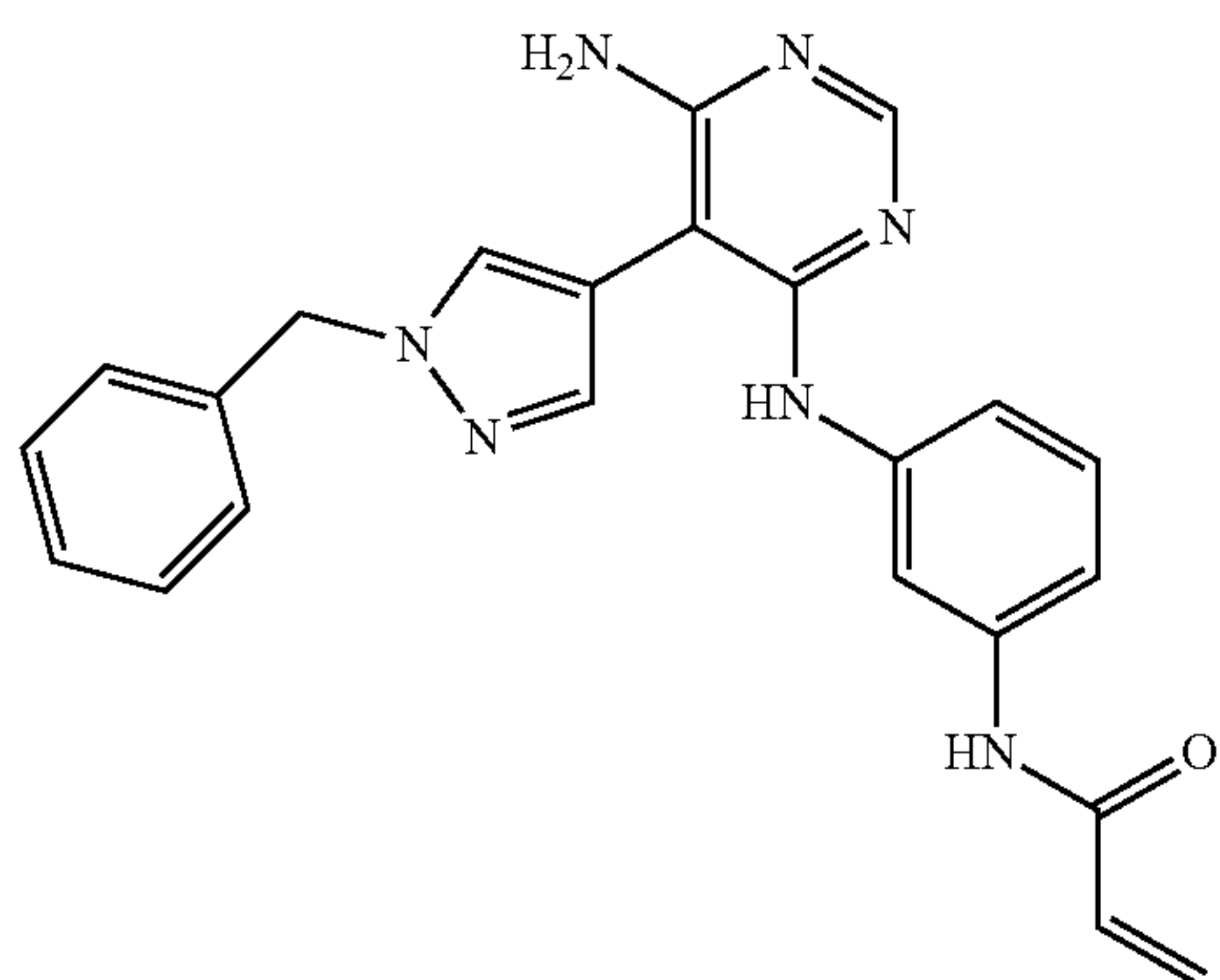
N-(3-((6-amino-5-(1-benzyl-1H-pyrazol-4-yl)pyrimidin-4-yl)amino)phenyl)acrylamide (A70)
