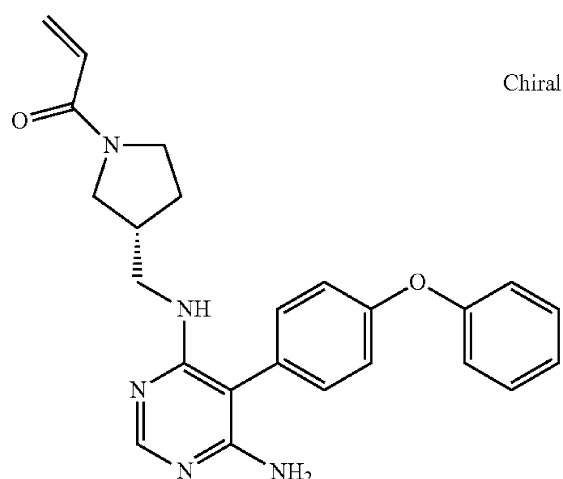
(R)-1-(3-(((6-amino-5-(4-phenoxyphenyl)pyrimidin-4-yl)amino)methyl)pyrrolidin-1-yl)prop-2-en-1-one (A4)
