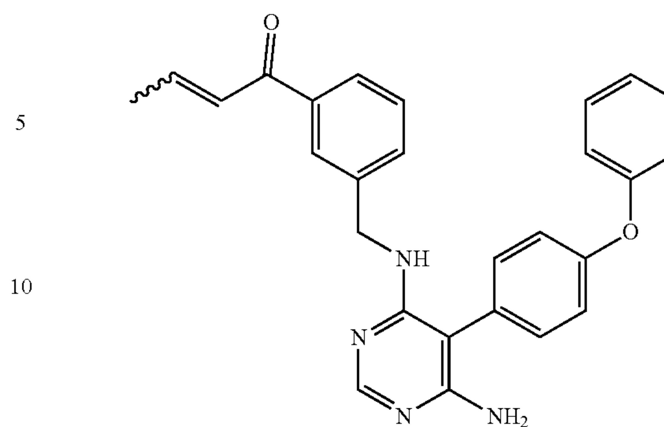
1-3-((6-Amino-5-(4-phenoxyphenyl)-pyrimidin-4-ylamino)-methyl)-phenyl)-but-2-en-1-one (A142)
