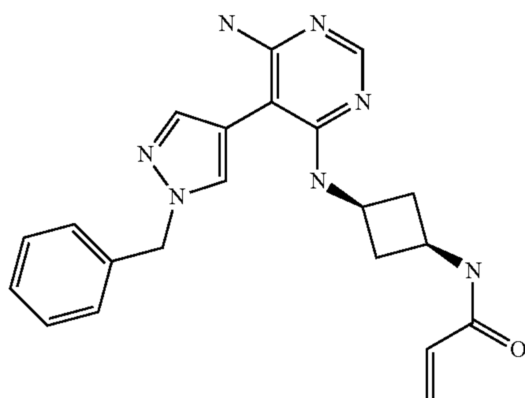
N-(1,3-cis-3-((6-amino-5-(1-benzyl-1H-pyrazol-4-yl)pyrimidin-4-yl)amino)cyclobutyl)acrylamide (A229)
