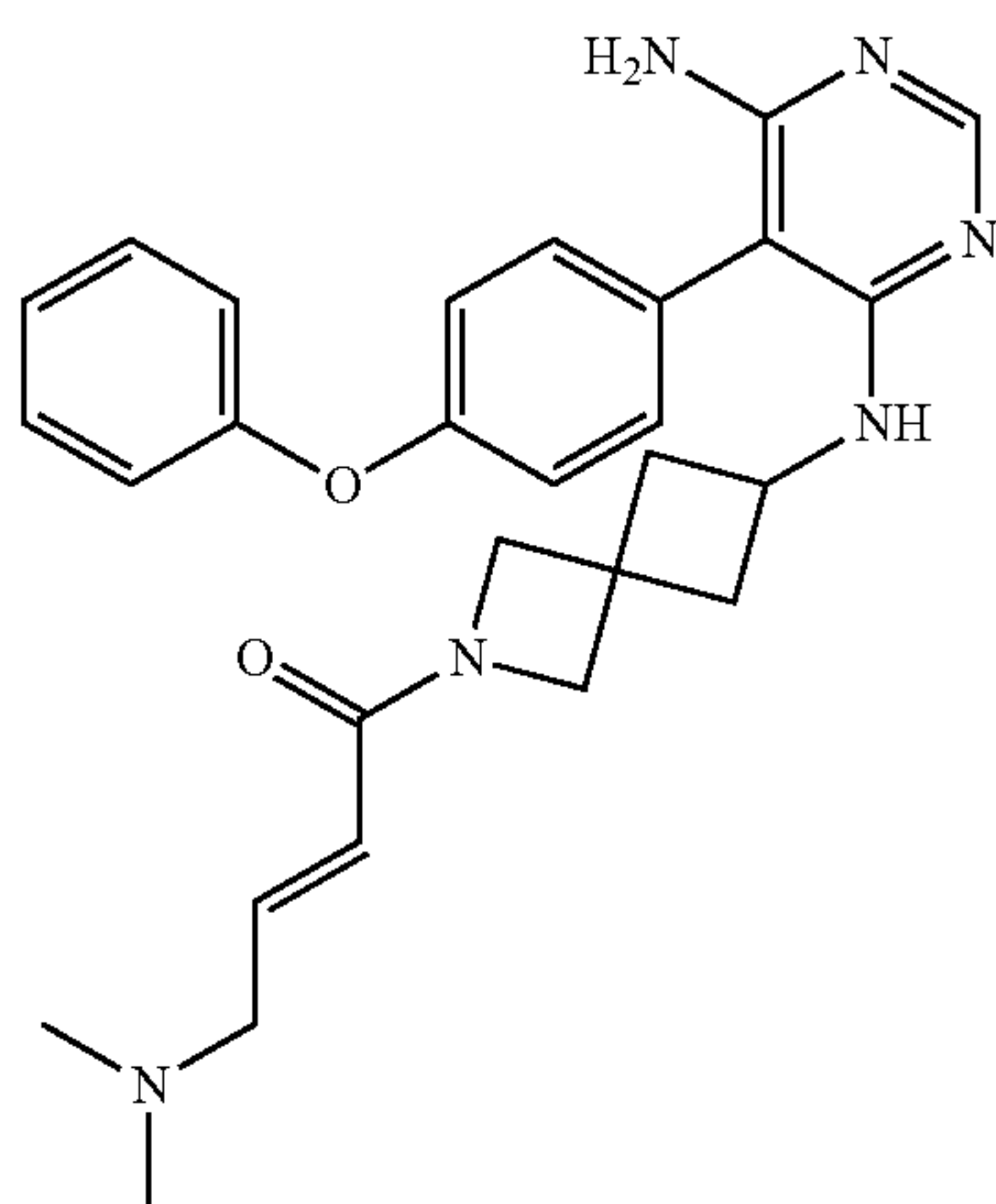
(E)-1-(6-((6-amino-5-(4-phenoxyphenyl)pyrimidin-4-yl)amino)-2-azaspiro[3.3]heptan-2-yl)-4-(dimethylamino)but-2-en-1-one (A127)
