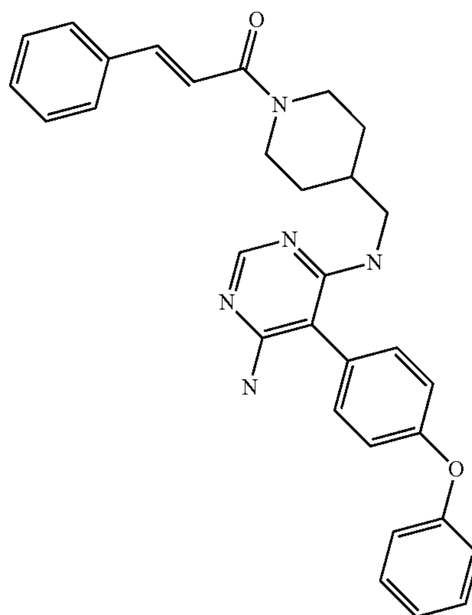
(E)-1-(4-(((6-amino-5-(4-phenoxyphenyl)pyrimidin-4-yl)amino)methyl)piperidin-1-yl)-3-phenylprop-2-en-1-one (A231)
