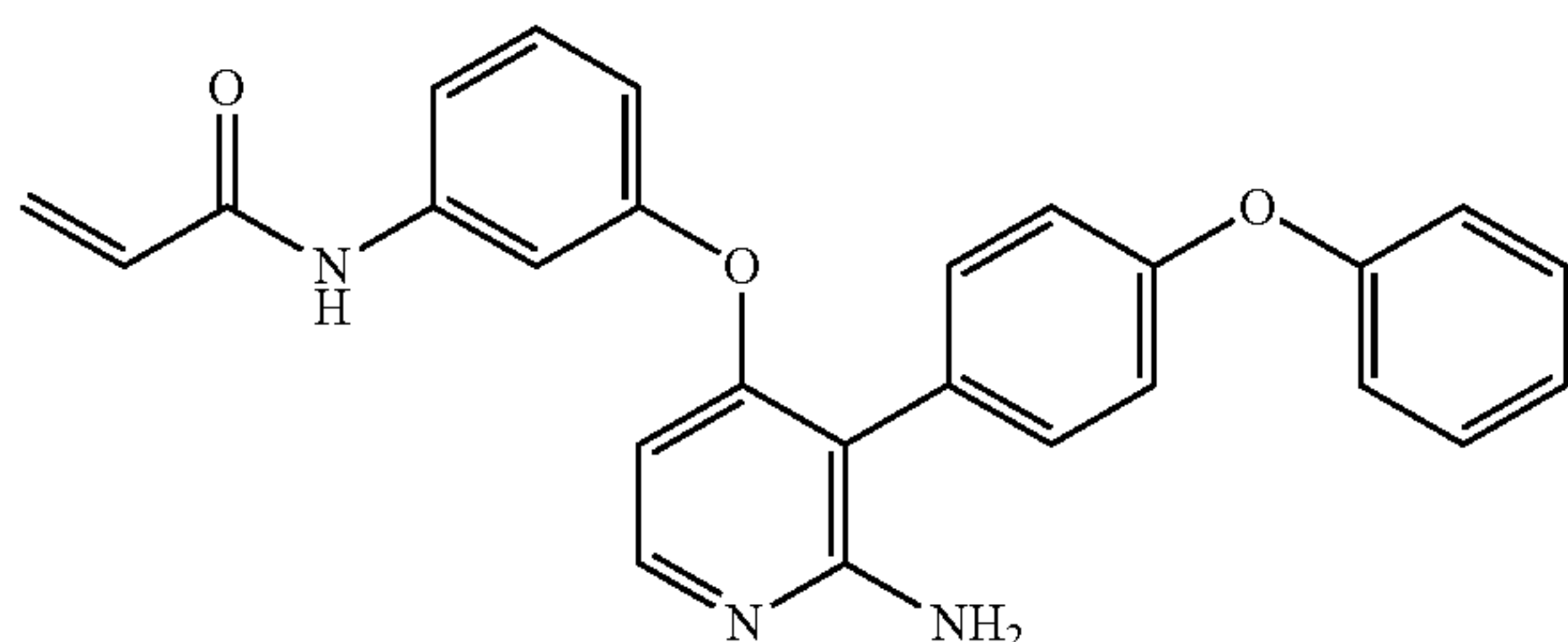
N-(3-((2-amino-3-(4-phenoxyphenyl)pyridin-4-yl)oxy)phenyl)acrylamide (A244)
