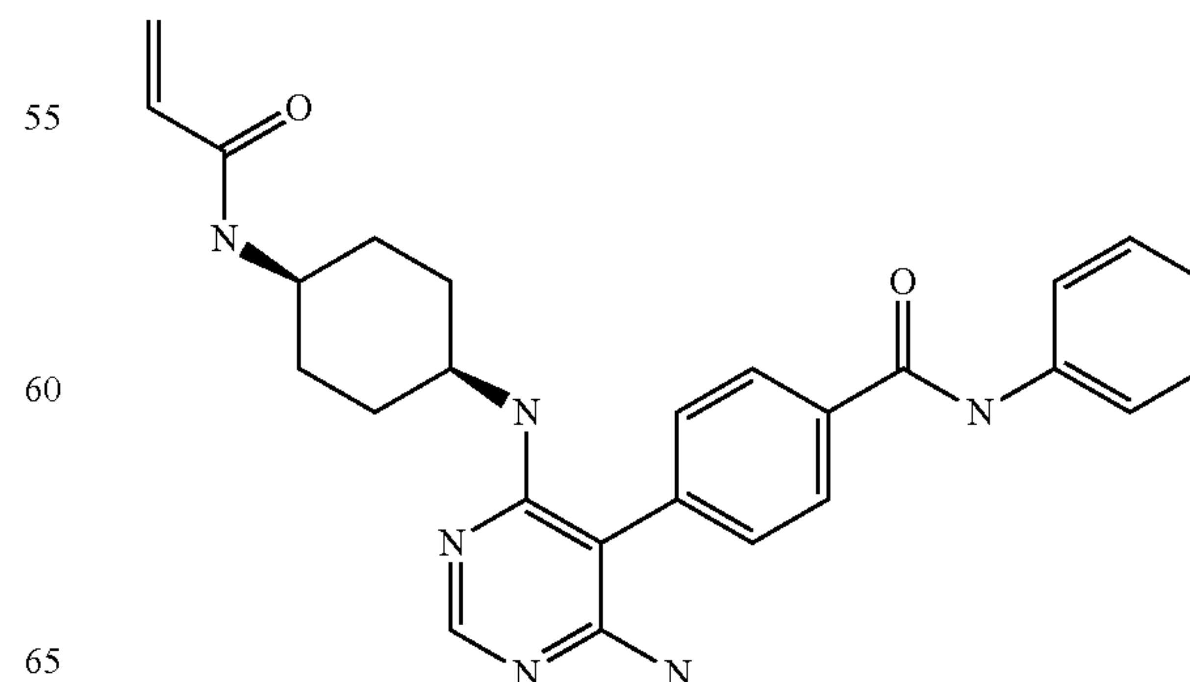
1-(3-(((6-amino-5-(4-(benzyloxy)phenyl)pyrimidin-4-yl)amino)methyl)pyrrolidin-1-yl)prop-2-en-1-one (A156)
