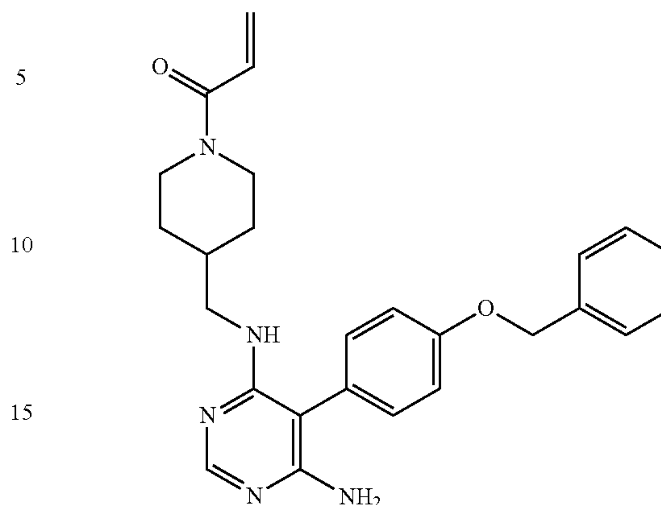
1-(4-(((6-amino-5-(4-(benzyloxy)phenyl)pyrimidin-4-yl)amino)methyl)piperidin-1-yl)prop-2-en-1-one (A292)
