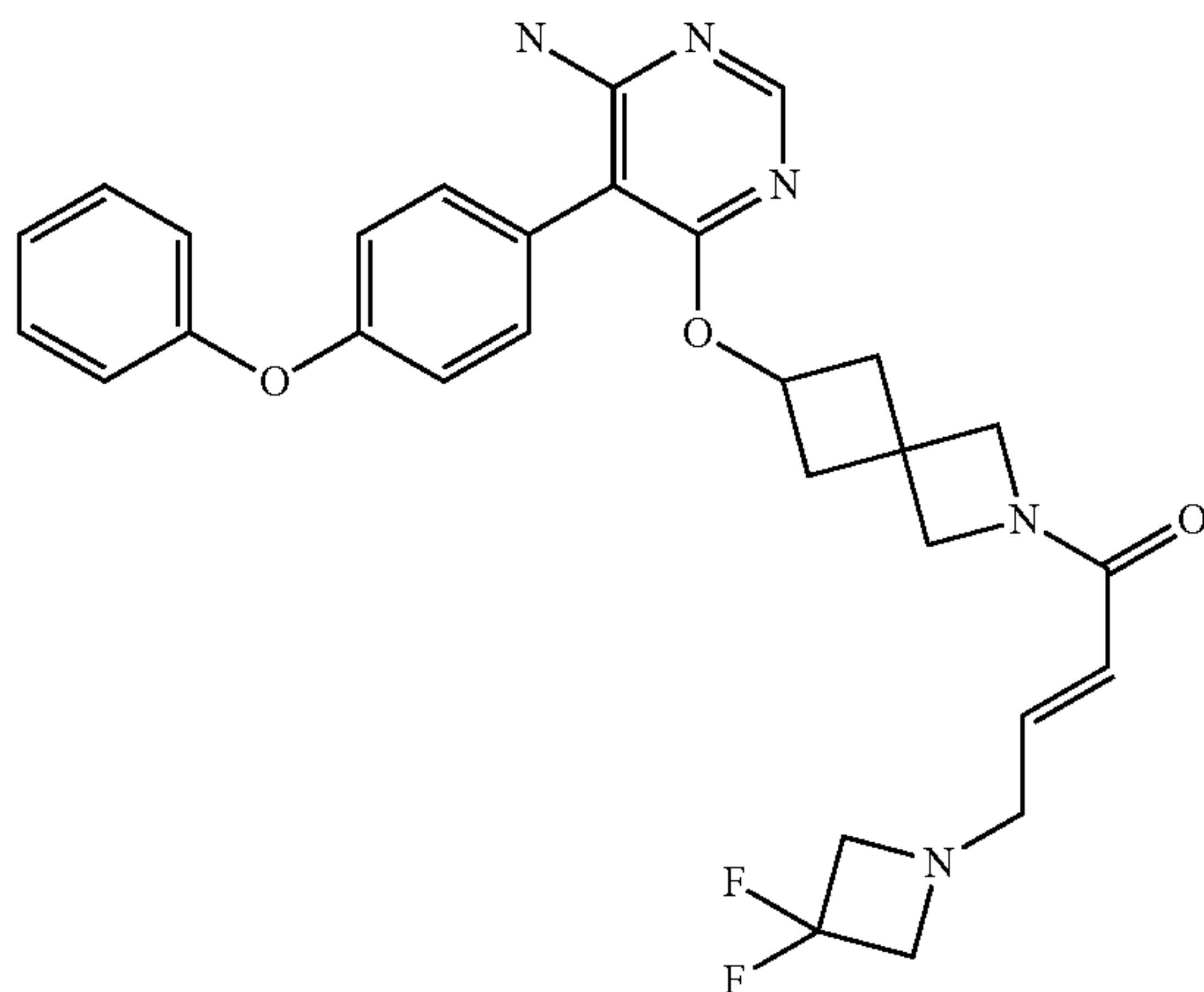
(E)-1-(6-((6-amino-5-(4-phenoxyphenyl)pyrimidin-4-yl)oxy)-2-azaspiro[3.3]heptan-2-yl)-4-(3,3-difluoroazetidin-1-yl)but-2-en-1-one (A223)
