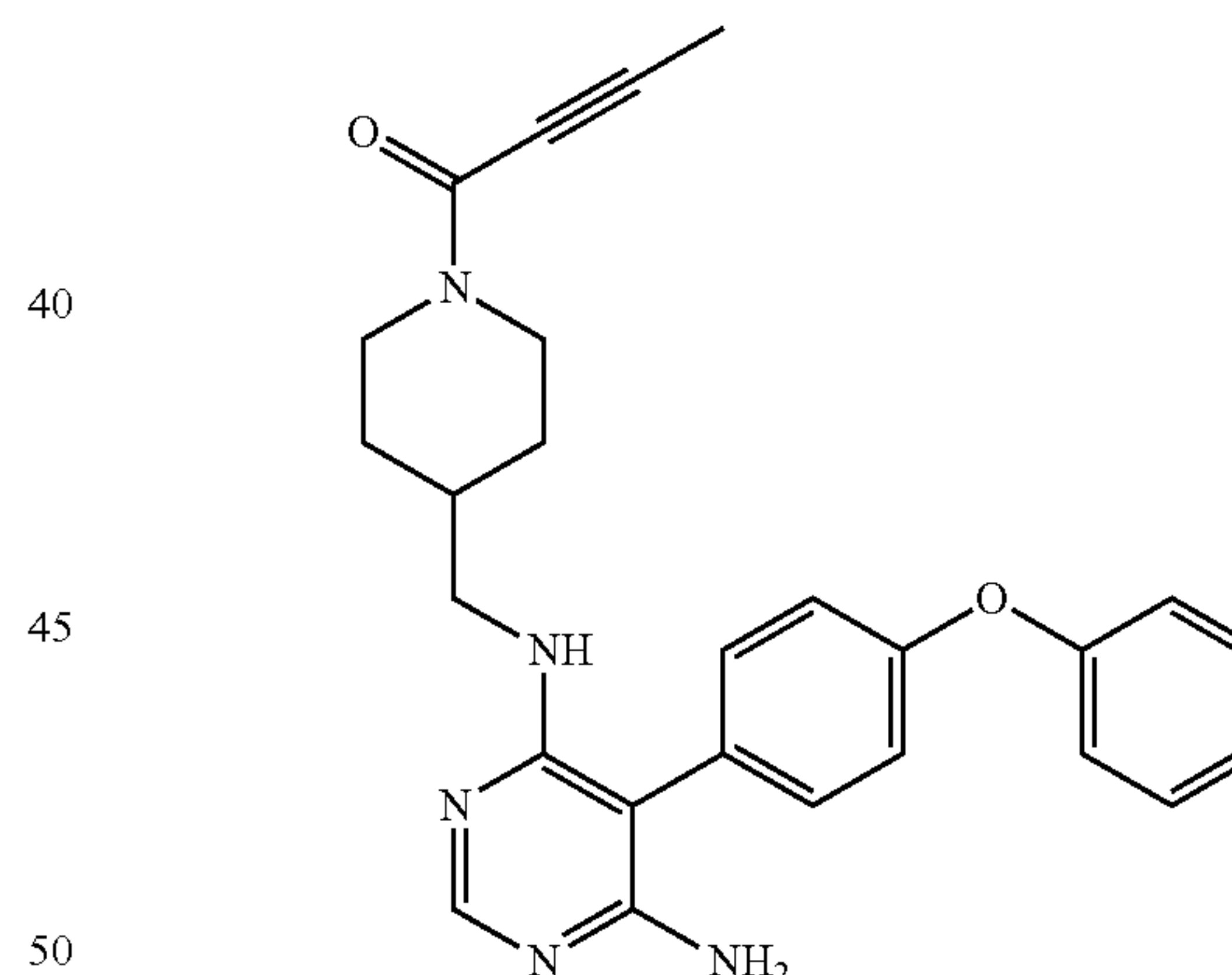
1-(4-(((6-amino-5-(4-phenoxyphenyl)pyrimidin-4-yl)amino)methyl)piperidin-1-yl)but-2-yn-1-one (A336)
