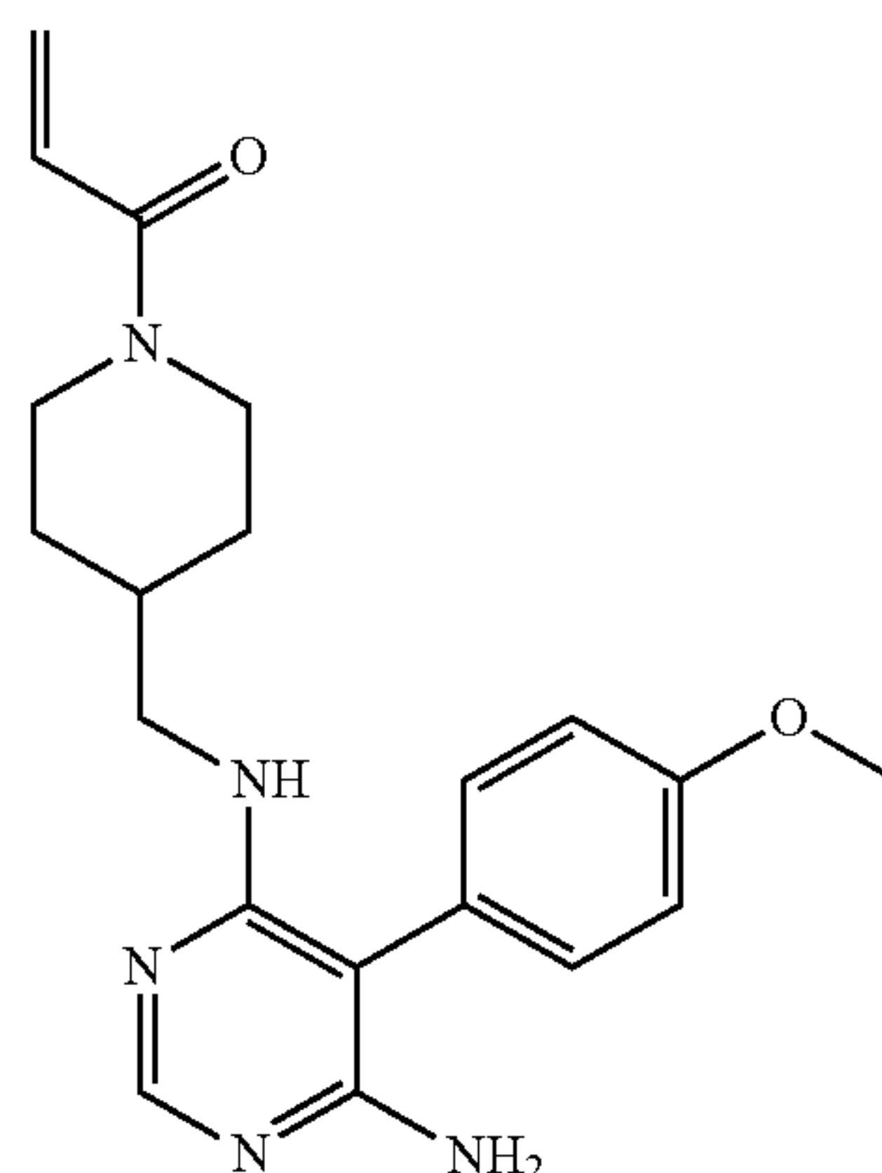
1-(4-(((6-amino-5-(4-methoxyphenyl)pyrimidin-4-yl)amino)methyl)piperidin-1-yl)prop-2-en-1-one (A85)
