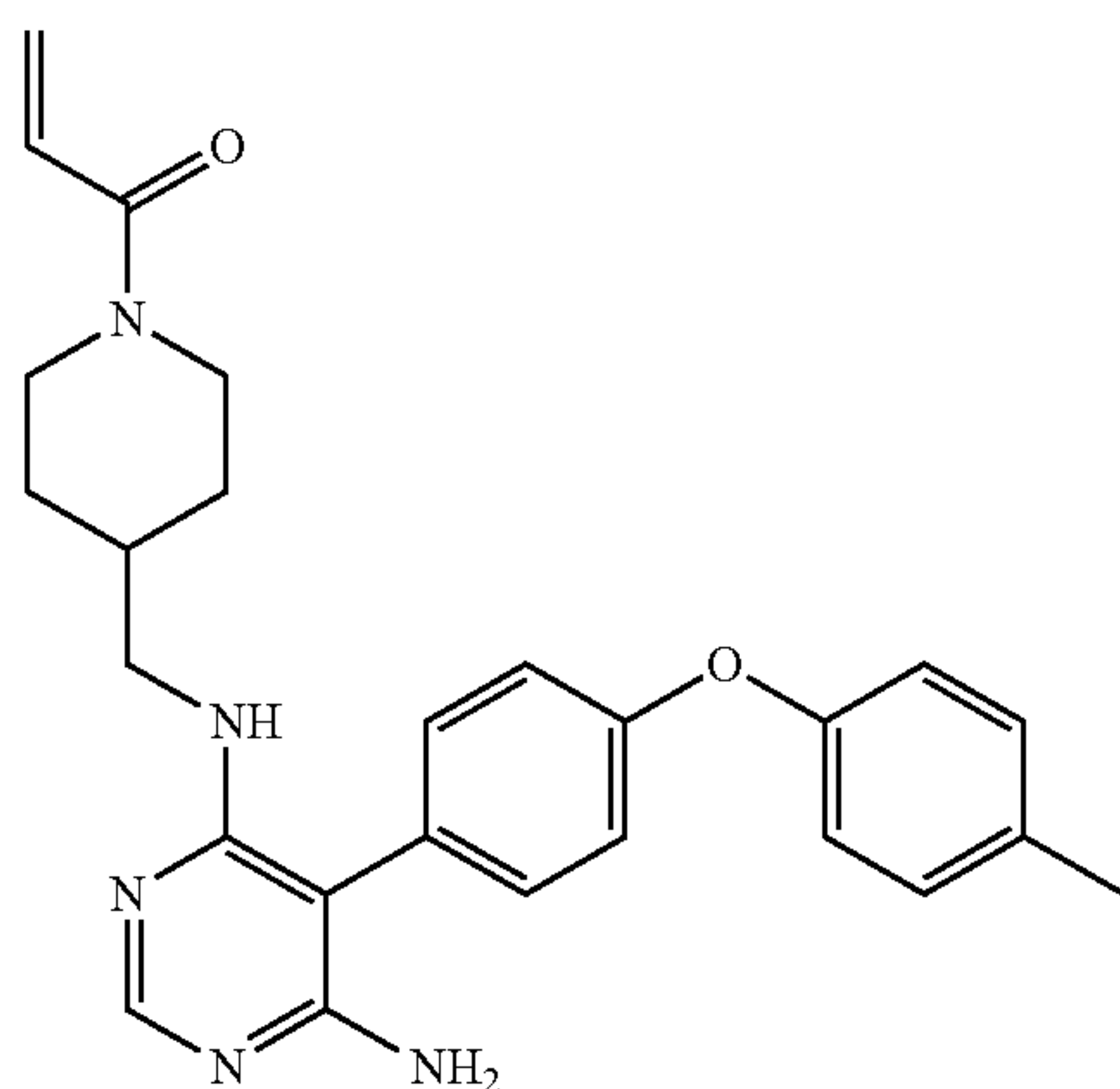
1-(4-(((6-amino-5-(4-(p-tolyloxy)phenyl)pyrimidin-4-yl)amino)methyl))piperidin-1-yl)prop-2-en-1-one (A98)
