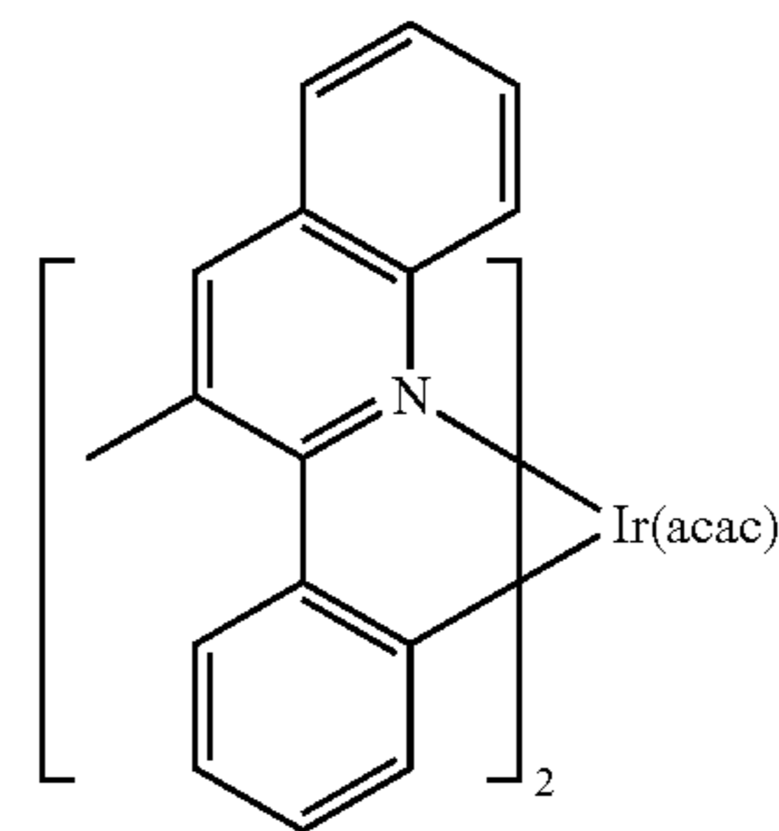
Ir(3-Mepq) 2 (acac)
