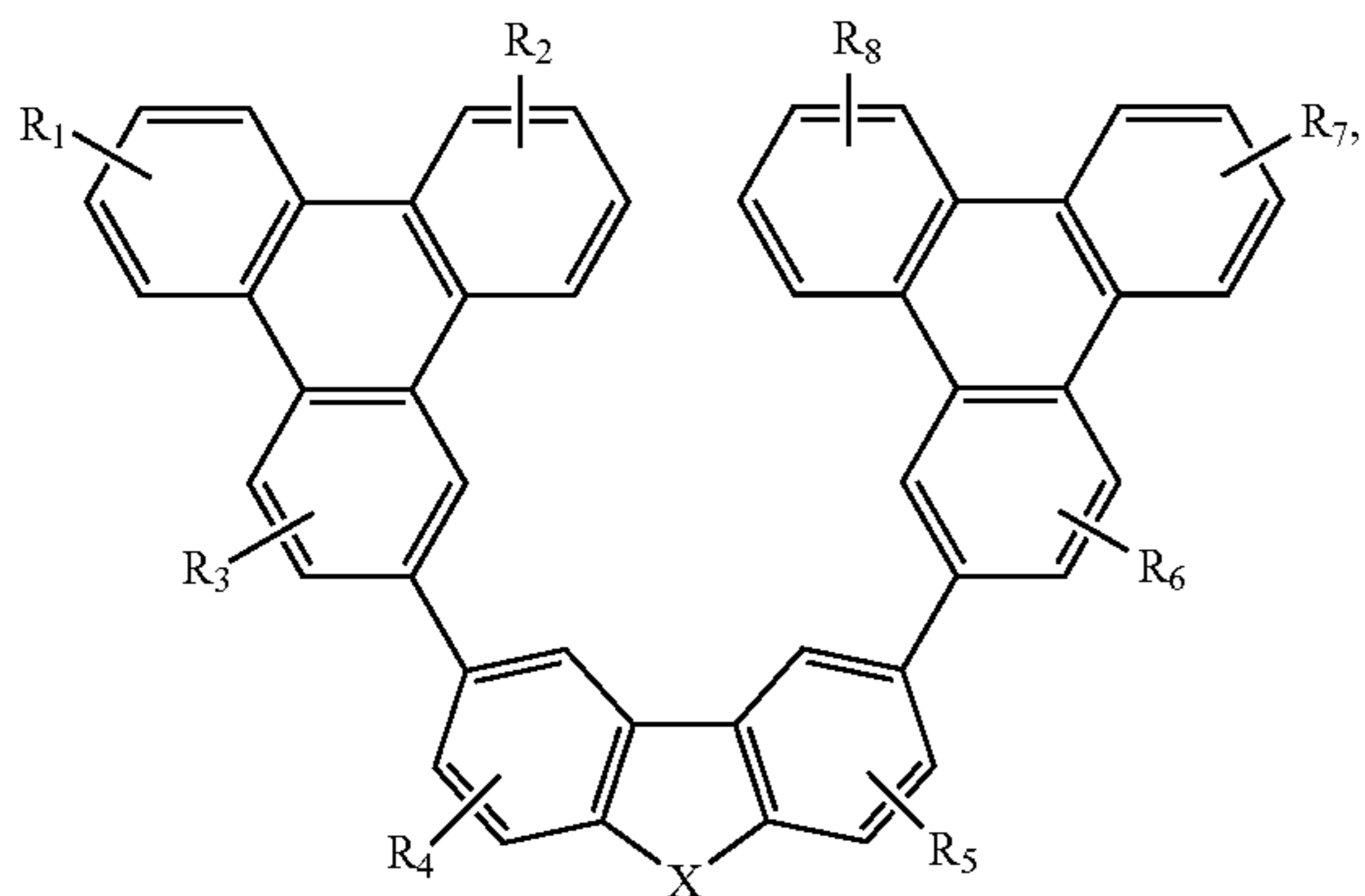
Compound 6G
