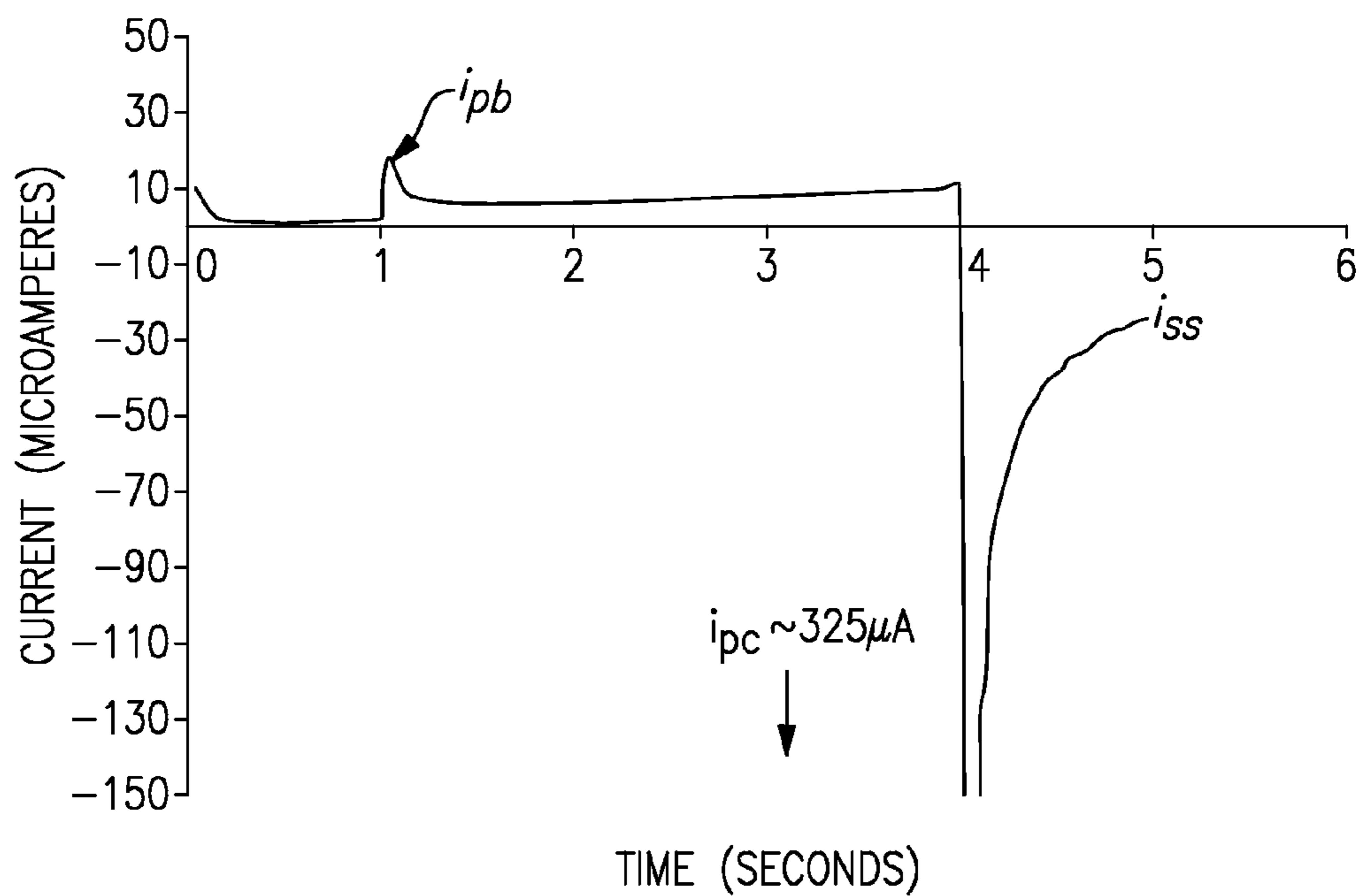
FIG.8B
