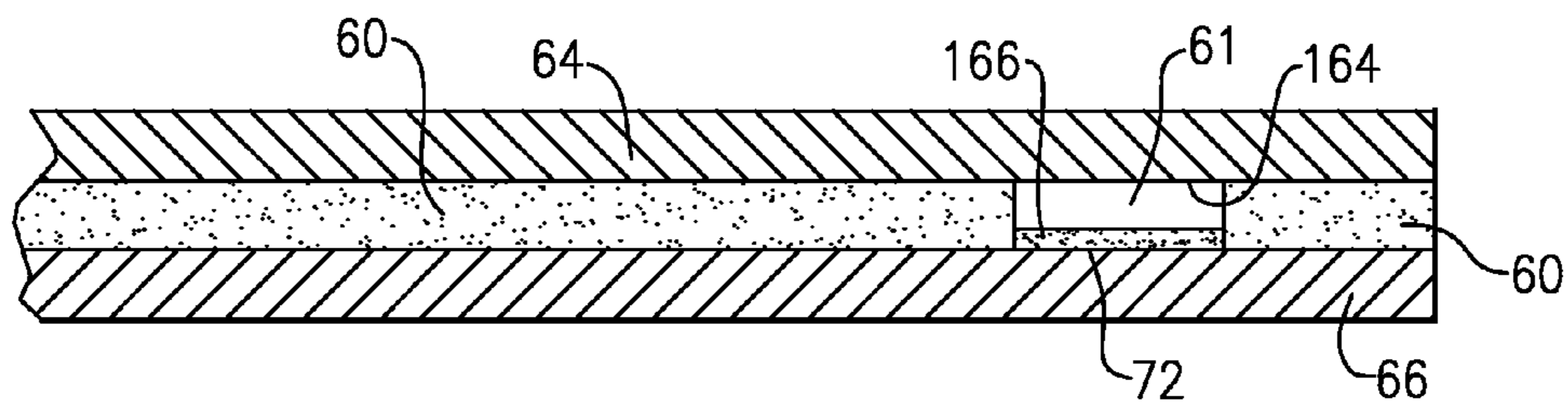
FIG. 4B
