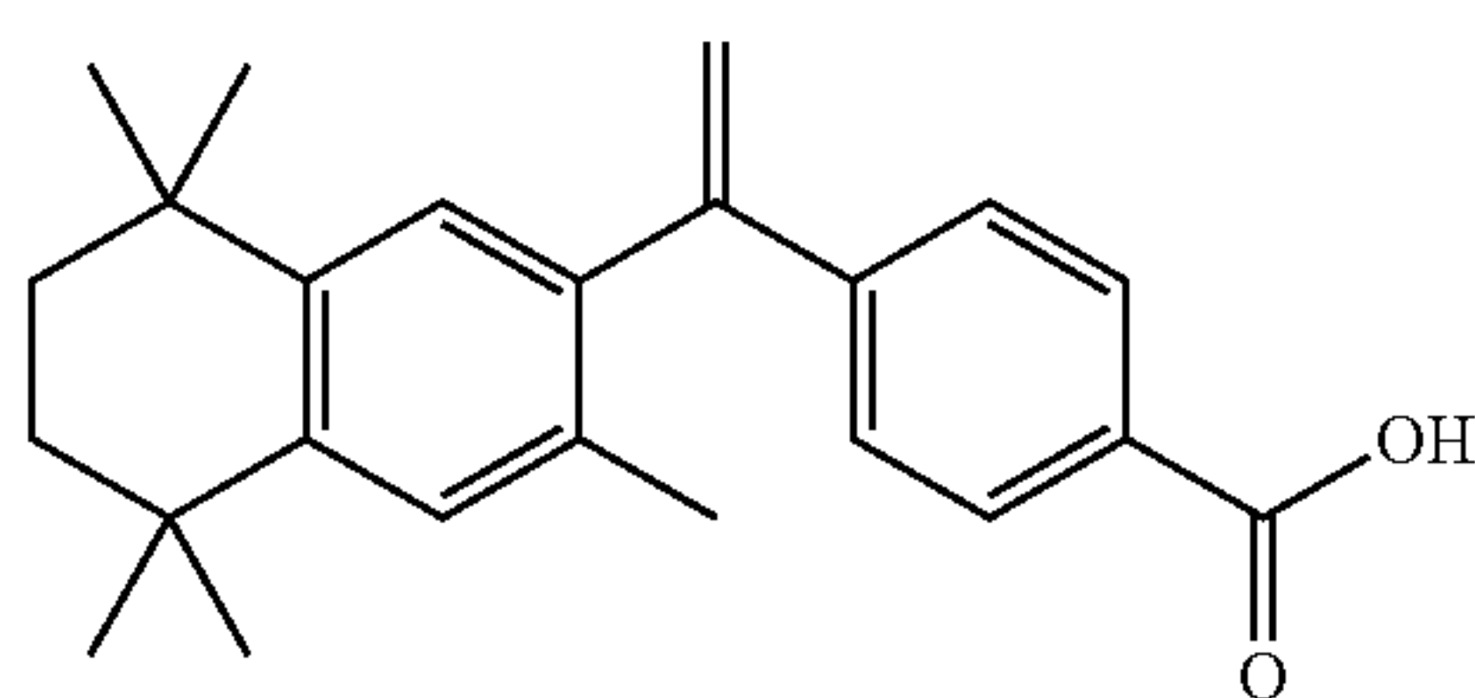
Bexarotene
